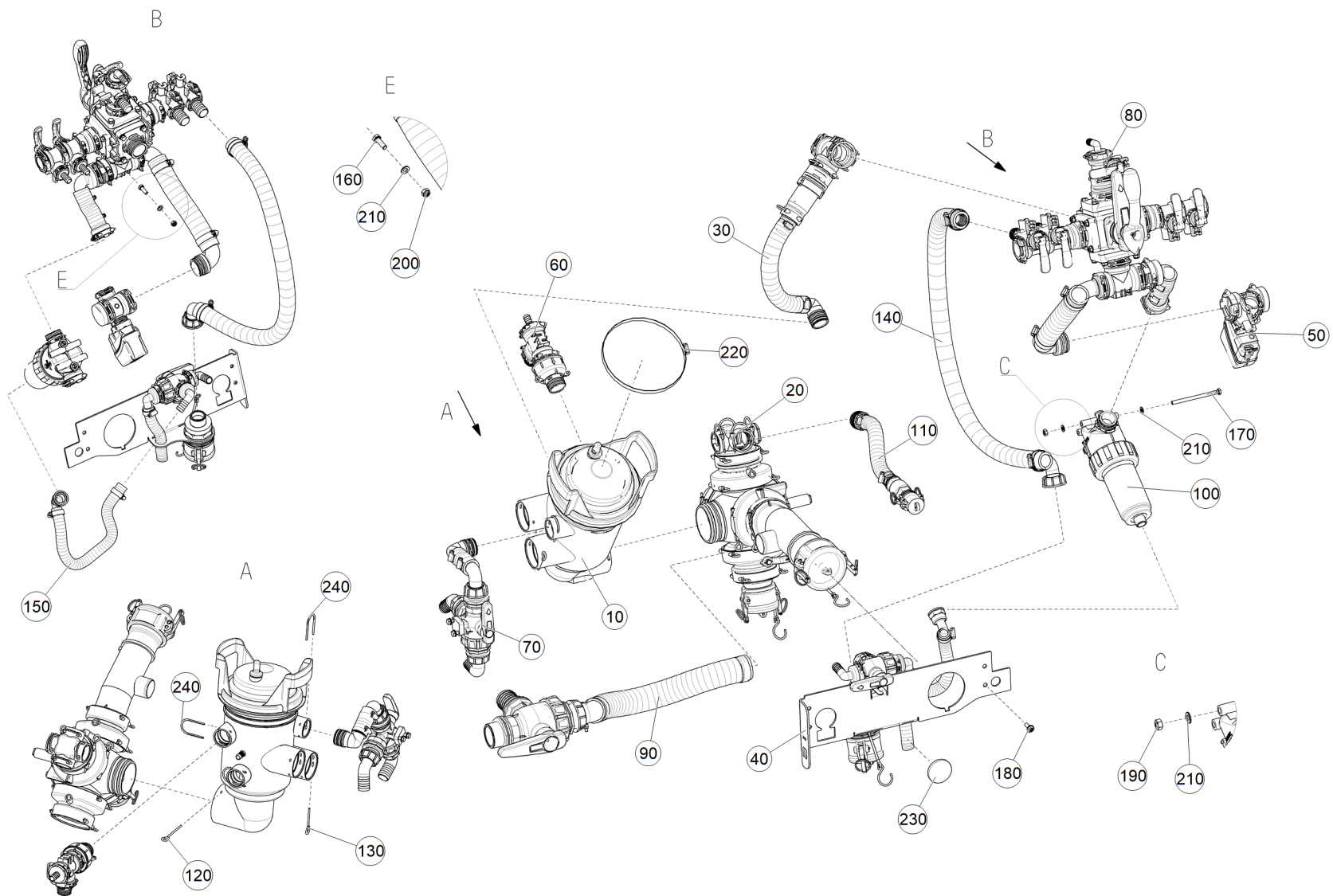
Рис. 1 ЕТВ-6000000268 (Аматюра)
