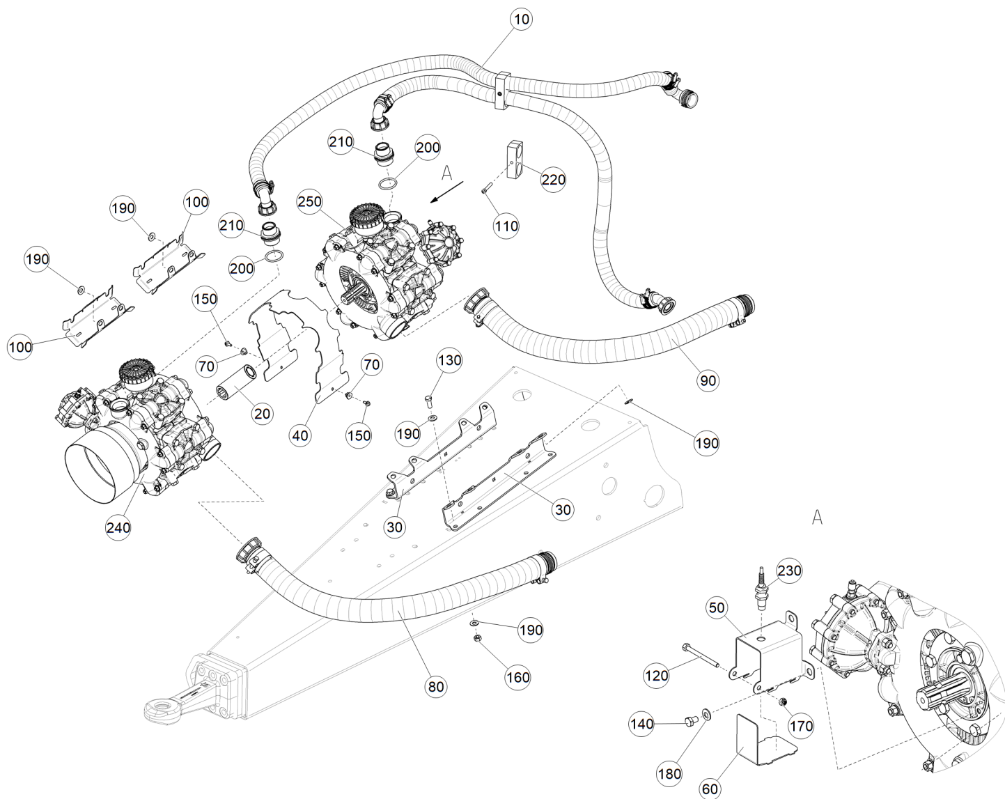
Рис. 1 ЕТВ-6000000259 (Крепление и подключение поршневых насосов)
