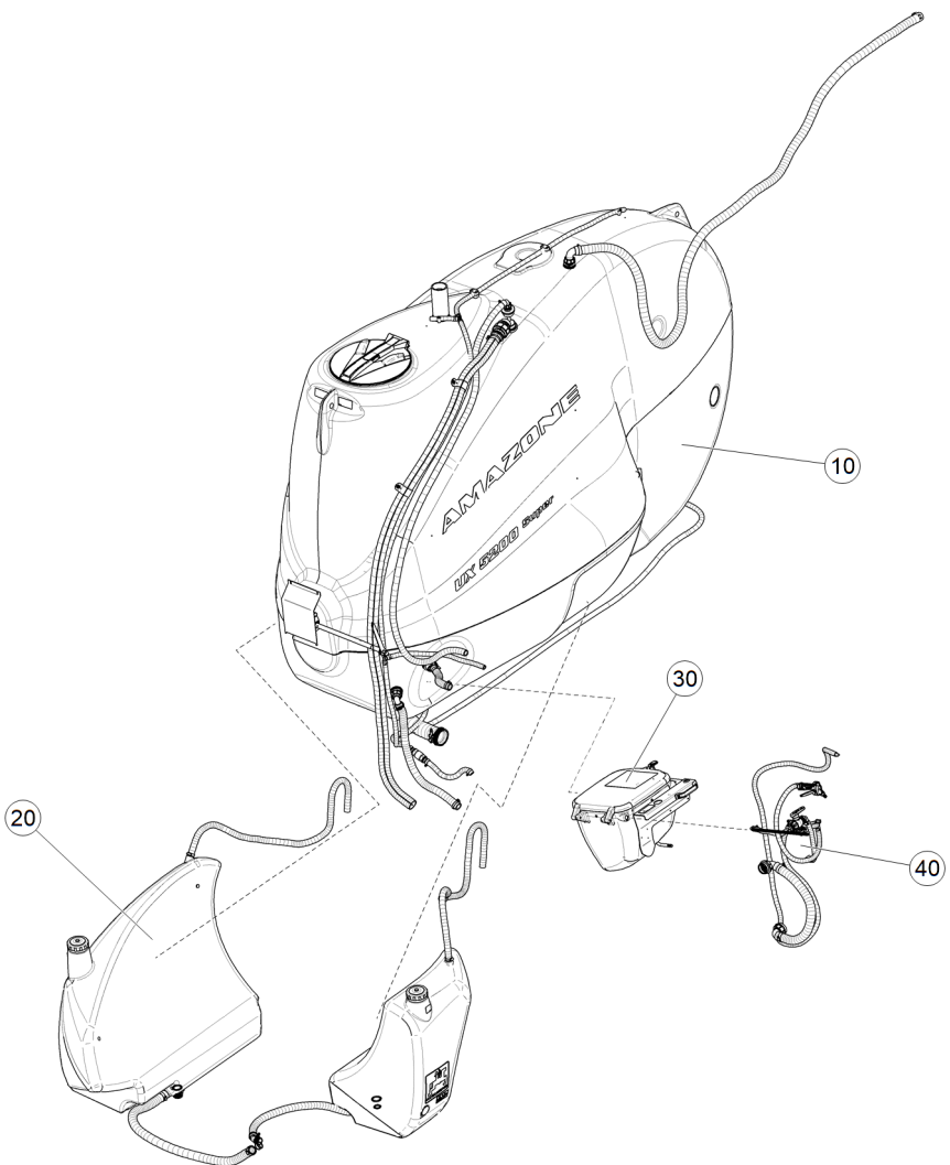
Рис. 1 ЕТВ-6000000270 (Емкости)
