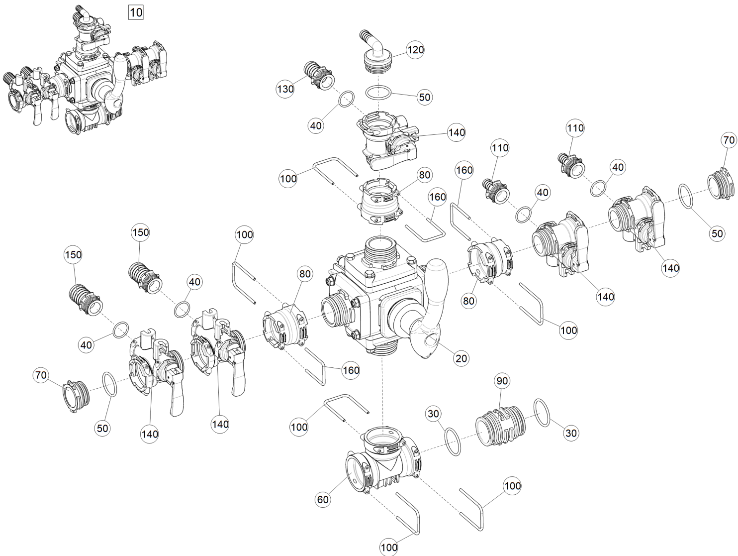
Рис. 1 ETV-6000000311 (Блок управления КН 1 1/4 ZOLL SPEZIAL)
