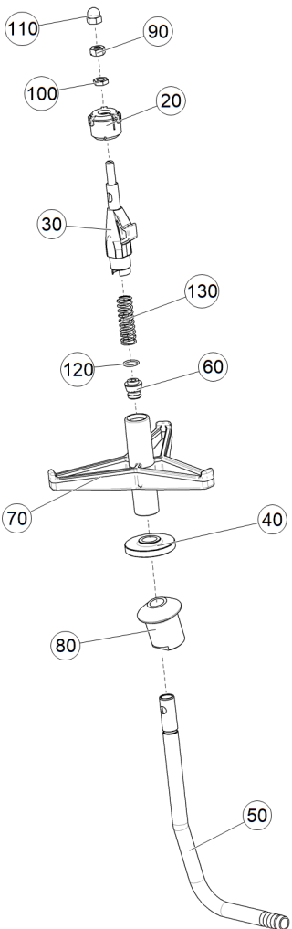
Рис. 1 ЕТВ-60000000343 (Очиститель канистр)
