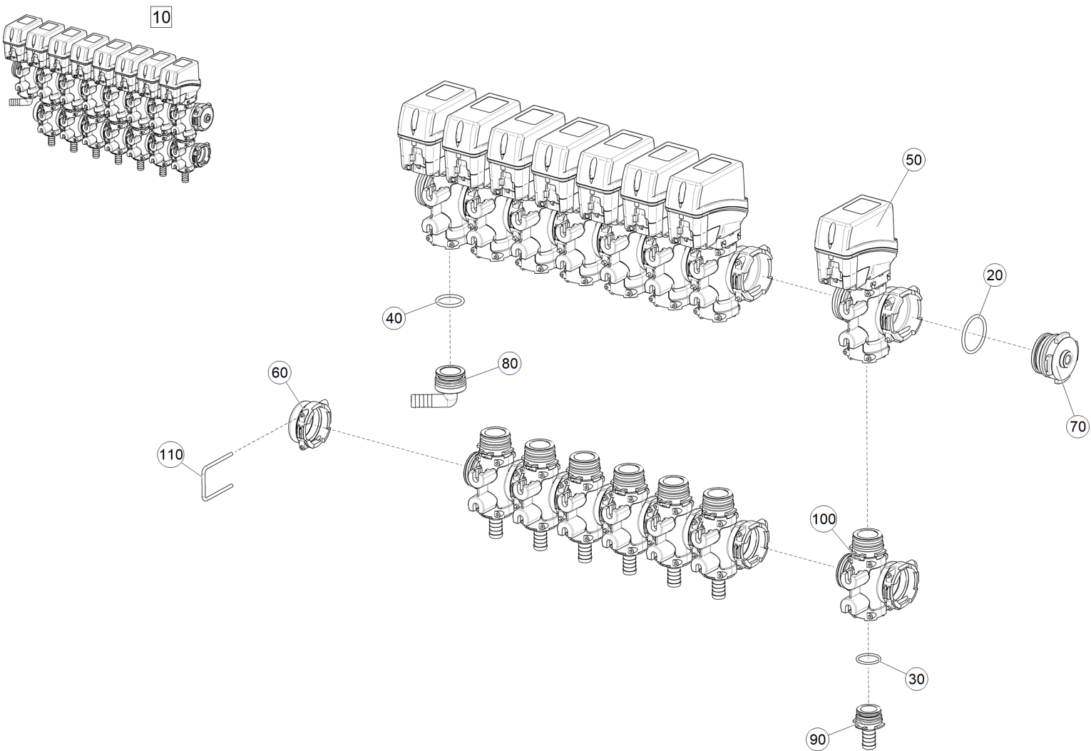
Рис. 1 ЕТВ-6000000346 (Блок модульный 7Т)
