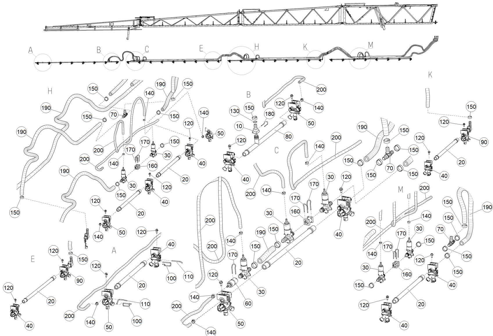
Рис. 1 ЕТВ-6000000291 (Штанга)
