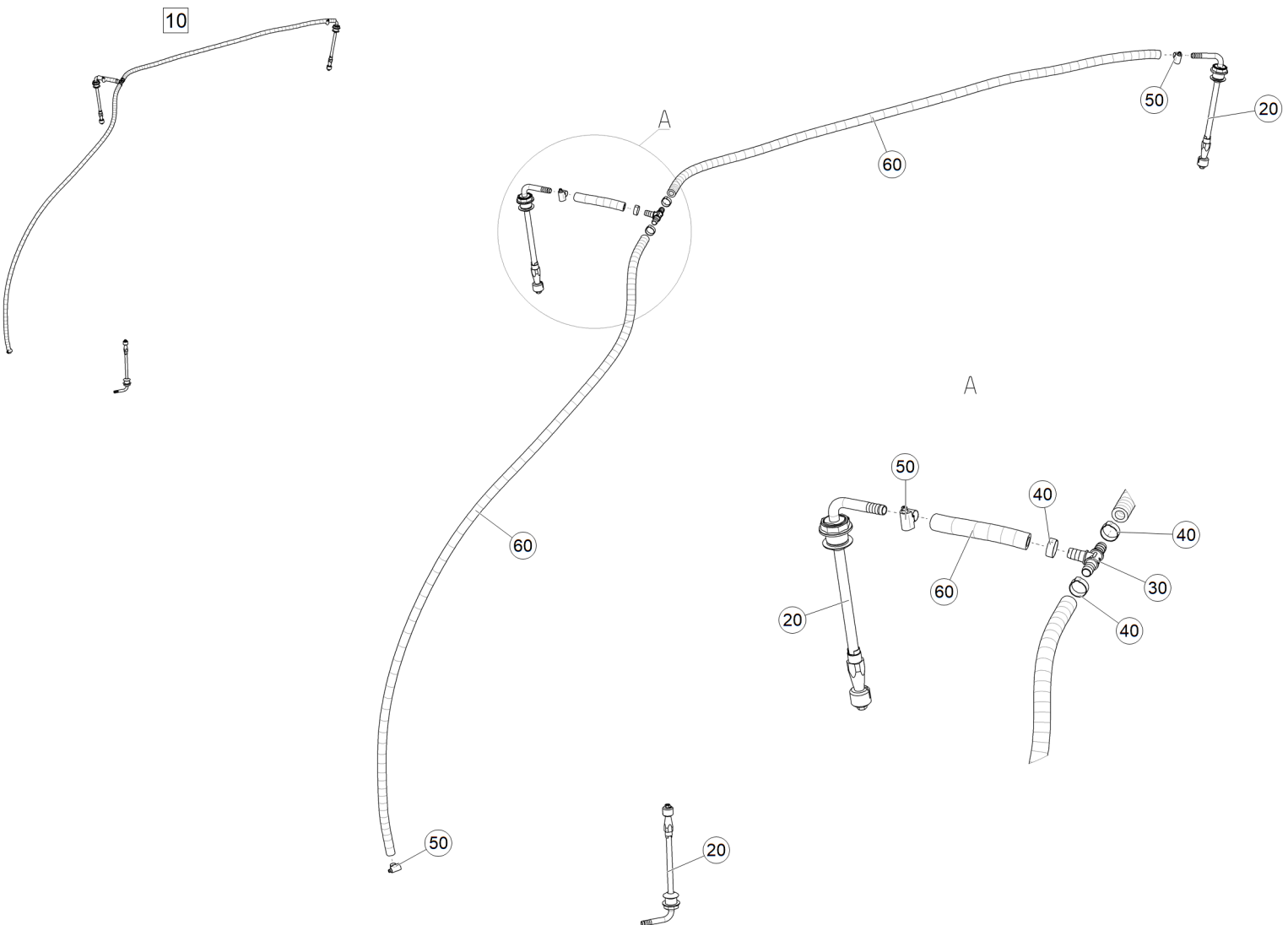
Рис. 1 ЕТВ-60000000328 (Очищение бункера)
