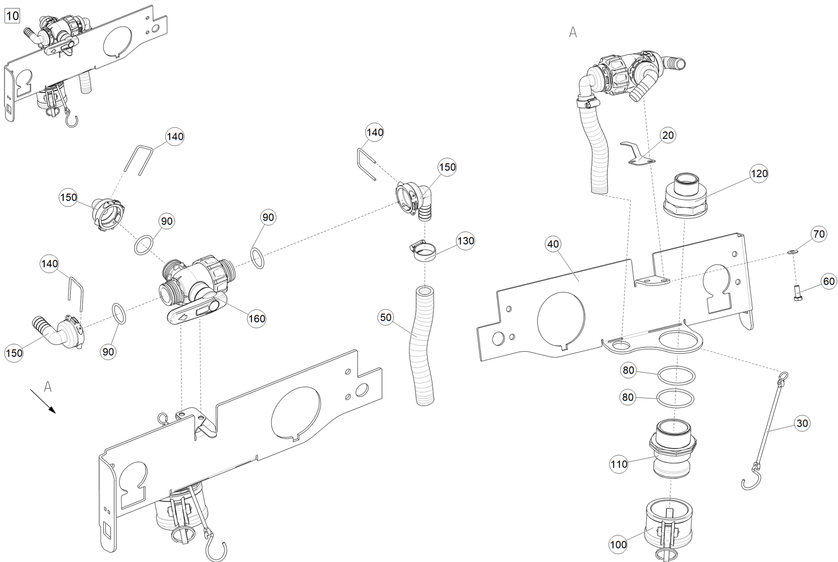
Рис. 1 ETB-6000000302 (Панель передняя 3" VORM.)
