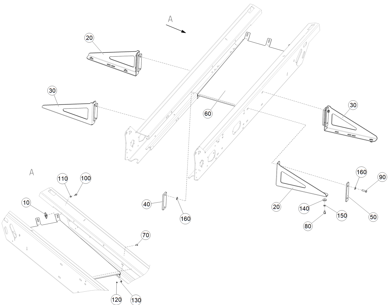
Рис. 1 ЕТВ-6000000261 (Крепление канистр и защитная пластина)
