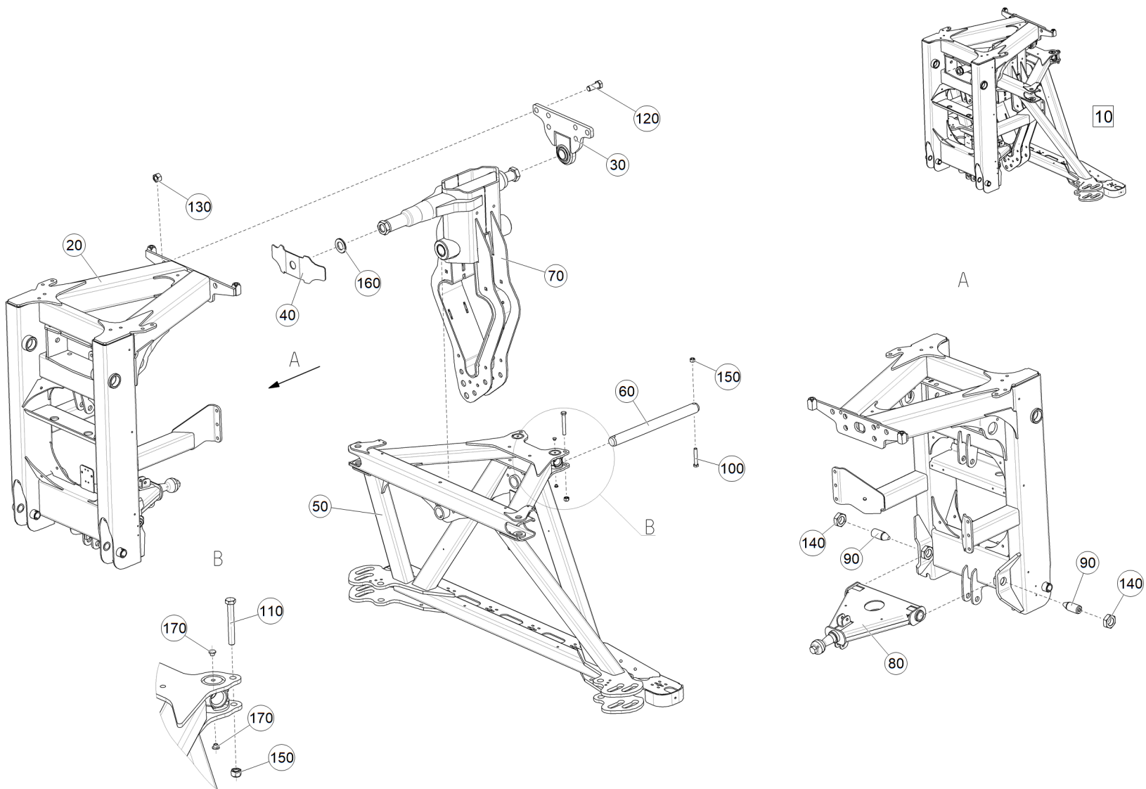
Рис. 1 ЕТВ-6000000345 (Компенсатор колебаний L2/L3 VORM.(02/K5))
