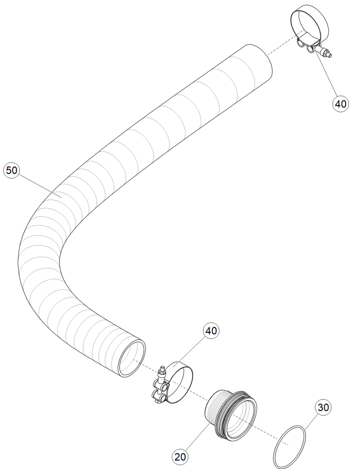
Рис. 1 ЕТВ-6000000308 (Шланг всасывающий)
