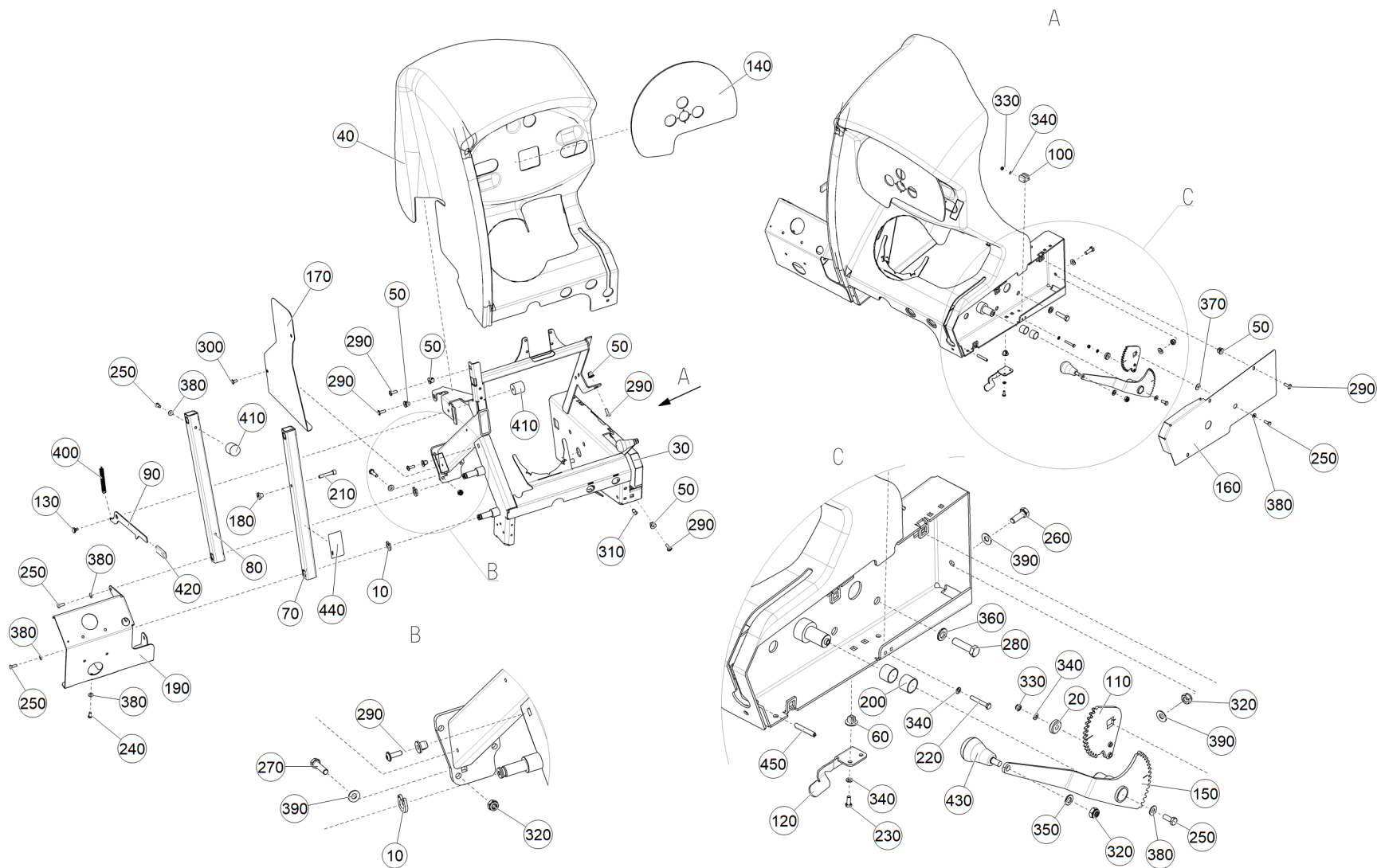
Рис. 1 ETB-6000000267 (Каркас)
