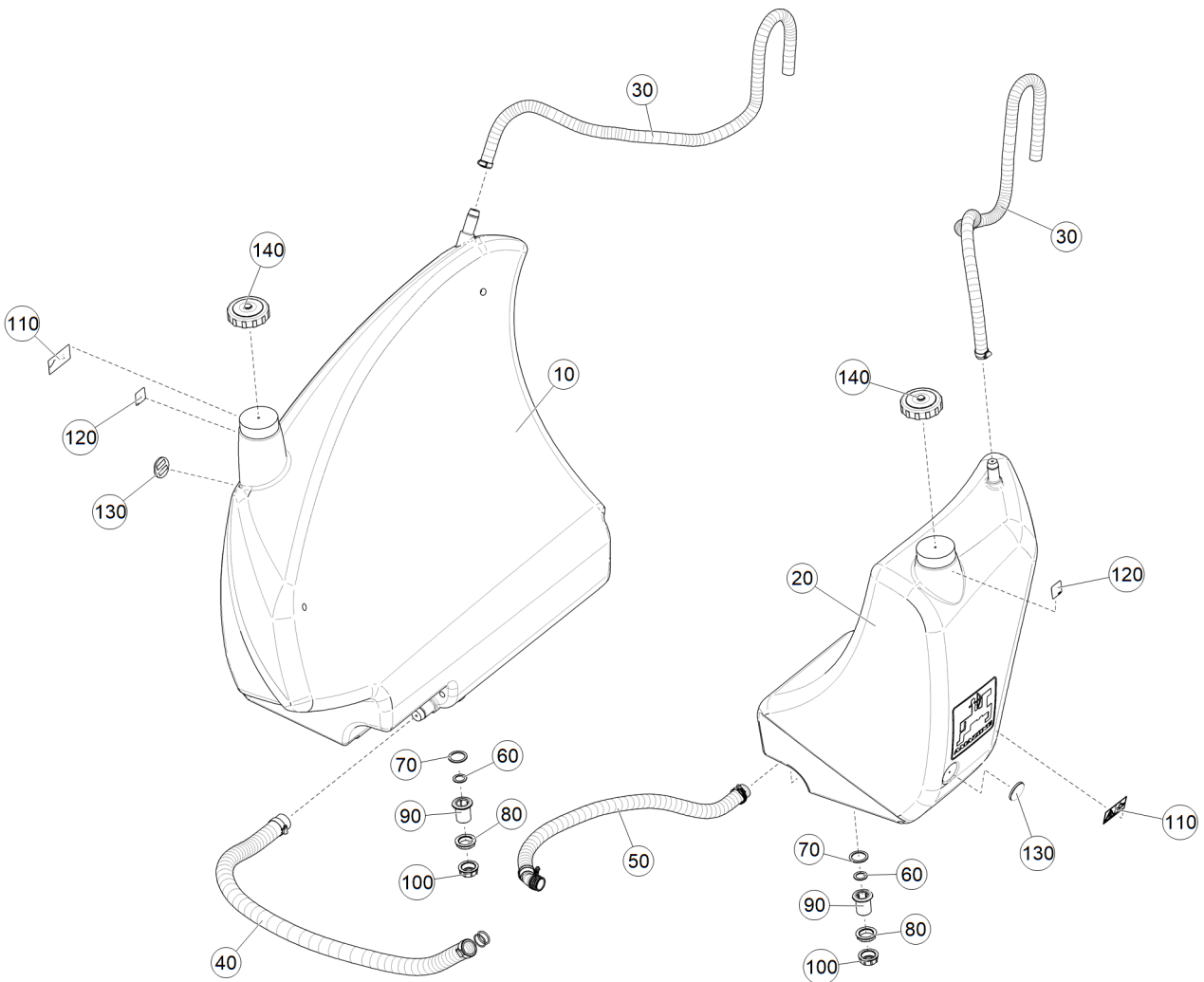
Рис. 1 ЕТВ-6000000272 (Канистры чистой воды)
