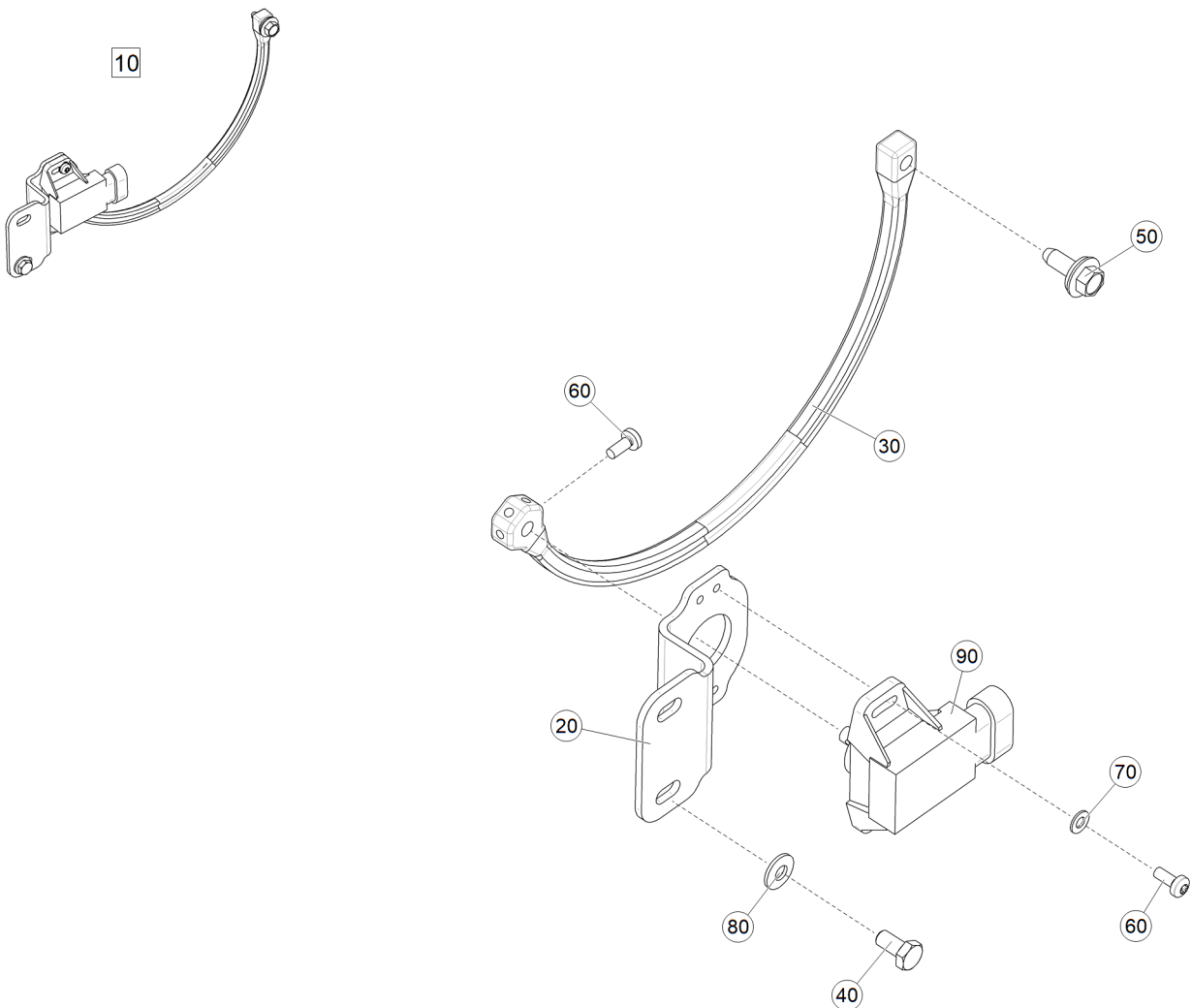
Рис. 1 ЕТВ-6000000348 (Потенциометр VORM.)
