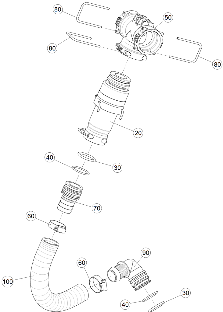
Рис. 1 ЕТВ-6000000315 (Шланг сливной DBV)
