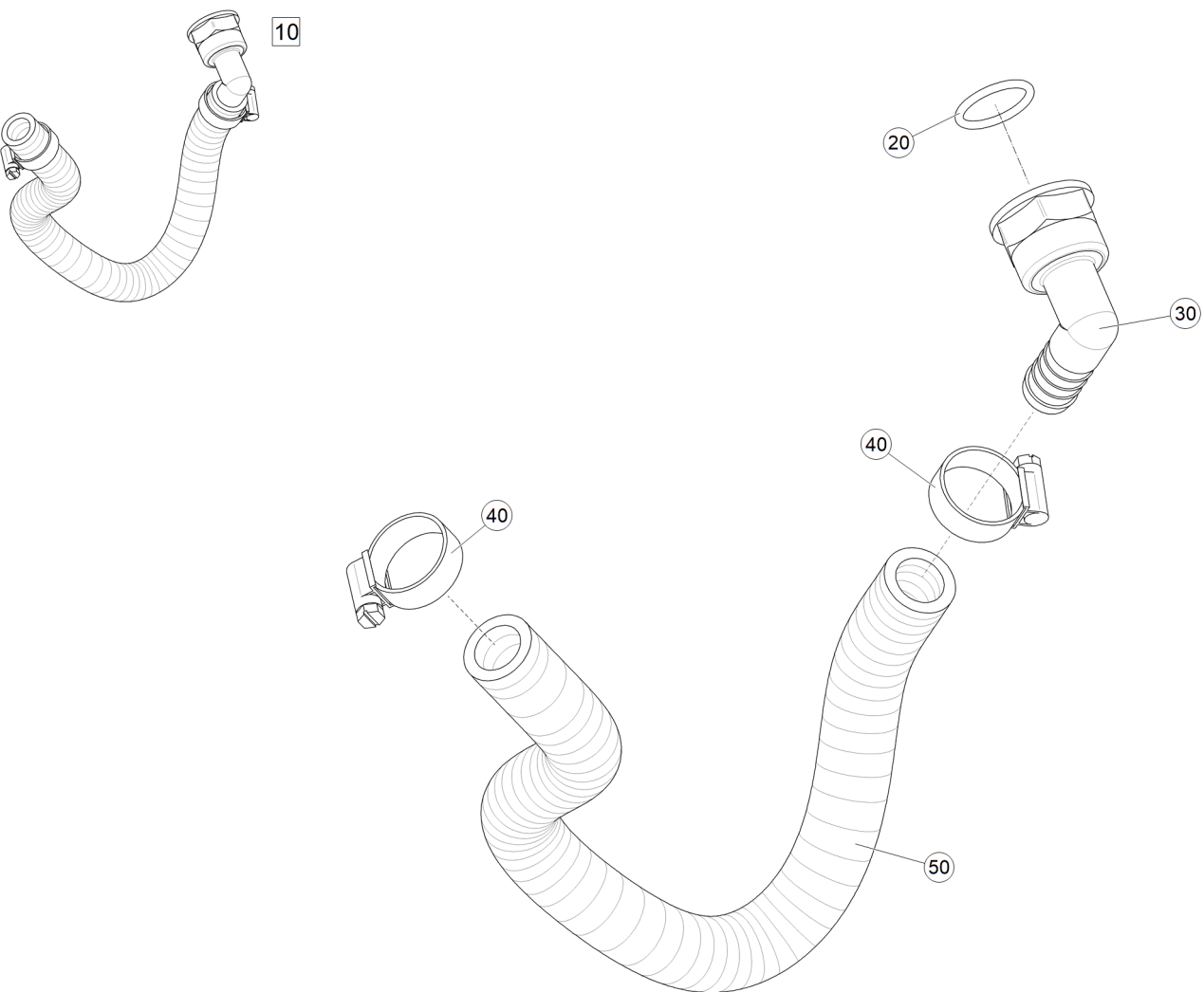
Рис. 1 ЕТВ-6000000317 (Шланг 19X4X440 VORM.)
