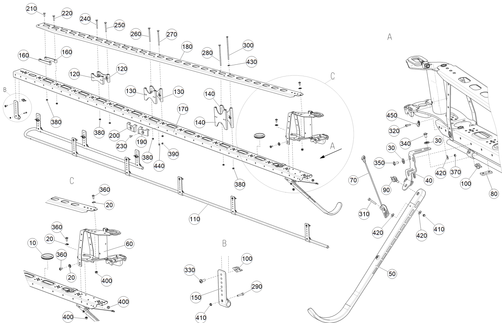
Рис. 1 ЕТВ-6000000287 (Правый край)
