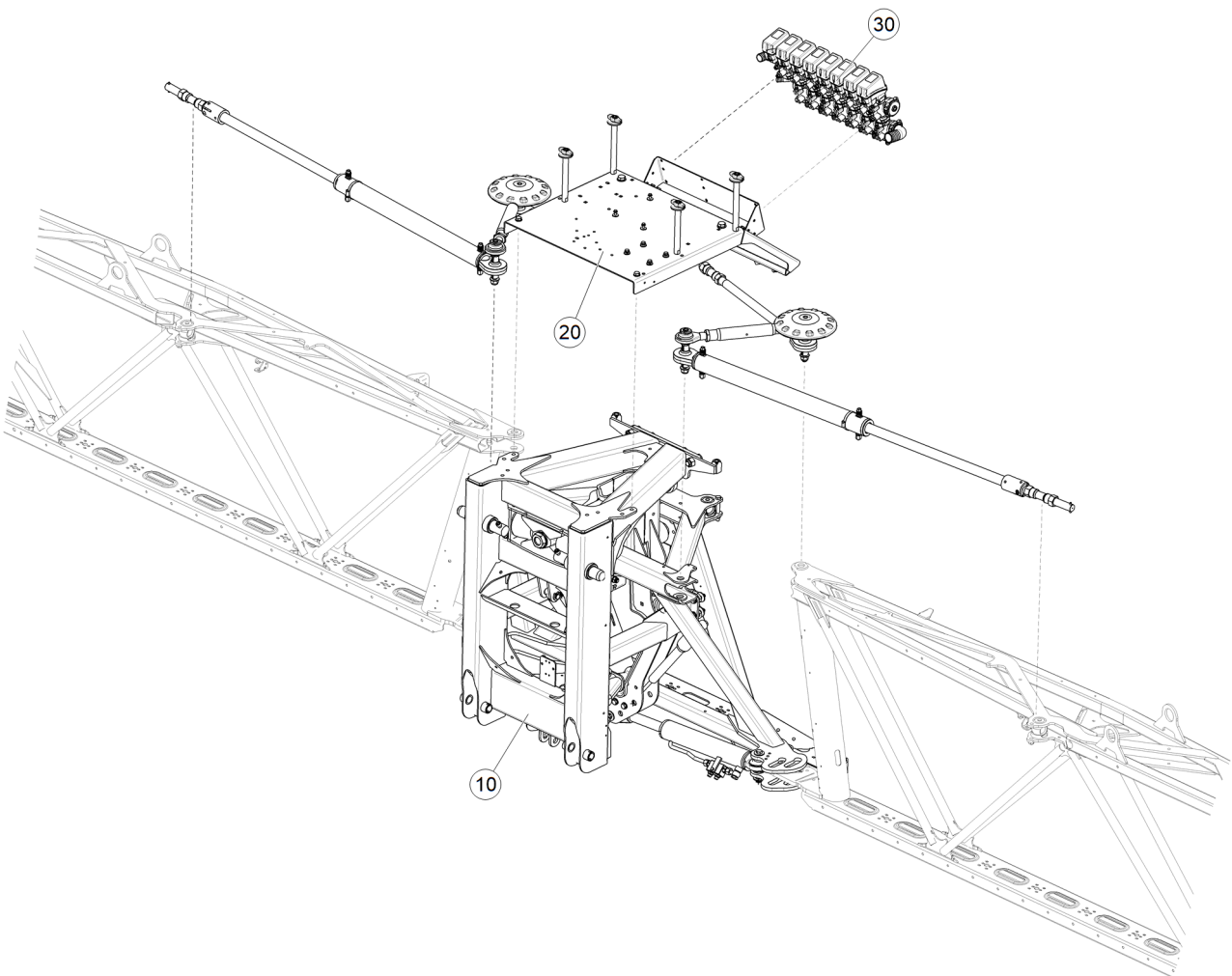
Рис. 1 ETB-6000000275 (Стабилизатор)
