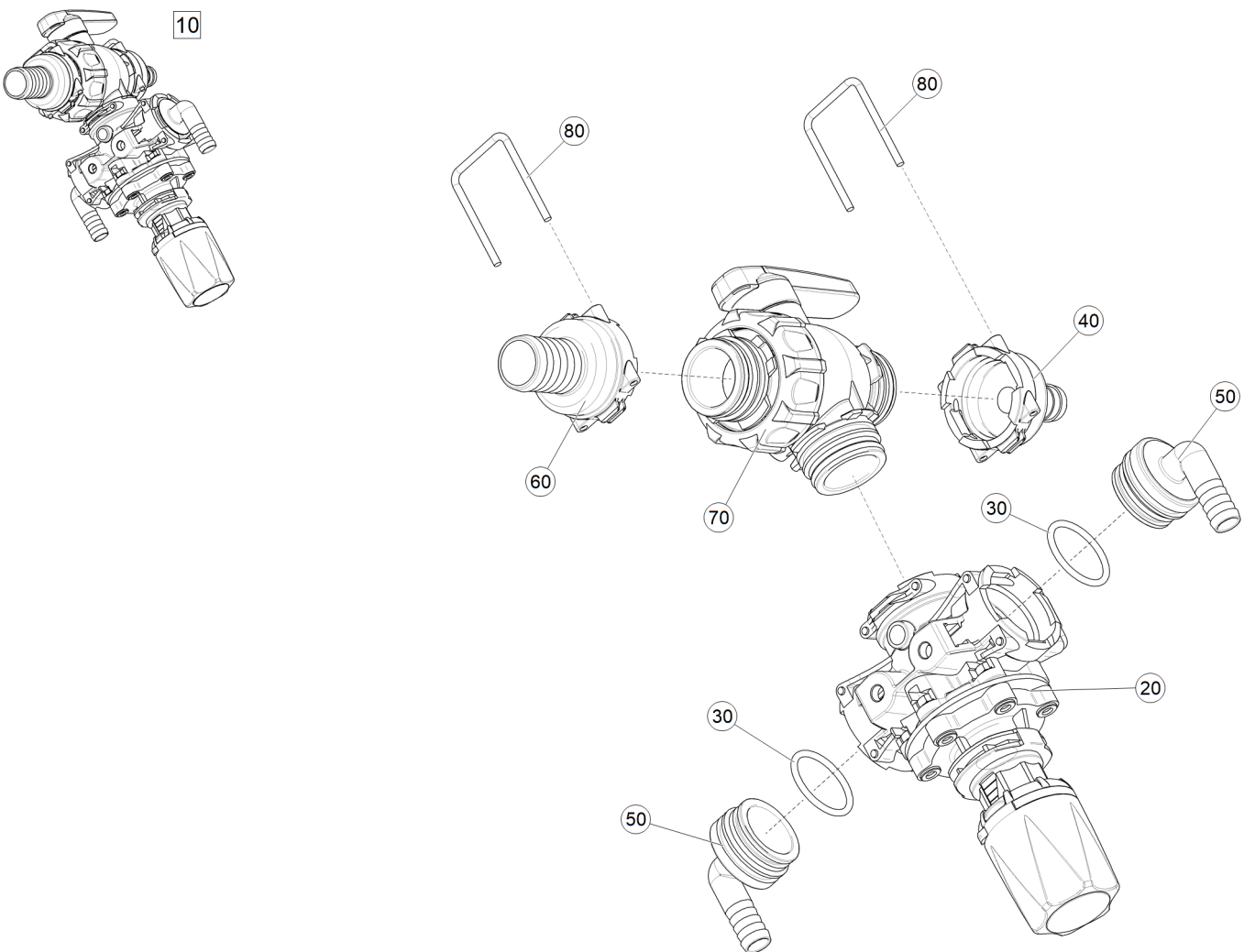
Рис. 1 ЕТВ-60000000338 (Клапан редукционный с краном)
