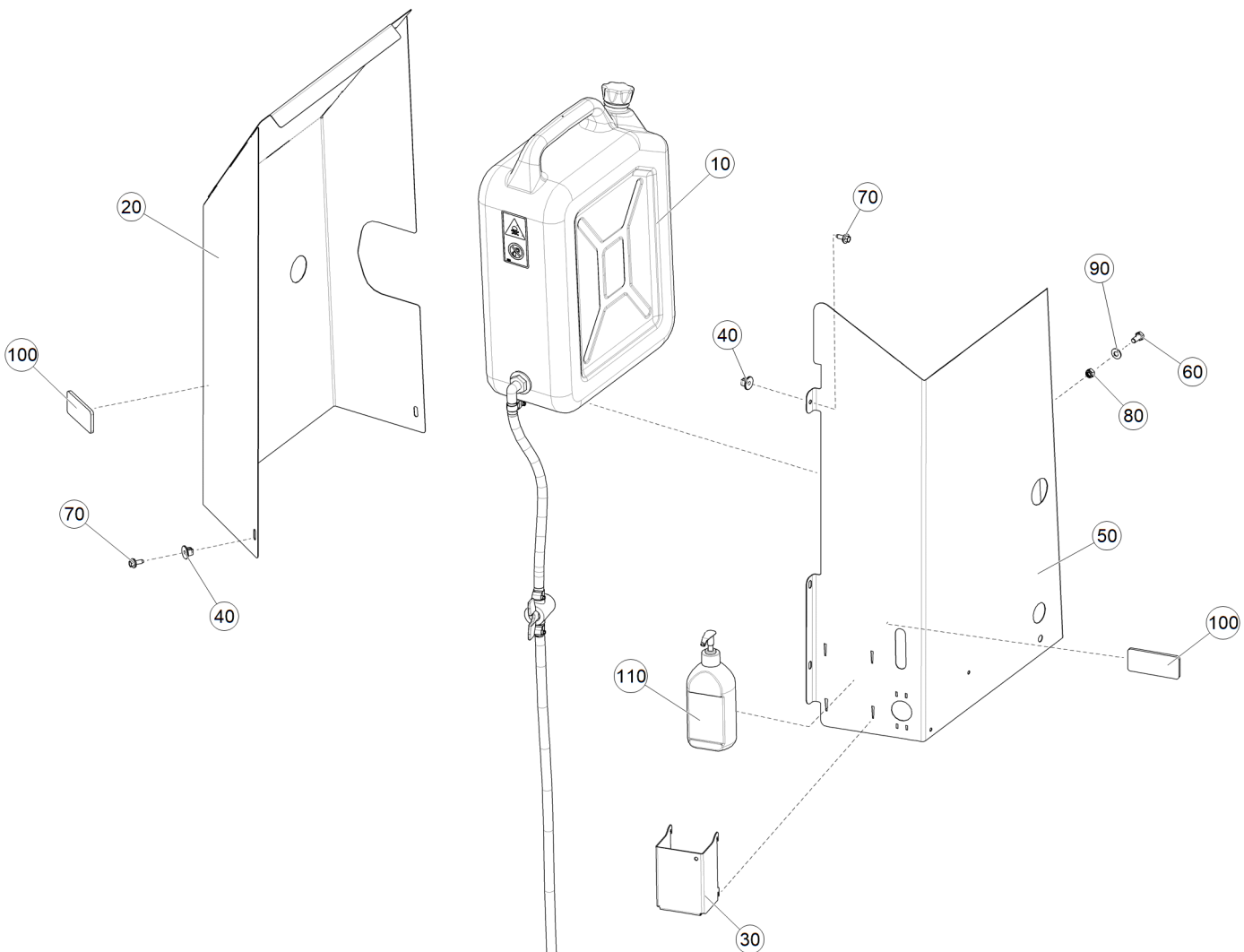
Рис. 1 ETV-6000000265 (Крепление обвесов)
