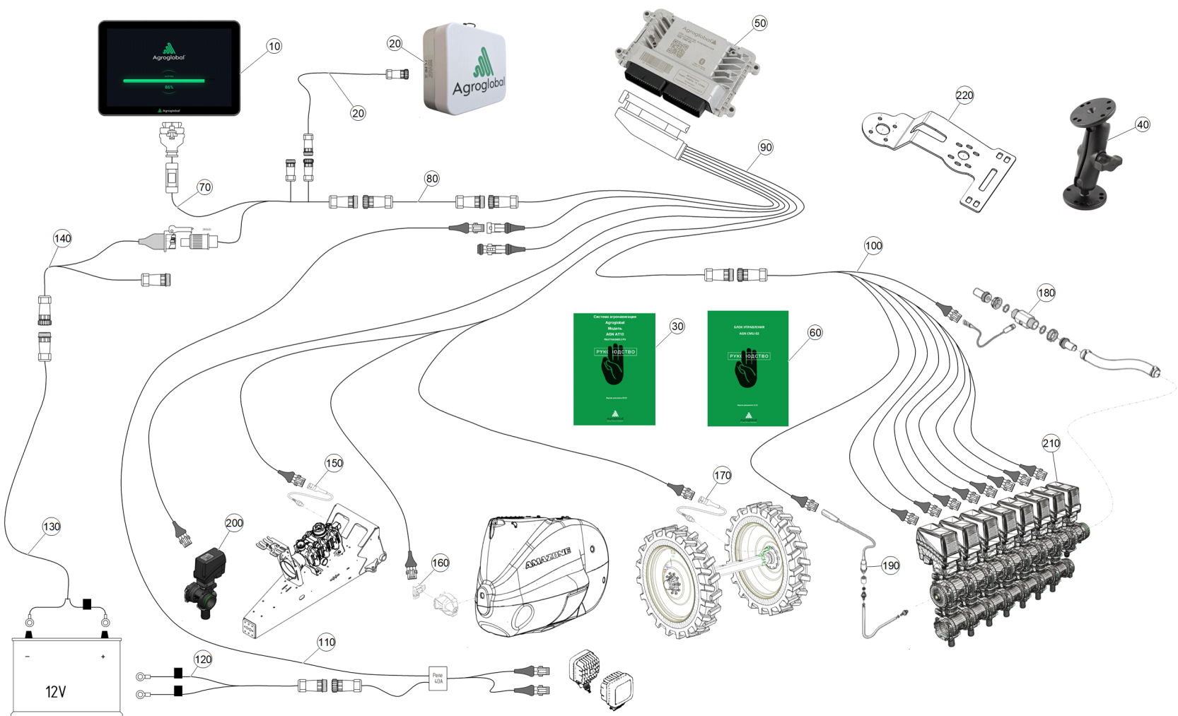
Рис. 1 ЕТВ-6000000167 (Электроника Агроглобал)
