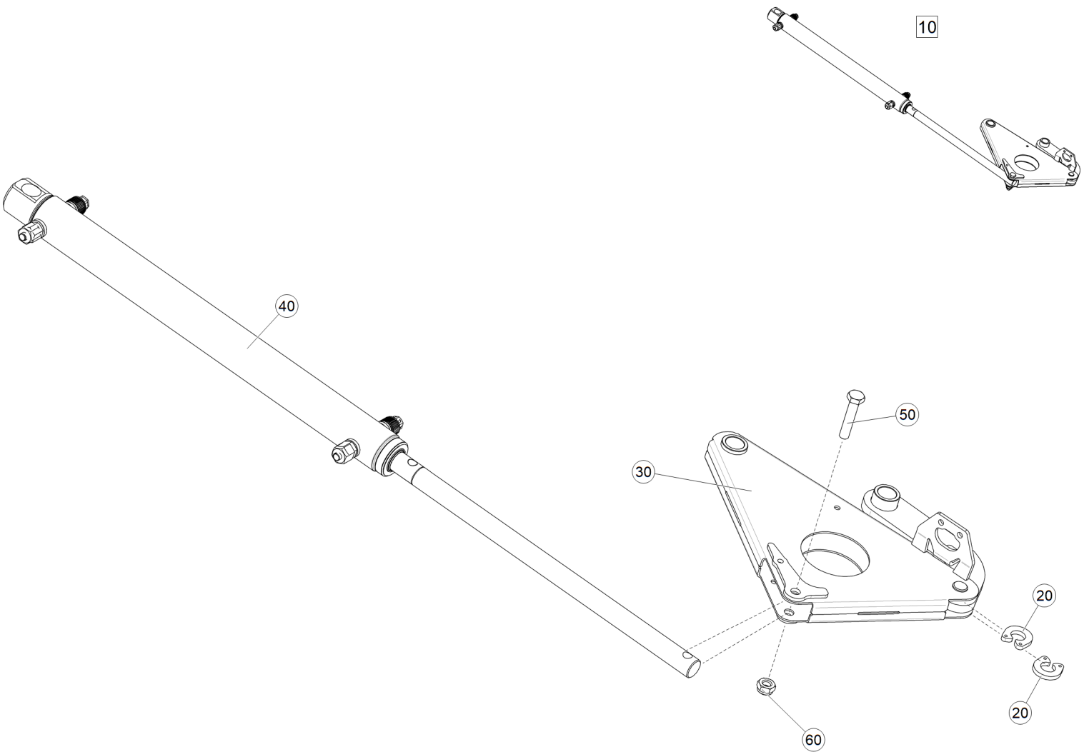
Рис. 1 ЕТВ-6000000379 (Рычаг поворотный внутр левый)
