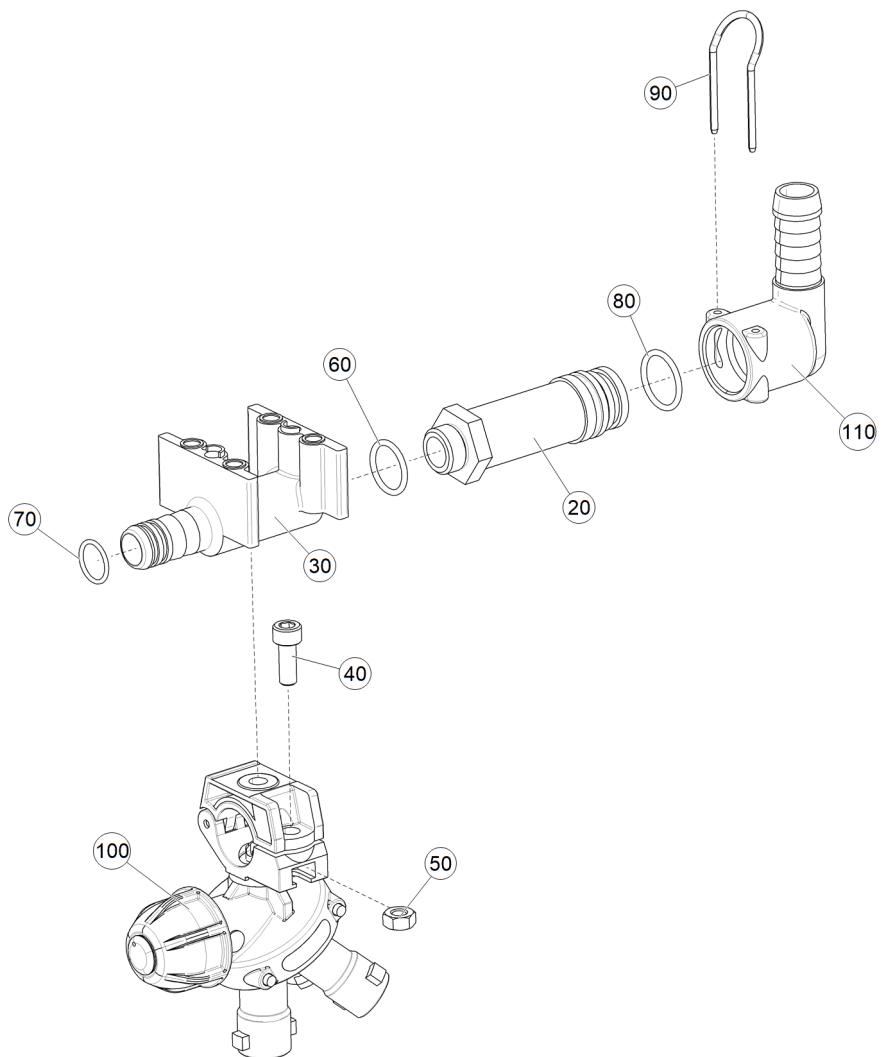
Рис. 1 ЕТВ-60000000355 (Корпус крепл форсунок 3-FACH LANG)
