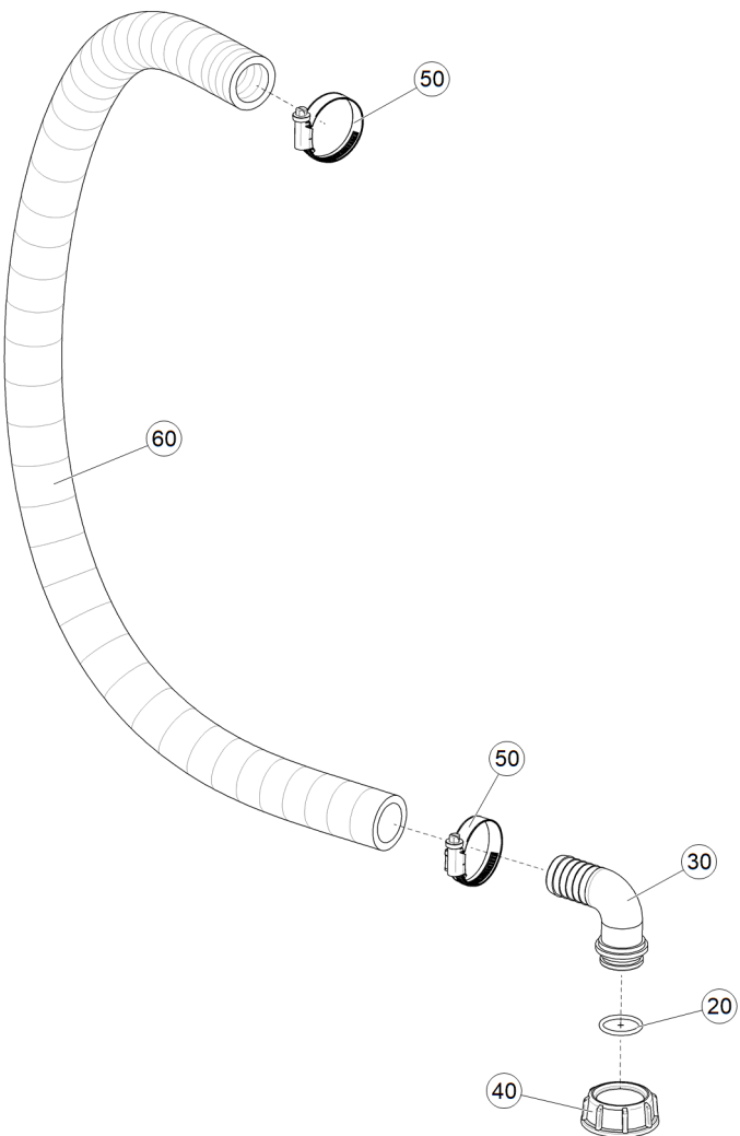
Рис. 1 ЕТВ-60000000331 (Шланг 28X6X1000 VORM.)
