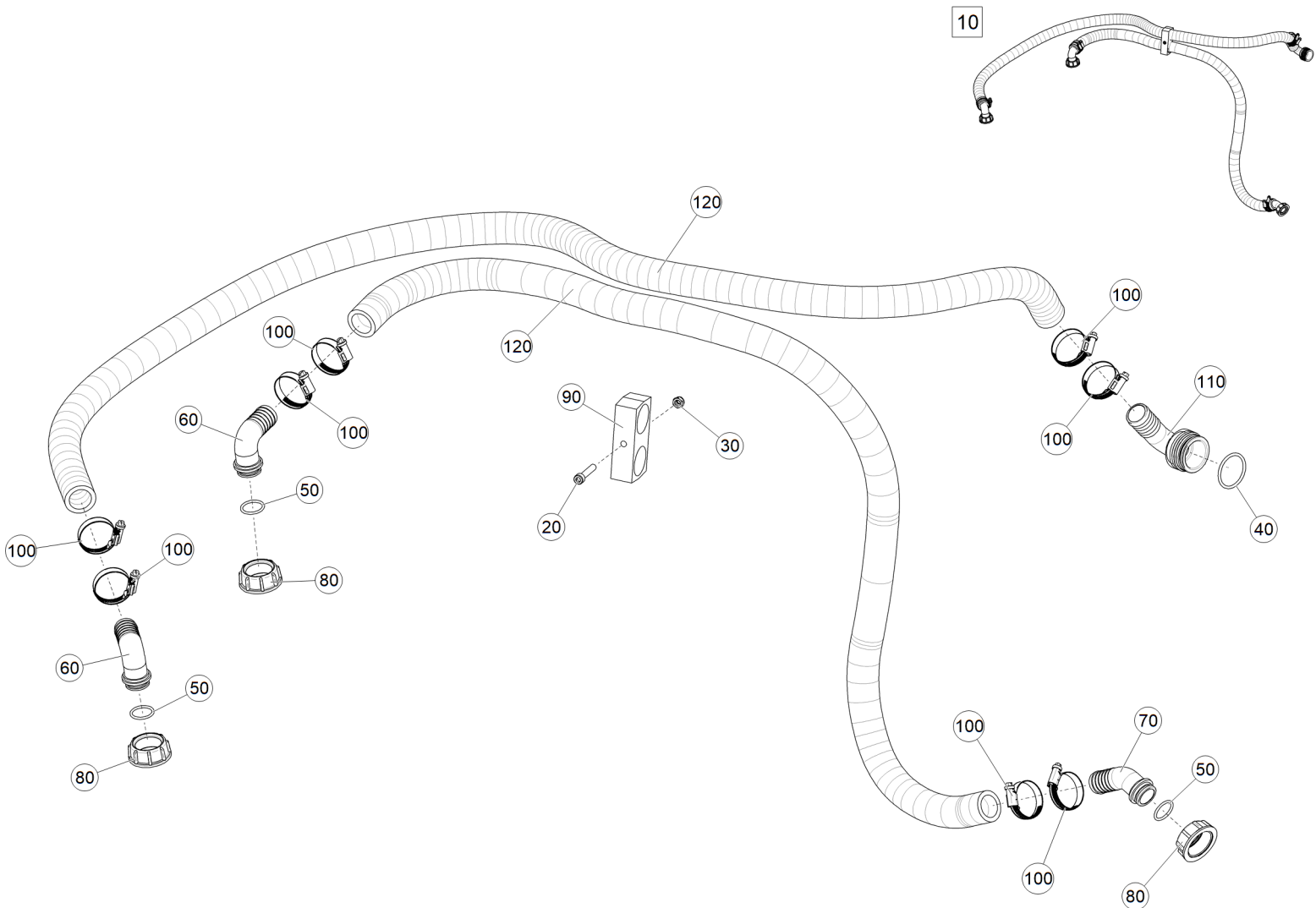
Рис. 1 ЕТВ-6000000296 (Шланги)
