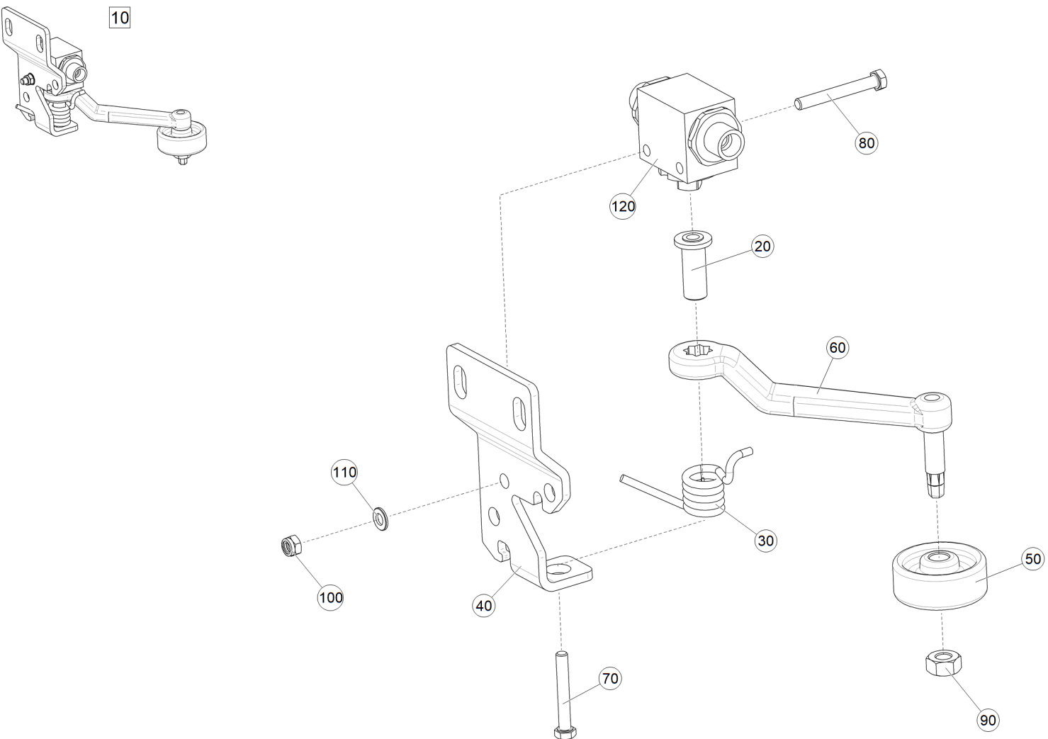
Рис. 1 ЕТВ-6000000375 (Кран гидравлический правый)
