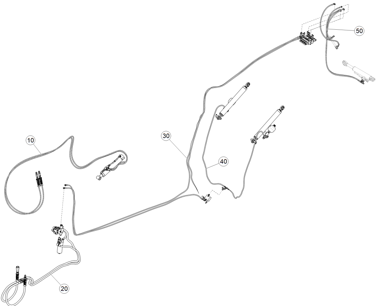
Рис. 1 ЕТВ-6000000356 (База)
