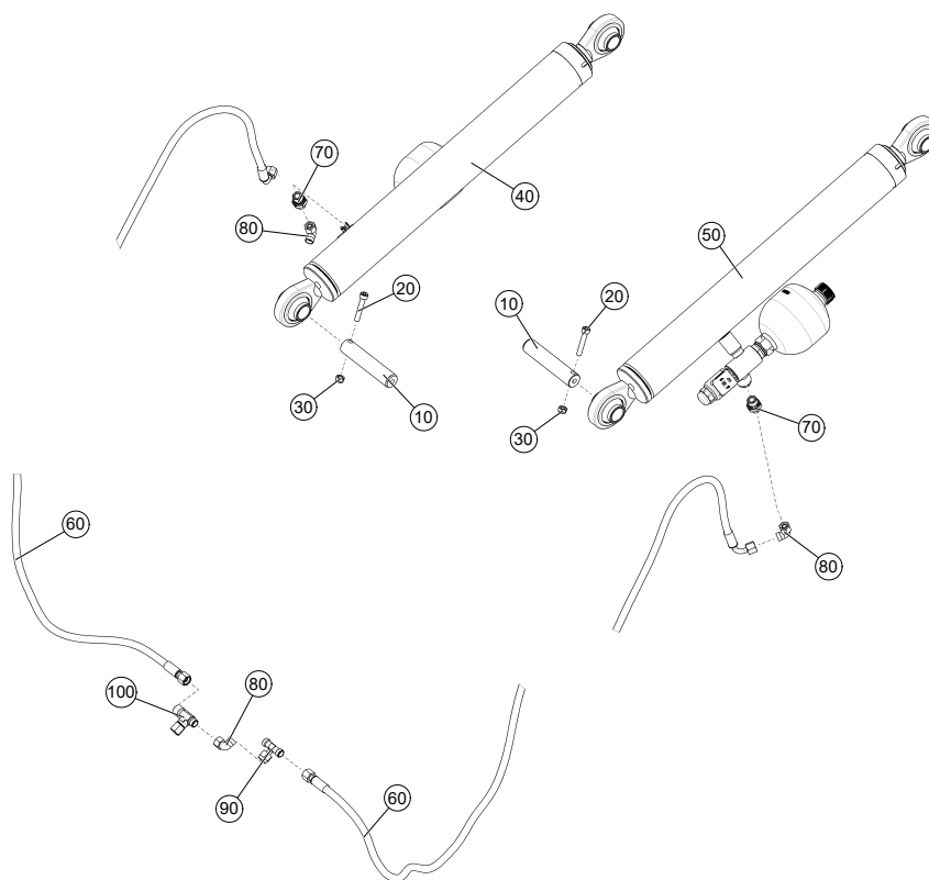
Рис. 1 ЕТВ-6000000360 (Линия маятника)
