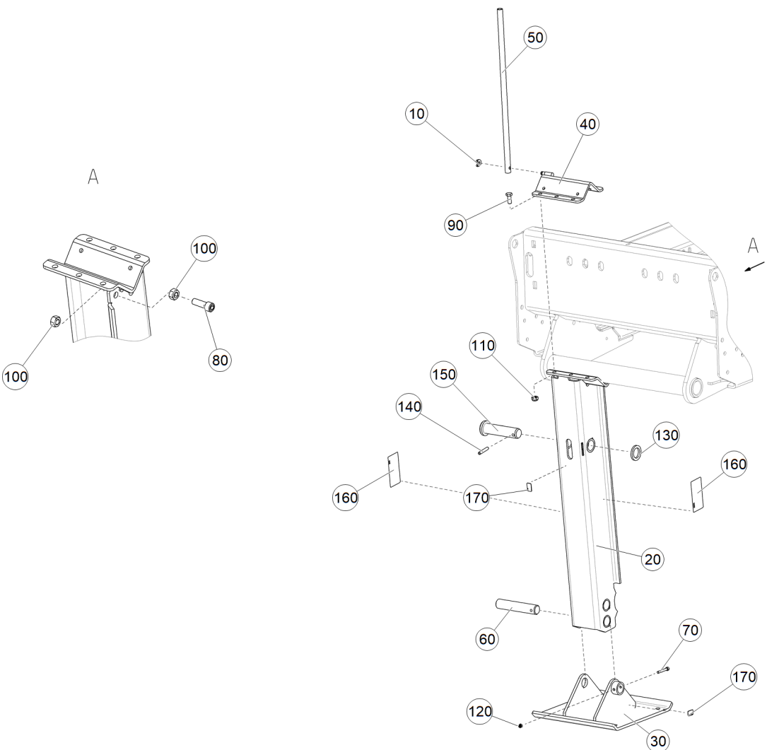
Рис. 1 ЕТВ-6000000262 (Опора гидравлическая)
