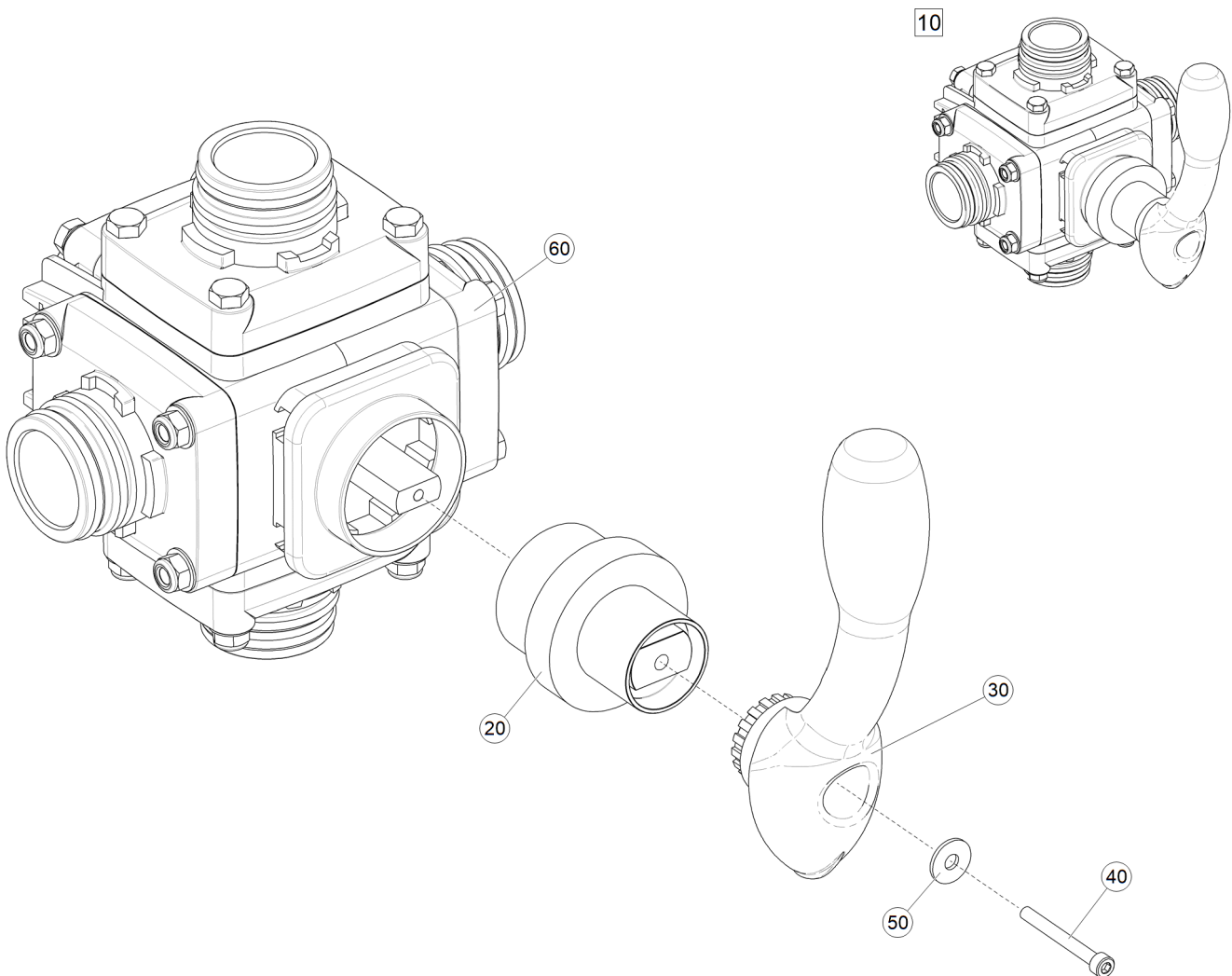
Рис. 1 ЕТВ-6000000312 (Кран 5-ходовой шаровый с ручкой AMAZONE)
