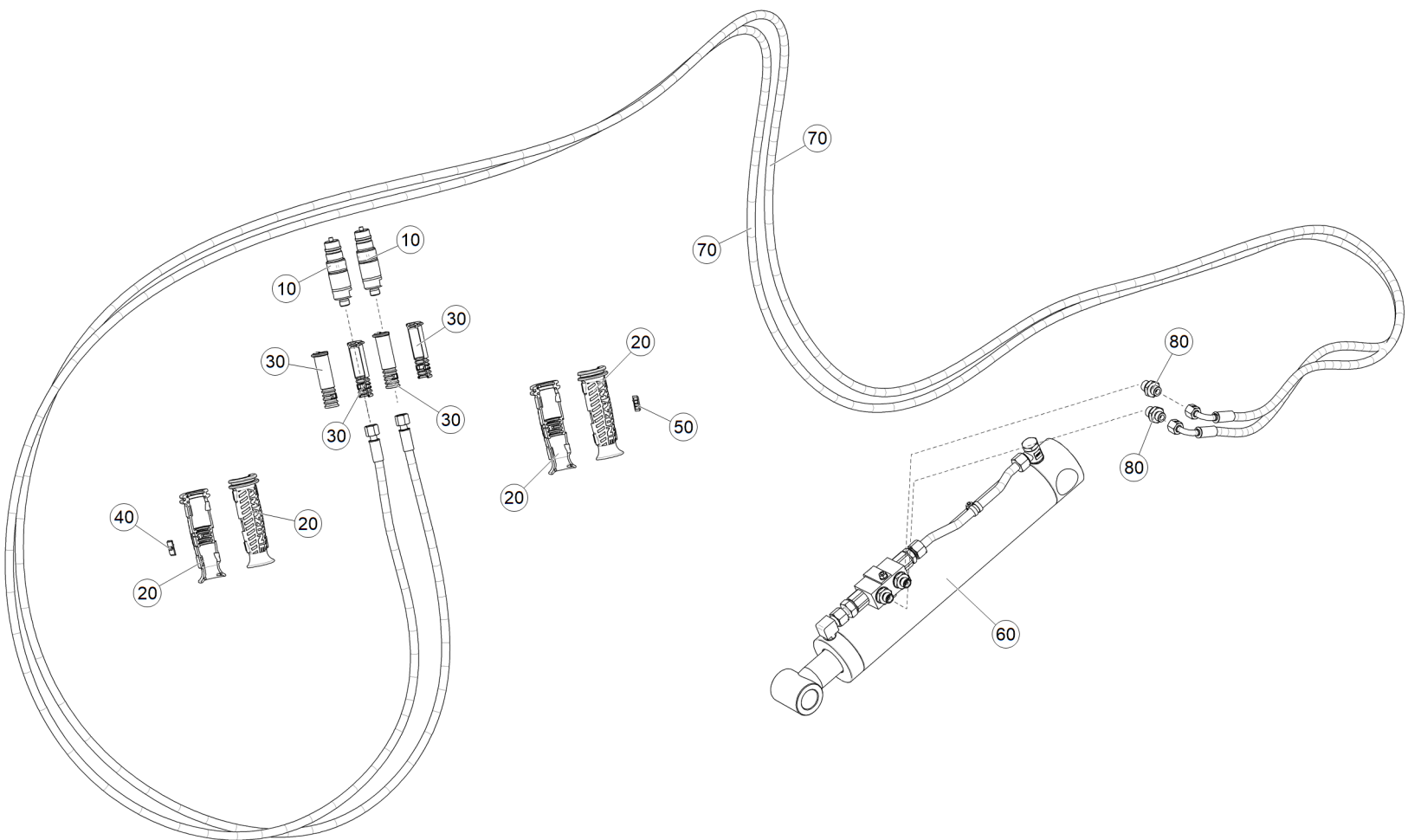
Рис. 1 ЕТВ-60000000357 (Линия опоры гидравлической)
