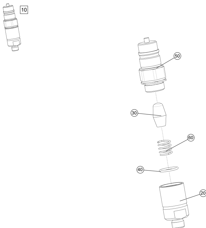
Рис. 1 ЕТВ-6000000362 (Муфта быстросъемная 12,5 с фильтром)
