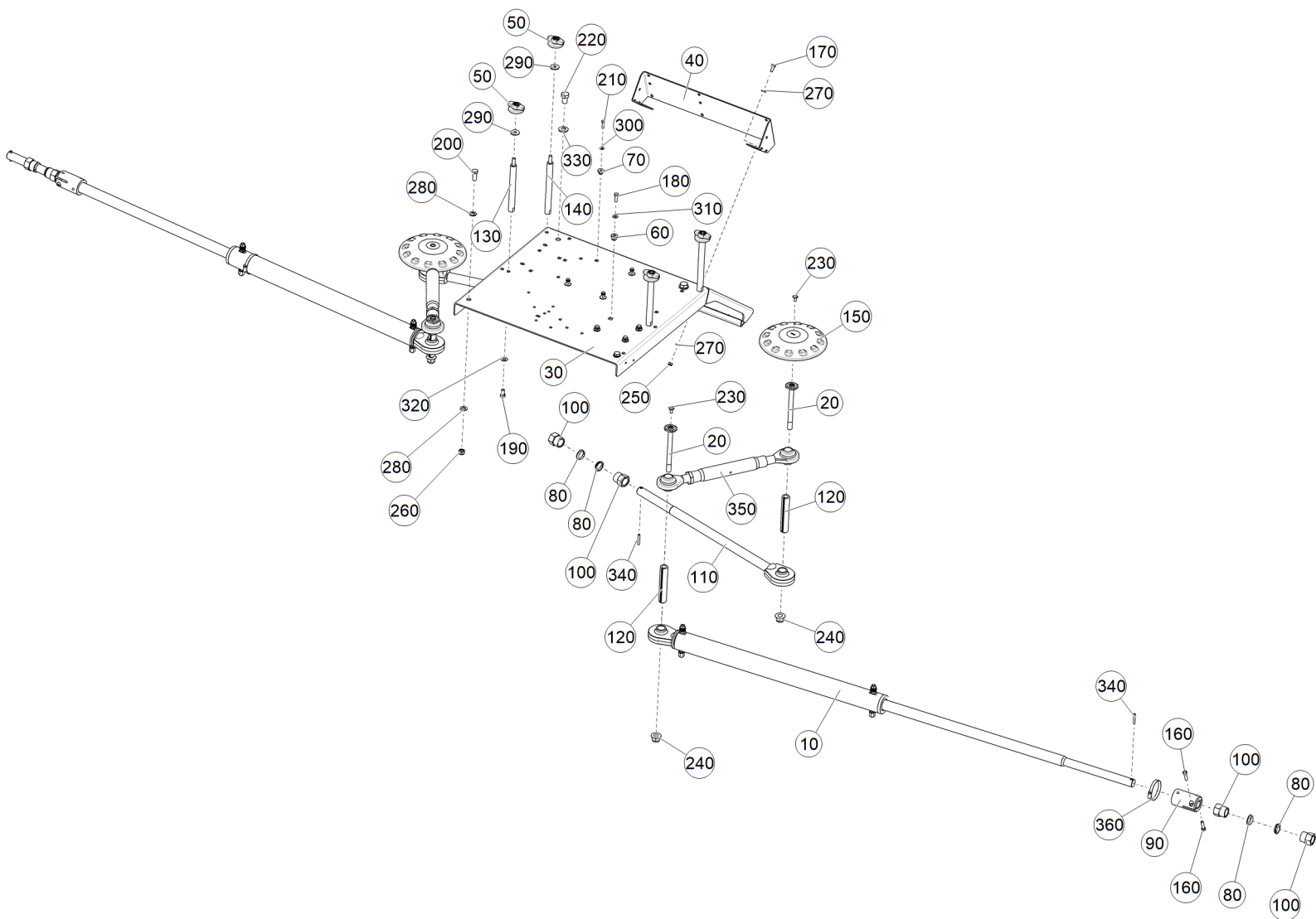
Рис. 1 ETV-6000000277 (Крепление крышки и соединение с штангой)
