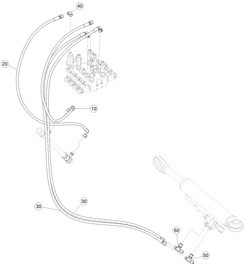
Рис. 1 ЕТВ-6000000361 (Линия стабилизатора)
