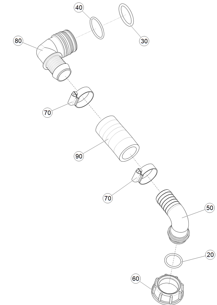
Рис. 1 ЕТВ-6000000337 (Шланг 28X6X85 перед.)
