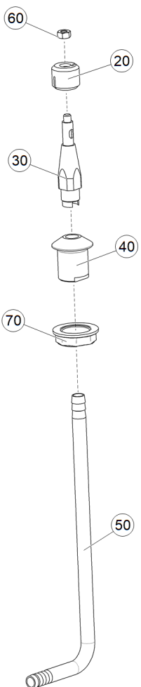
Рис. 1 ЕТВ-6000000333 (Форсунка промывочная)
