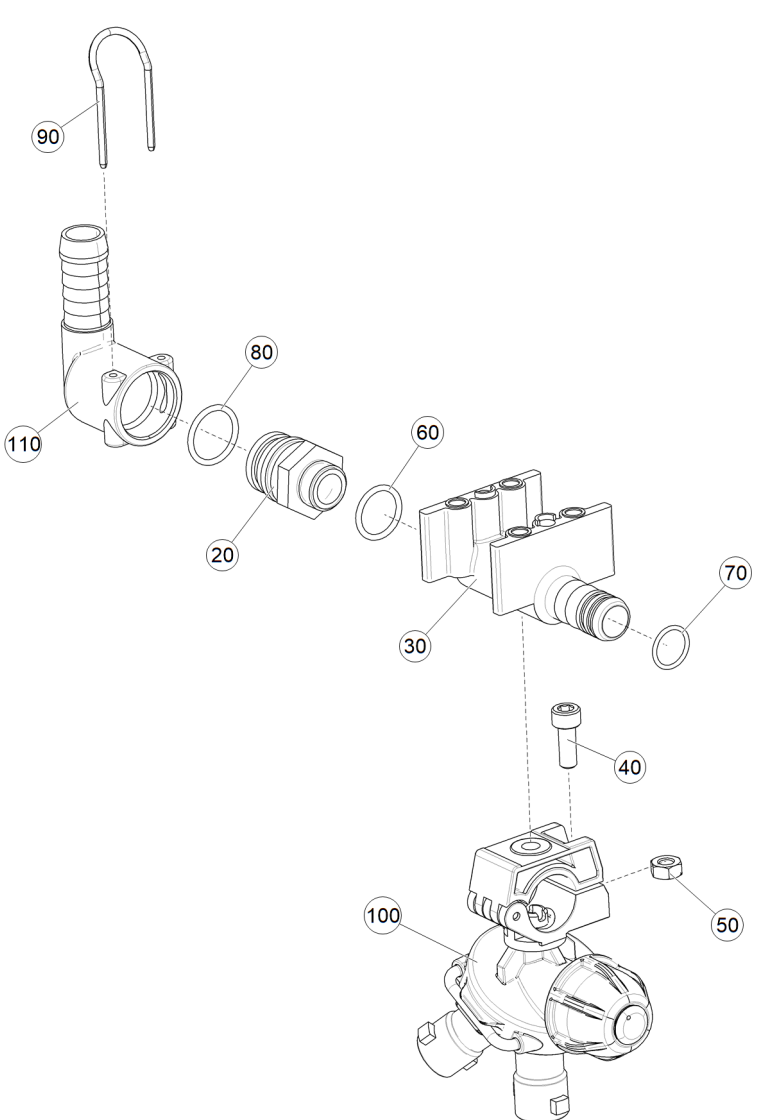
Рис. 1 ЕТВ-6000000350 (Корпус 3-точечной форсунки с уголком 90)
