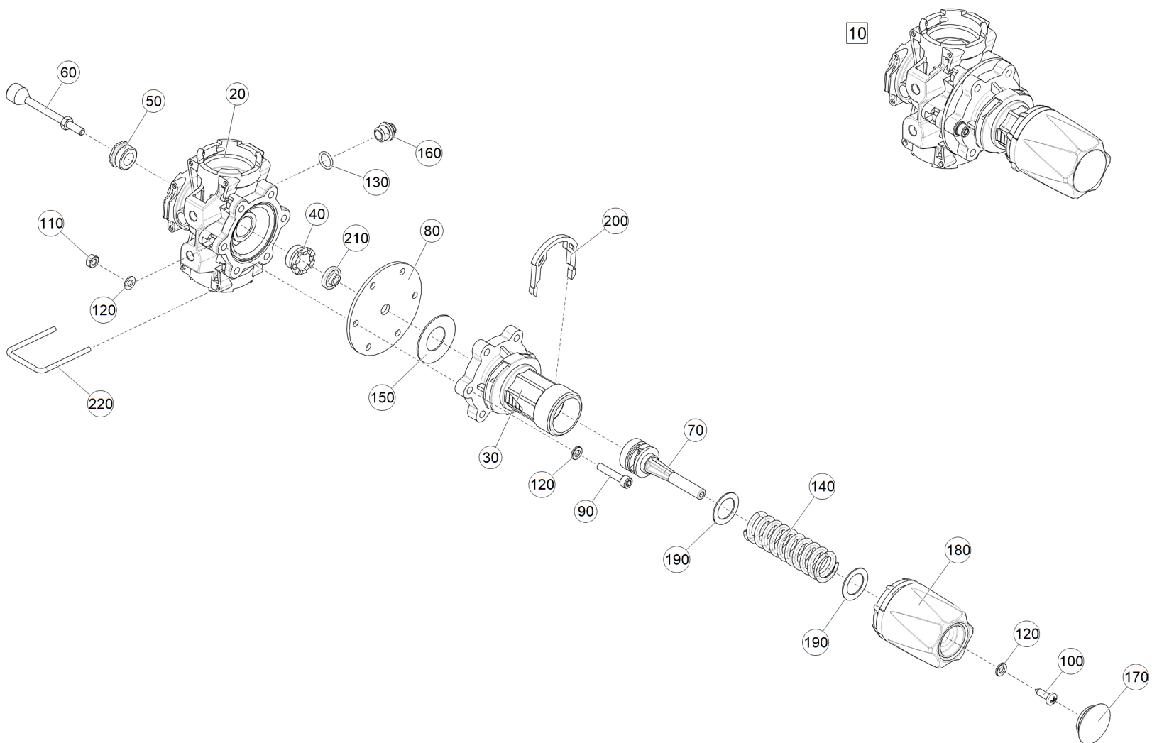
Рис. 1 ЕТВ-6000000339 (Клапан редукционный)
