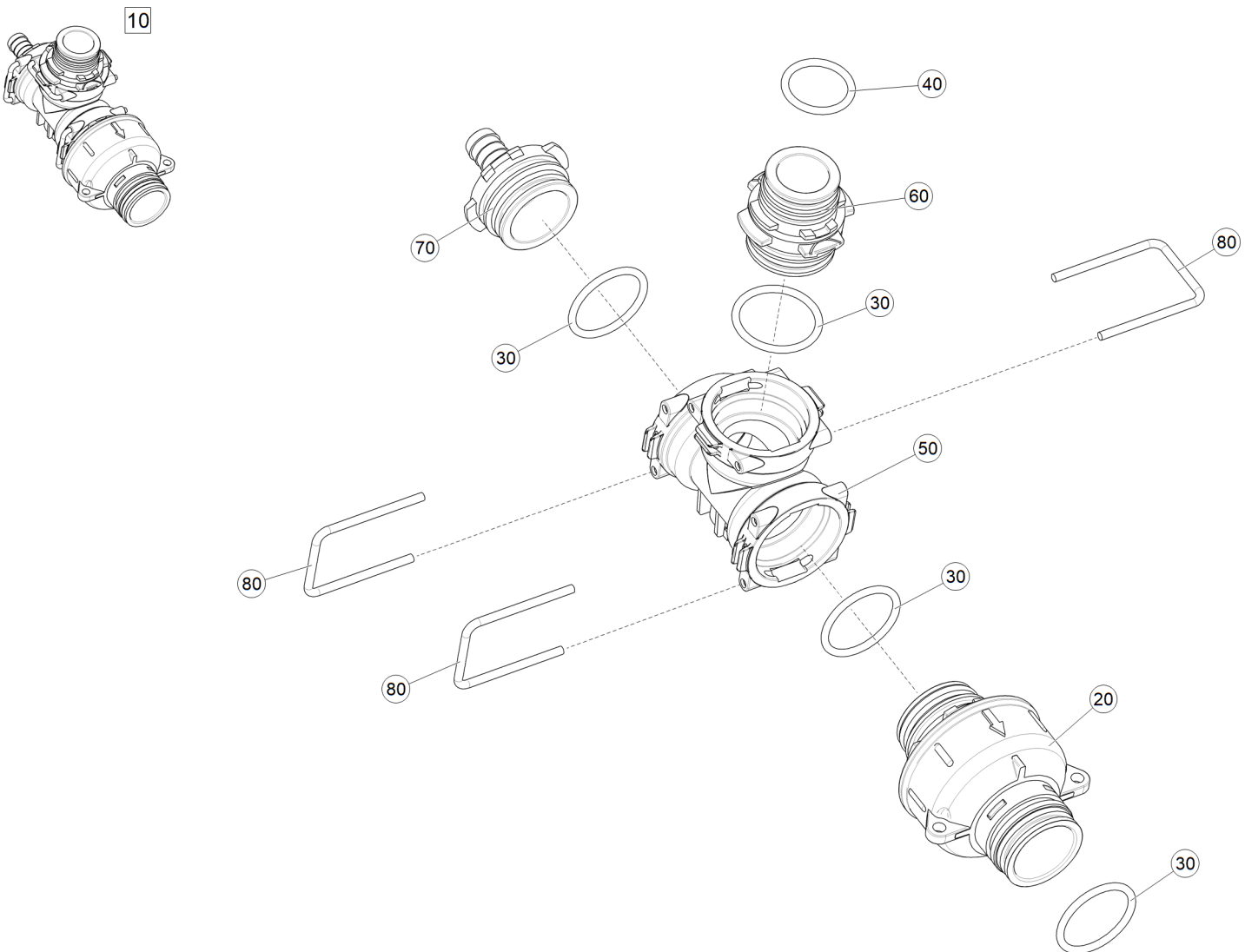
Рис. 1 ЕТВ-6000000304 (Клапан давления)
