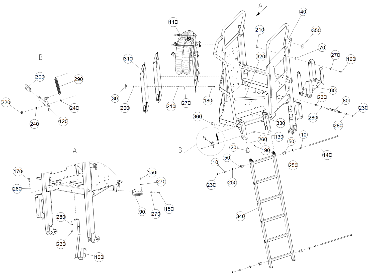
Рис. 1 ЕТВ-6000000264 (Площадка и лестница)
