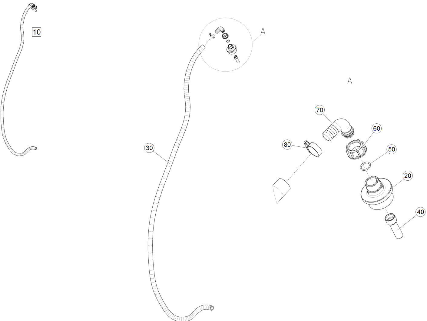
Рис. 1 ЕТВ-6000000330 (Инжектор дозирующий 2 дюйма VORMON)
