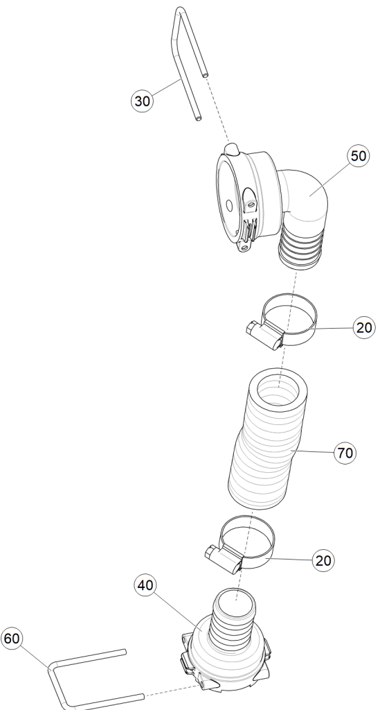
Рис. 1 ETB-6000000314 (Шланг перед)
