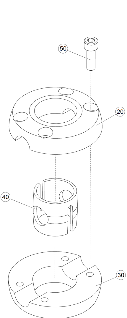
Рис. 1 ЕТВ-6000000349 (Шарнир VORM.)
