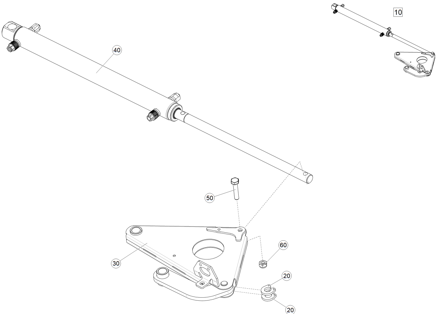
Рис. 1 ЕТВ-6000000382 (Рычаг поворотный внутрь правый)
