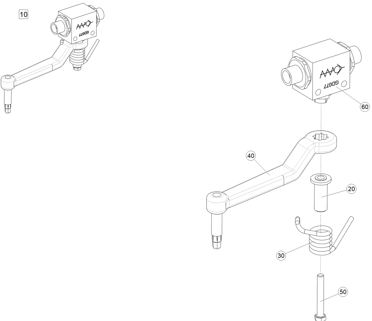
Рис. 1 ЕТВ-6000000376 (Кран гидравлический левый)
