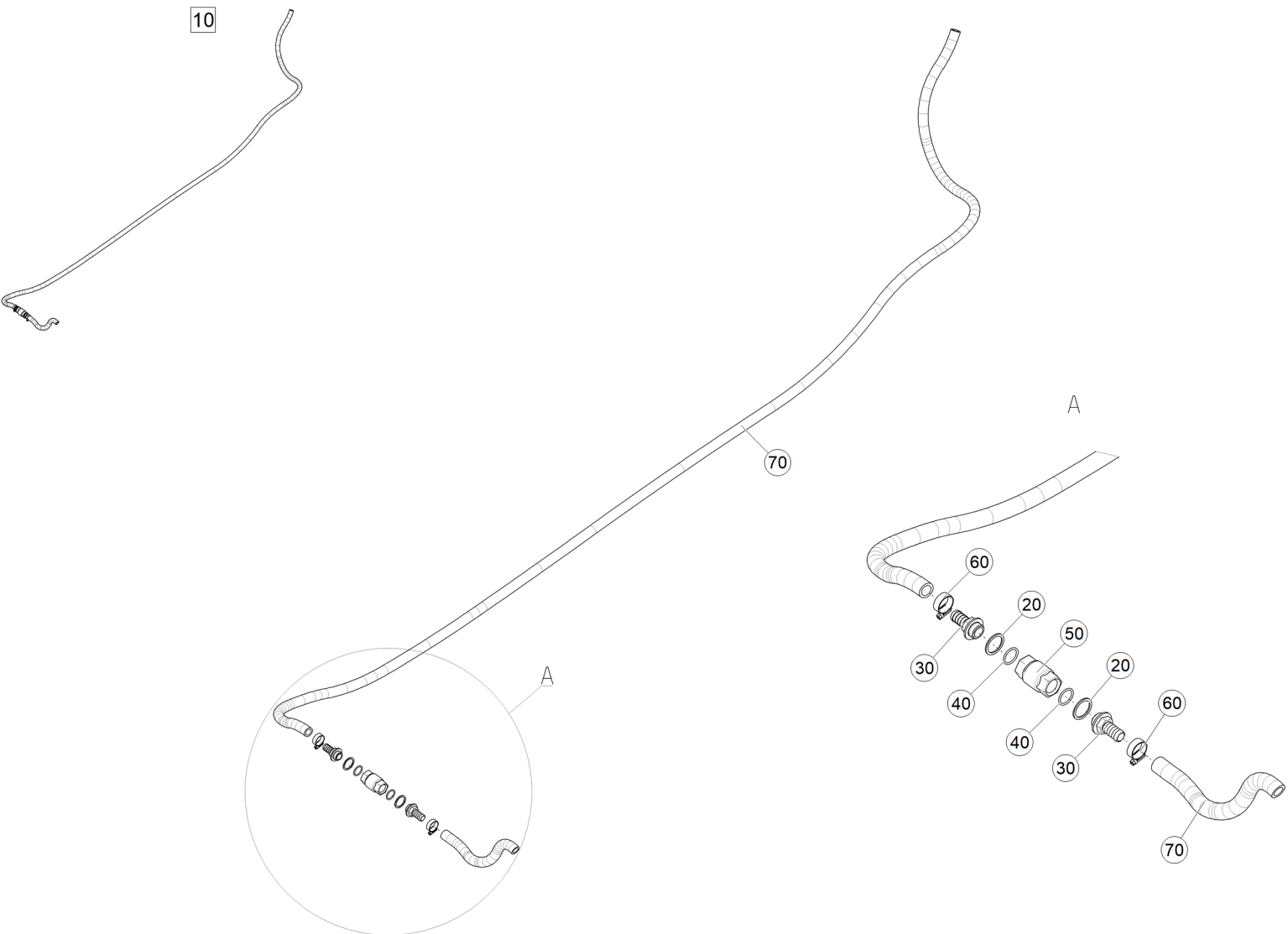
Рис. 1 ЕТВ-6000000320 (Шланг VORM)
