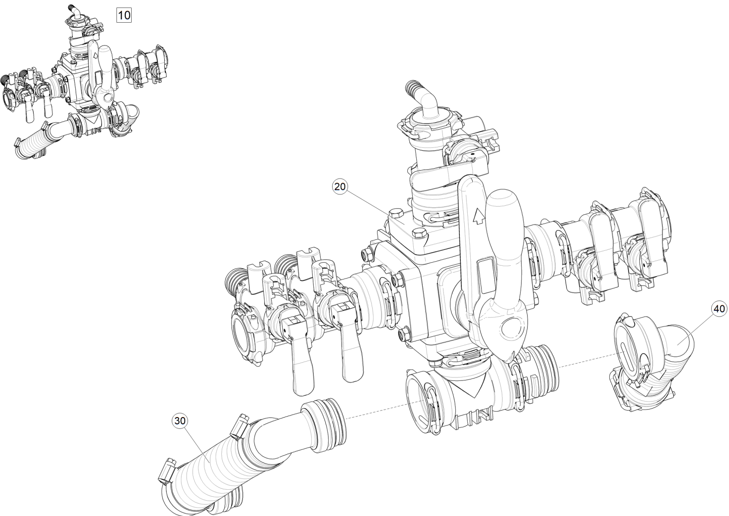
Рис. 1 ЕТВ-6000000310 (Панель управления VORM.)
