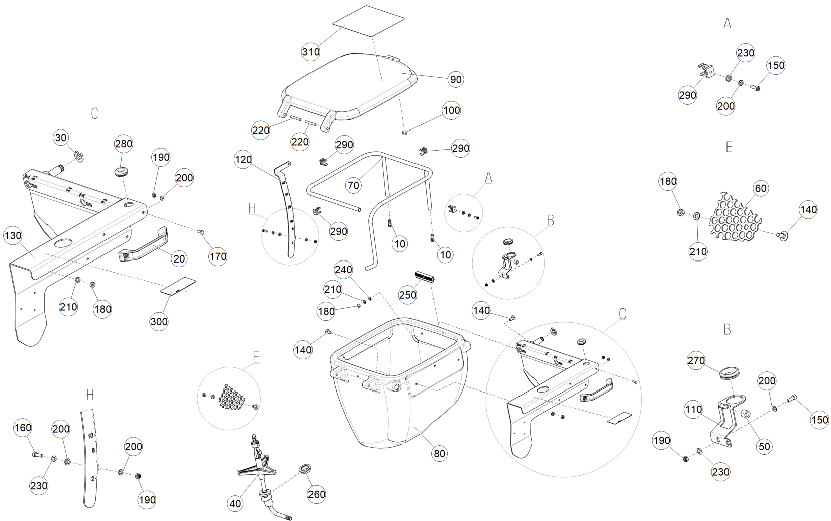
Рис. 1 ЕТВ-6000000273 (Емкость для промывки)
