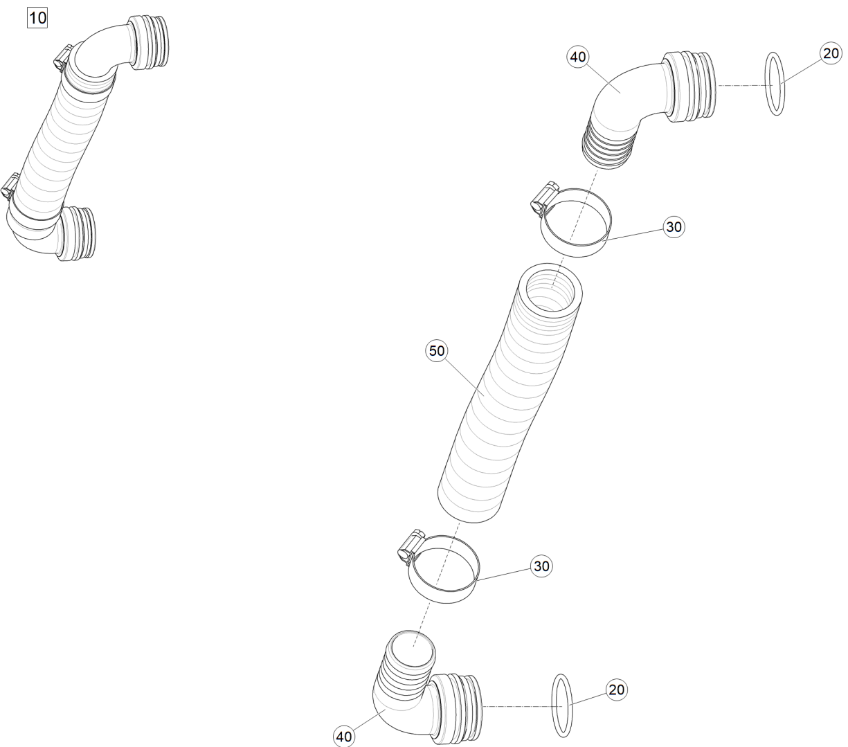
Рис. 1 ЕТВ-6000000313 (Шланг регулятора давления монт.)
