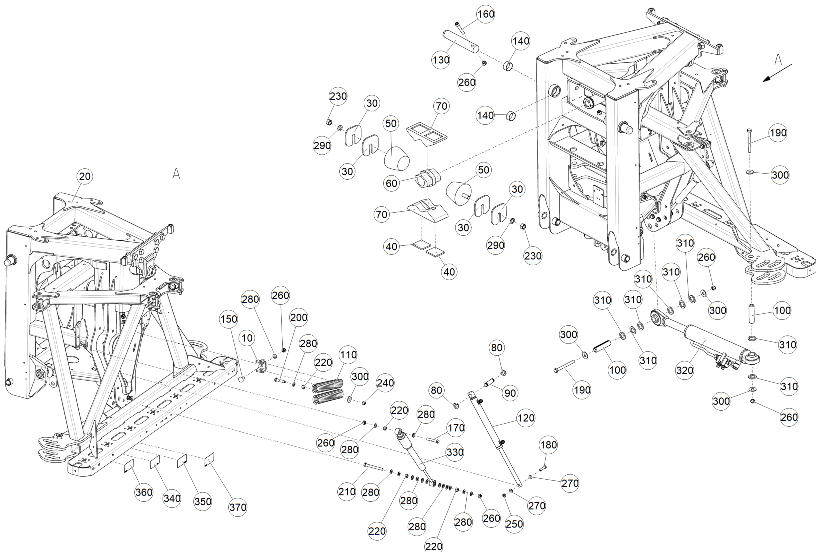
Рис. 1 ЕТВ-6000000276 (Рама подъемная)
