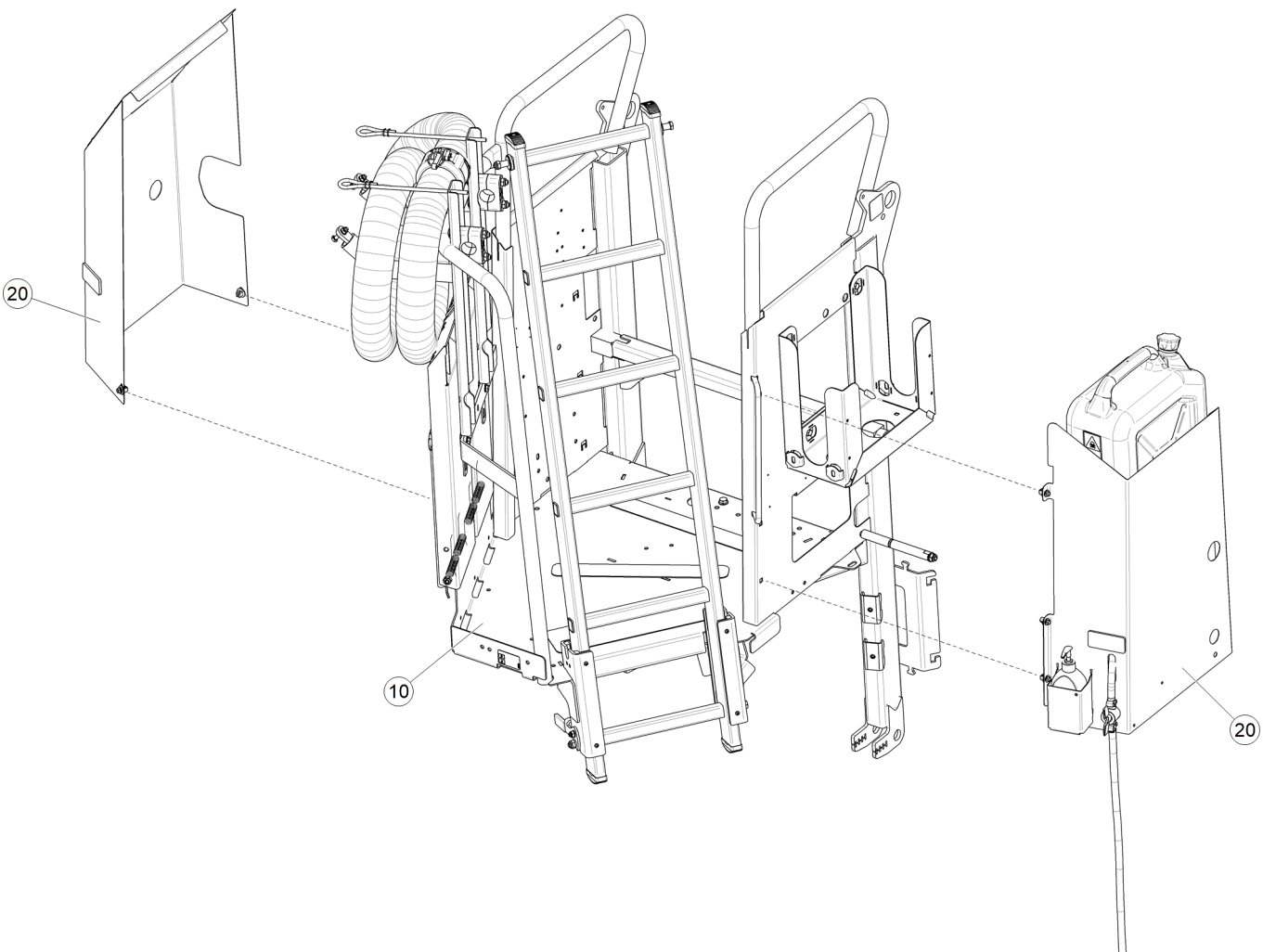
Рис. 1 ЕТВ-6000000263 (Площадка обслуживания)
