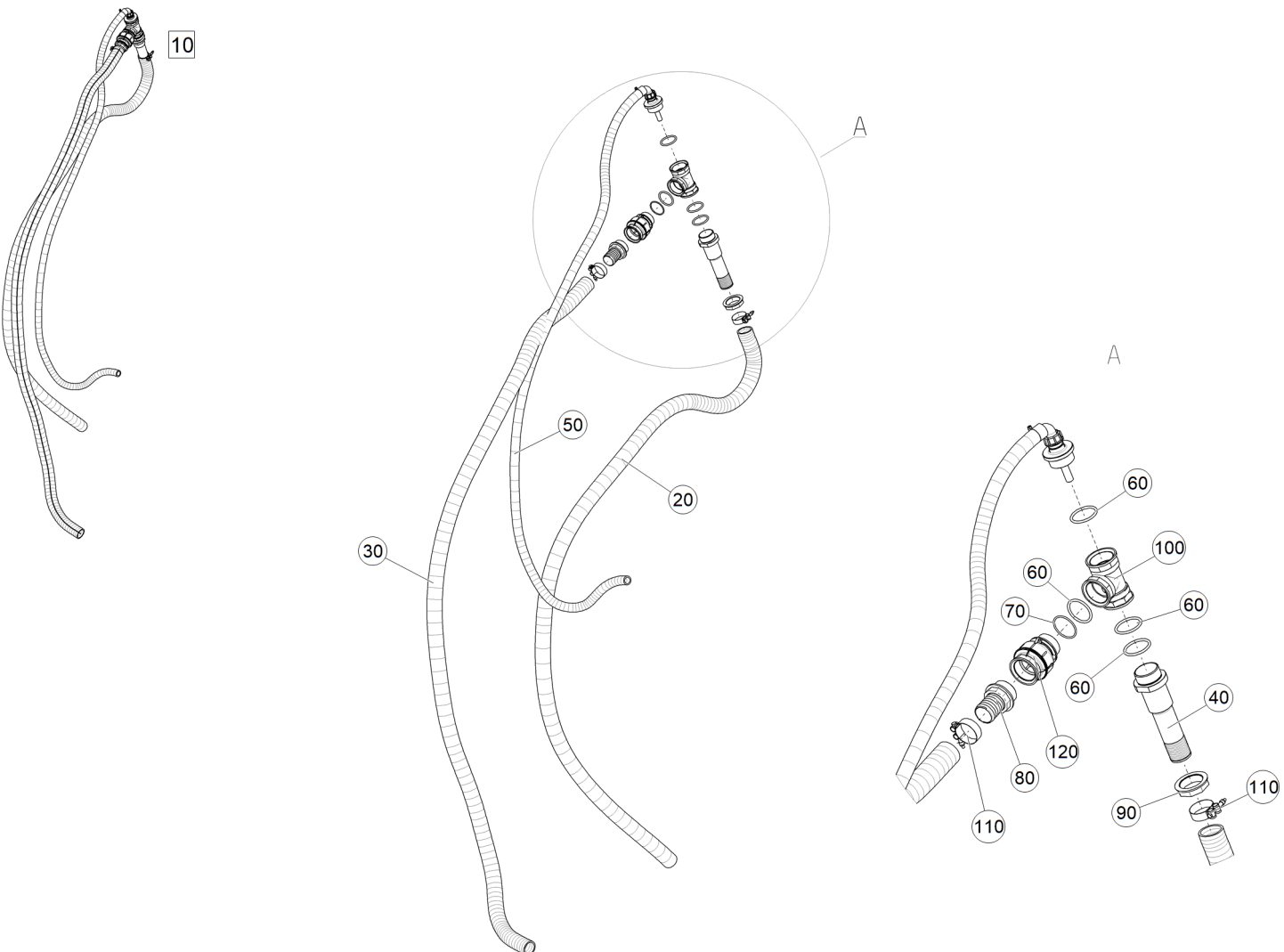
Рис. 1 ЕТВ-60000000325 (Шланг заполнения 2 ZOLL)
