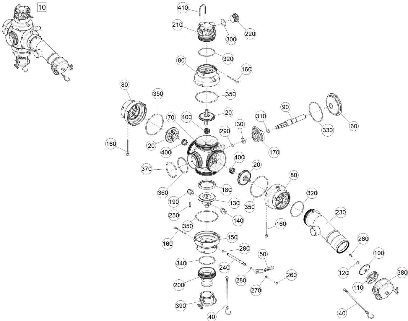
Рис. 1 ЕТВ-6000000319 (Кран всасывающий VORM. UX)
