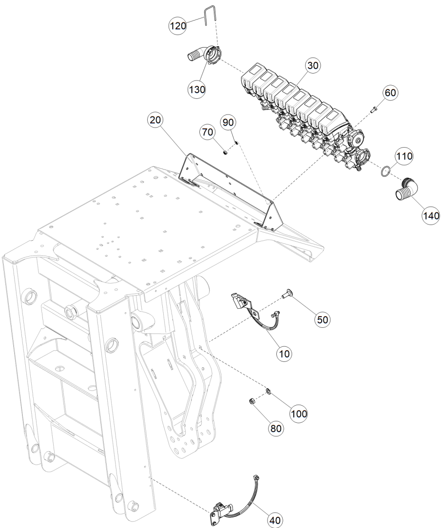
Рис. 1 ЕТВ-6000000278 (Потенциометры и модульный блок)
