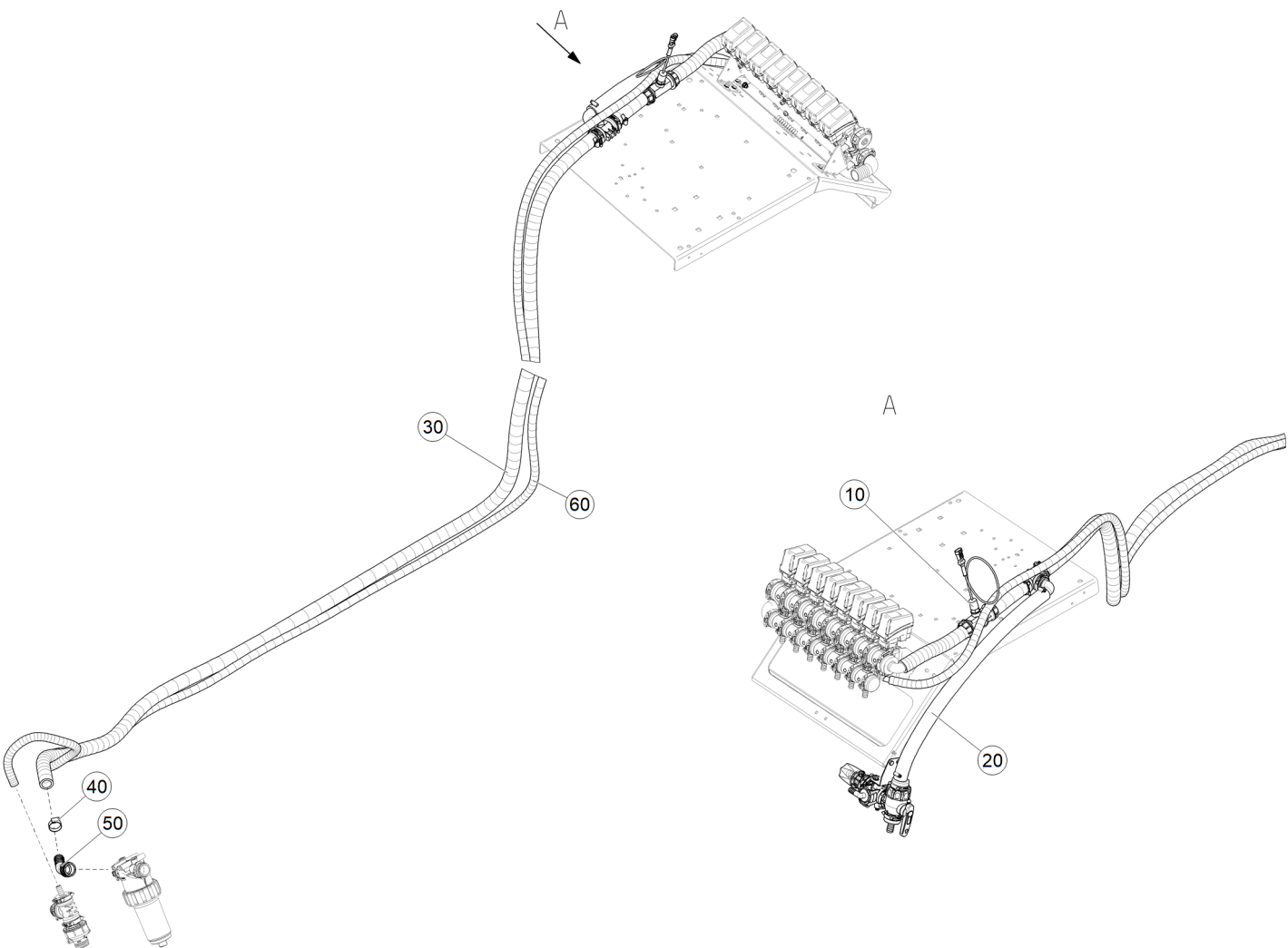
Рис. 1 ЕТВ-6000000269 (Подключение арматуры и клапана напорного)
