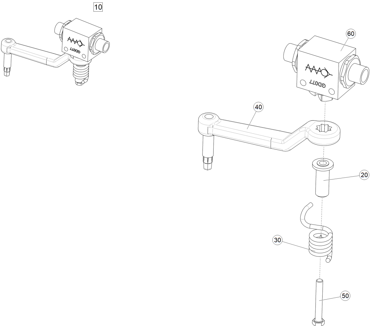
Рис. 1 ЕТВ-60000000380 (Кран гидравлический правый)
