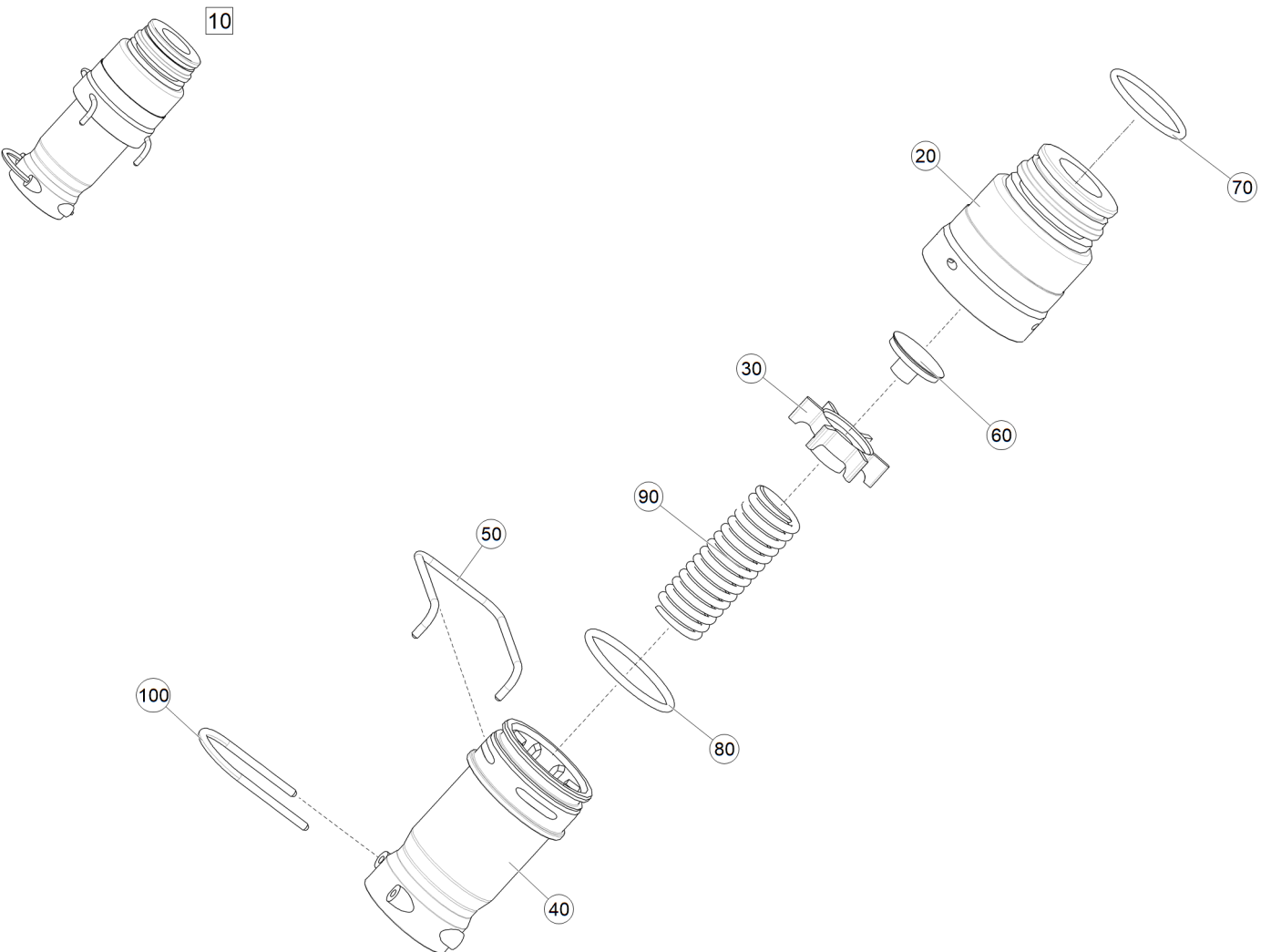
Рис. 1 ЕТВ-6000000316 (Клапан предохранительный NW28 (ROT))
