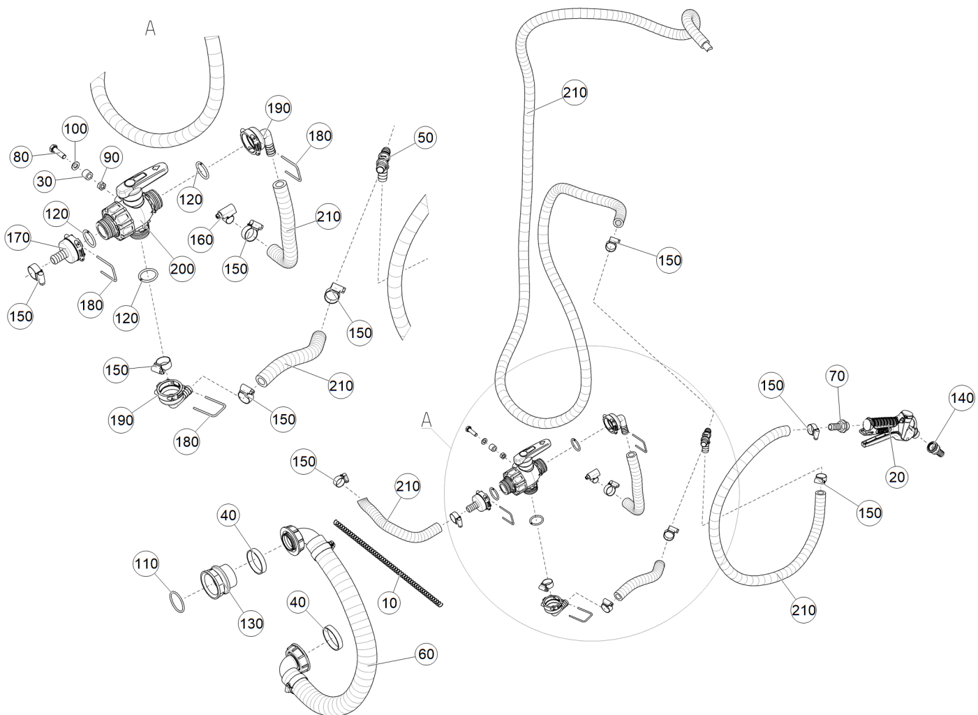
Рис. 1 ЕТВ-6000000274 (Подключения емкости для промывки)
