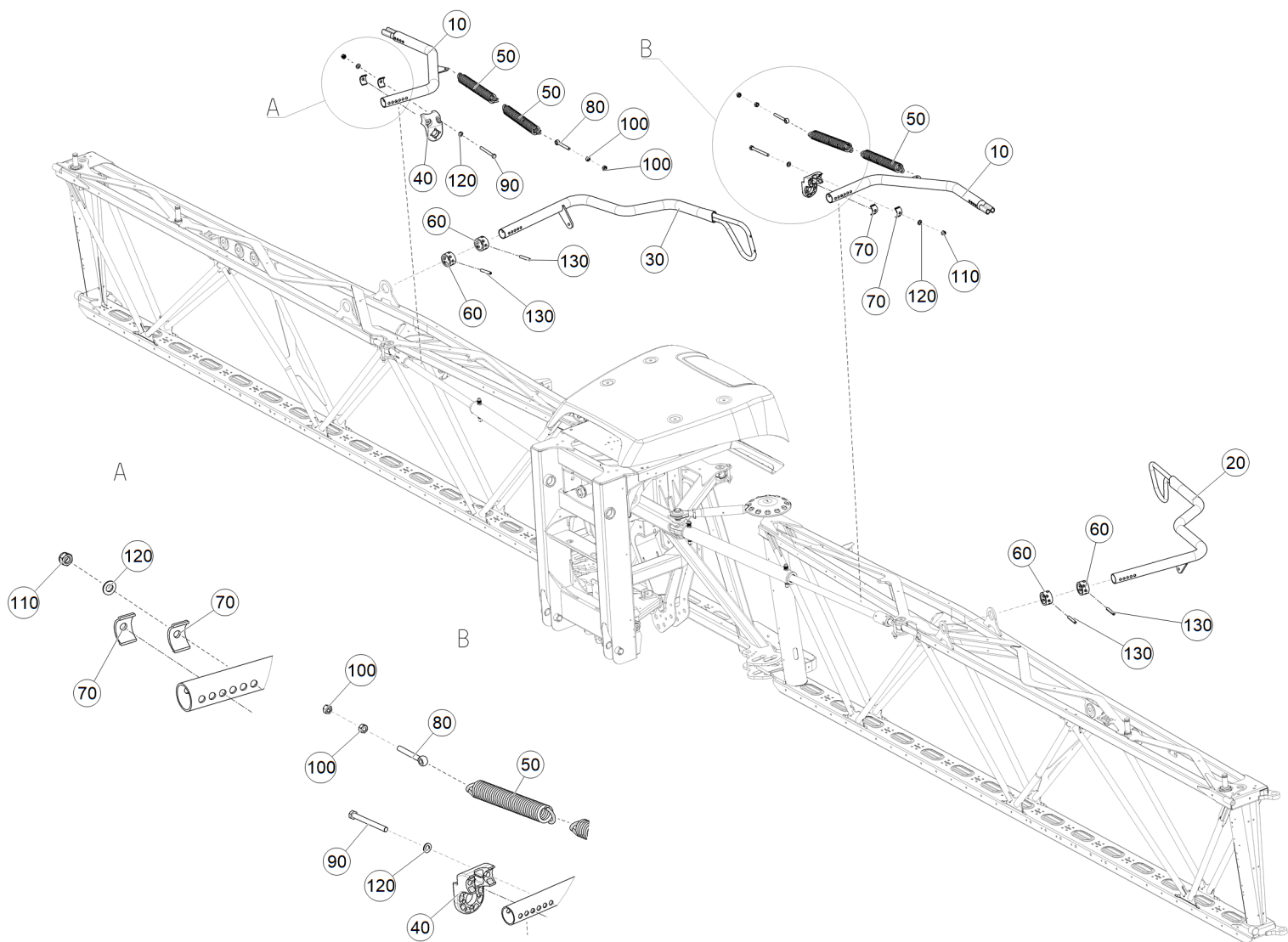
Рис. 1 ETV-6000000288 (Транспортное крепление)
