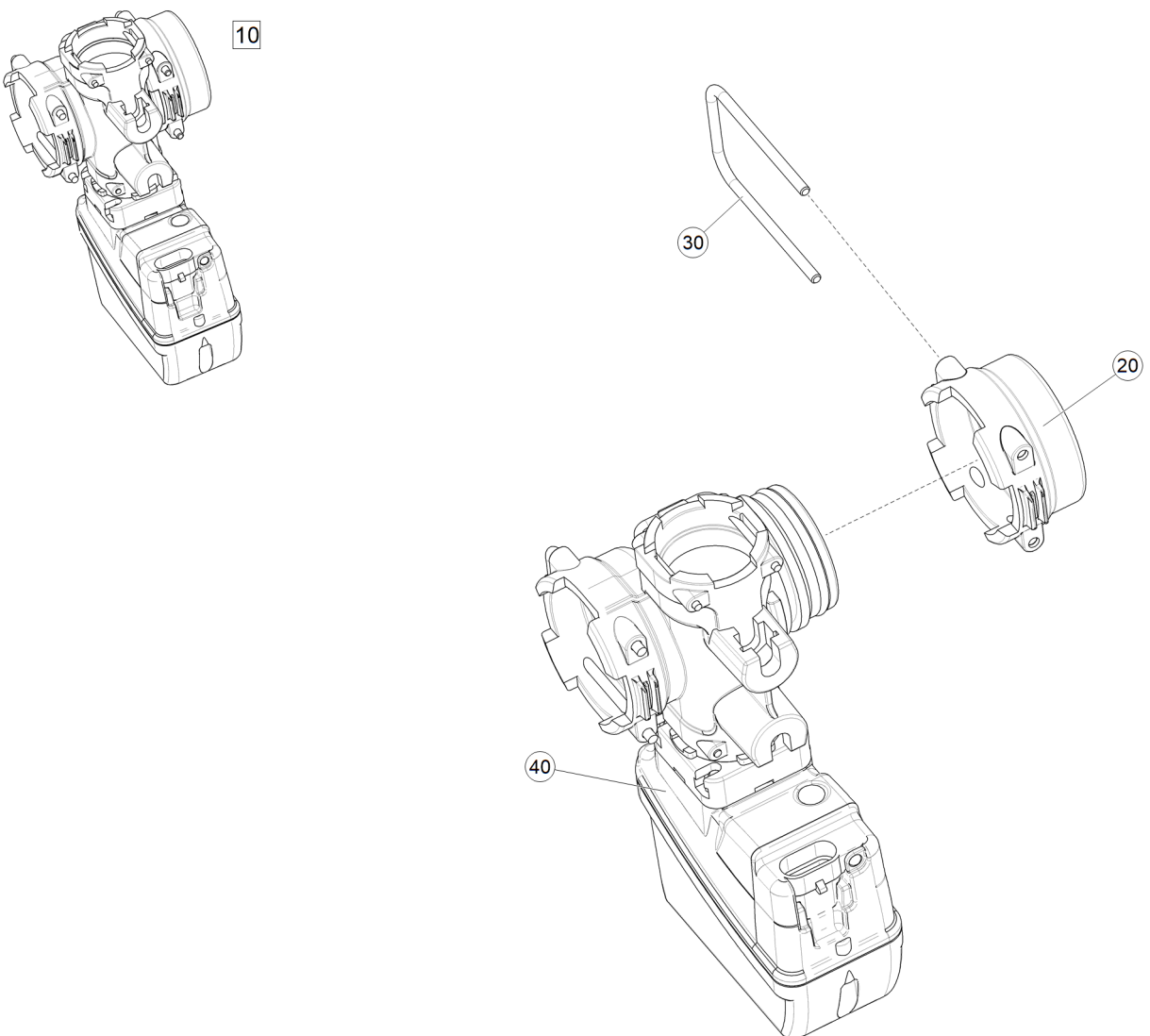
Рис. 1 ЕТВ-6000000303 (Вентиль мотора vormontiert)
