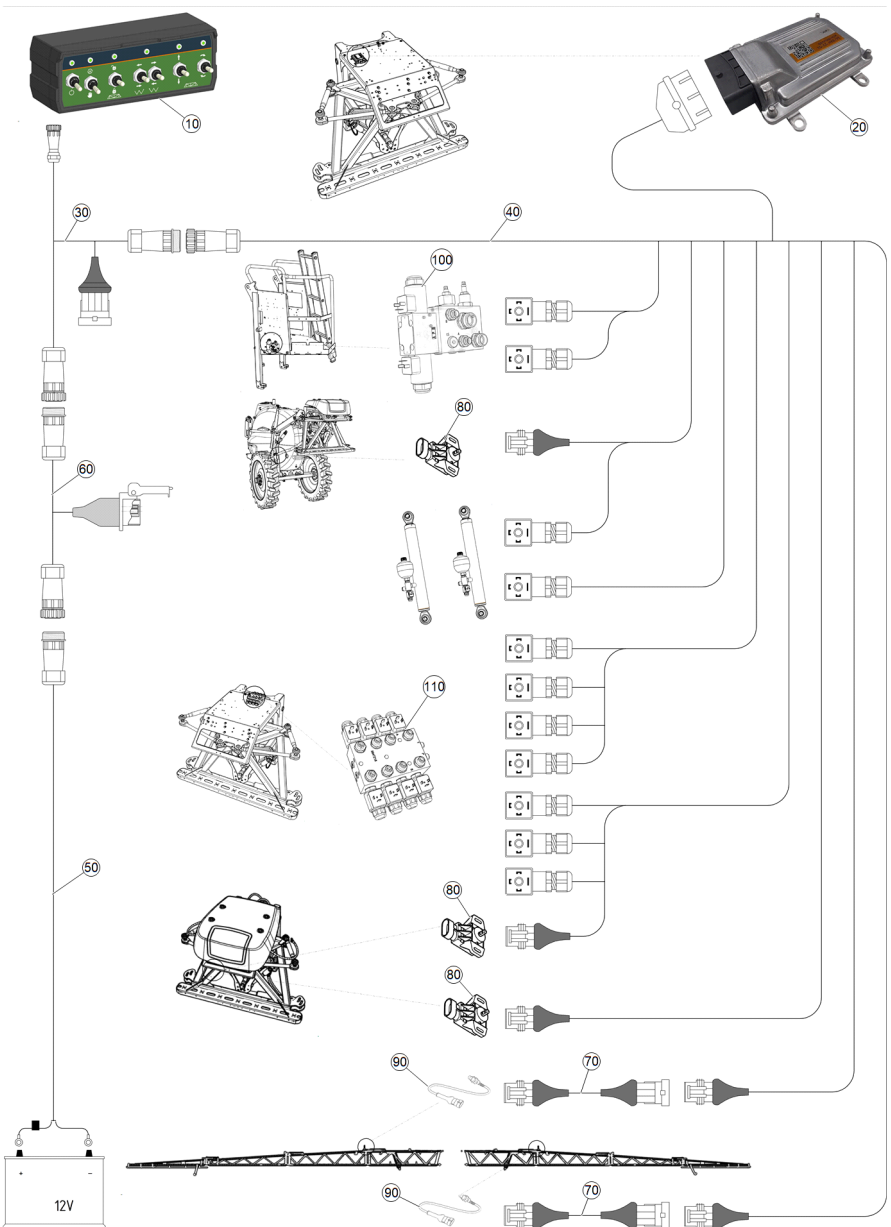
Рис. 1 ETB-6000000168 (Электроника управления гидравликой)
