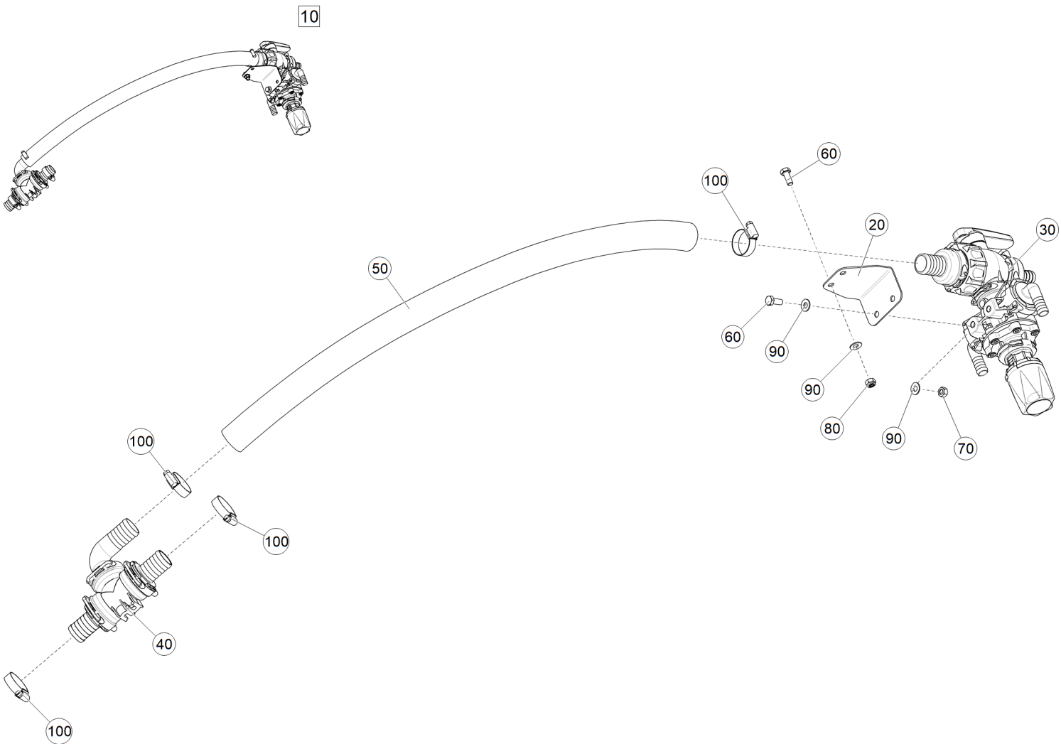
Рис. 1 ETB-6000000335 (Клапан напорный)
