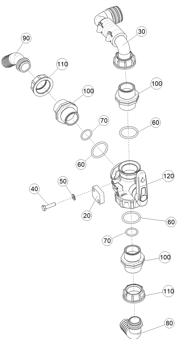
Рис. 1 ЕТВ-6000000305 (Кран VORM. UX)
