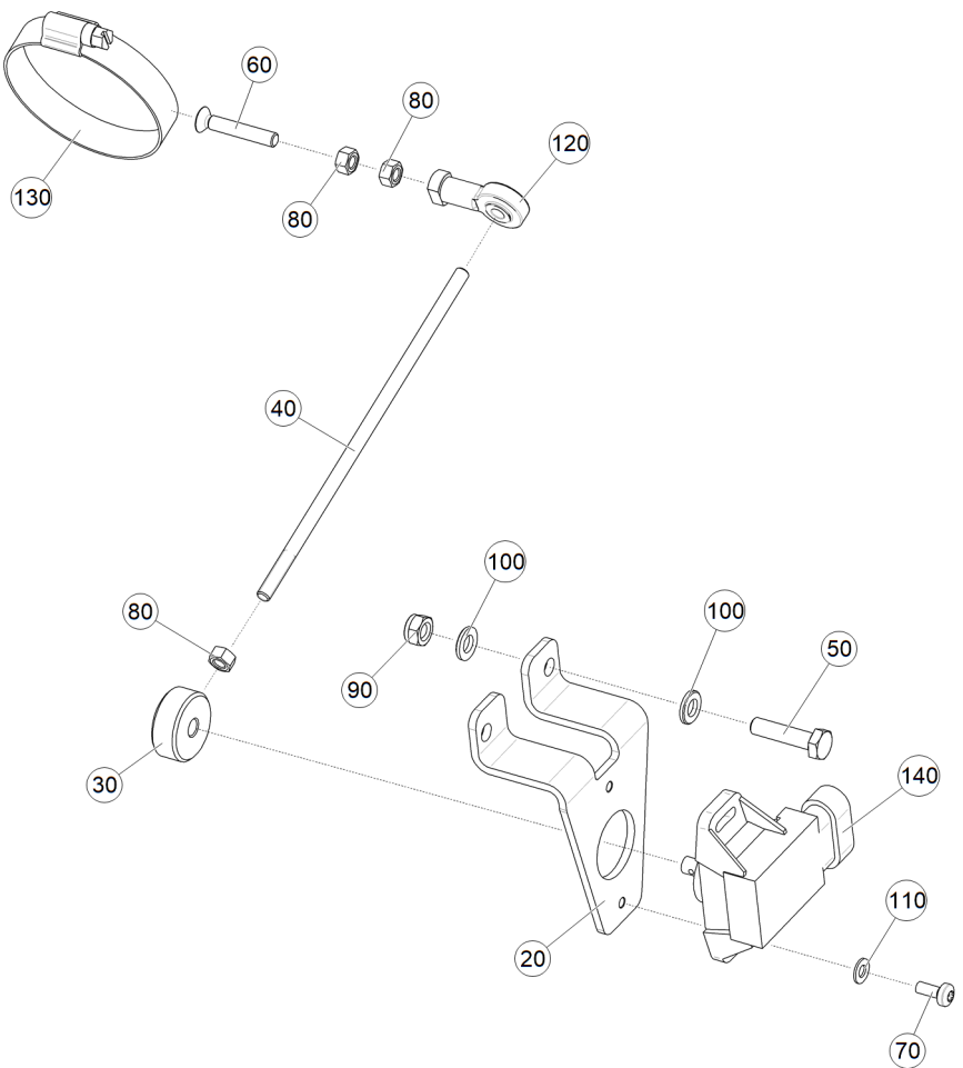
Рис. 1 ЕТВ-6000000295 (Сенсор)
