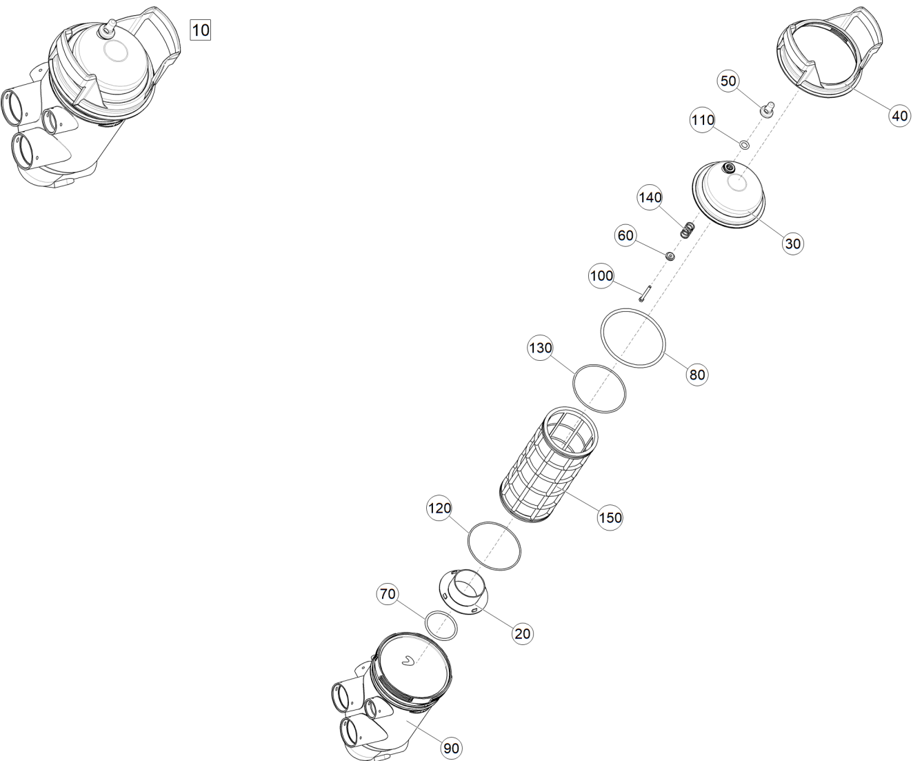
Рис. 1 ЕТВ-6000000334 (Фильтр VORM. UX)
