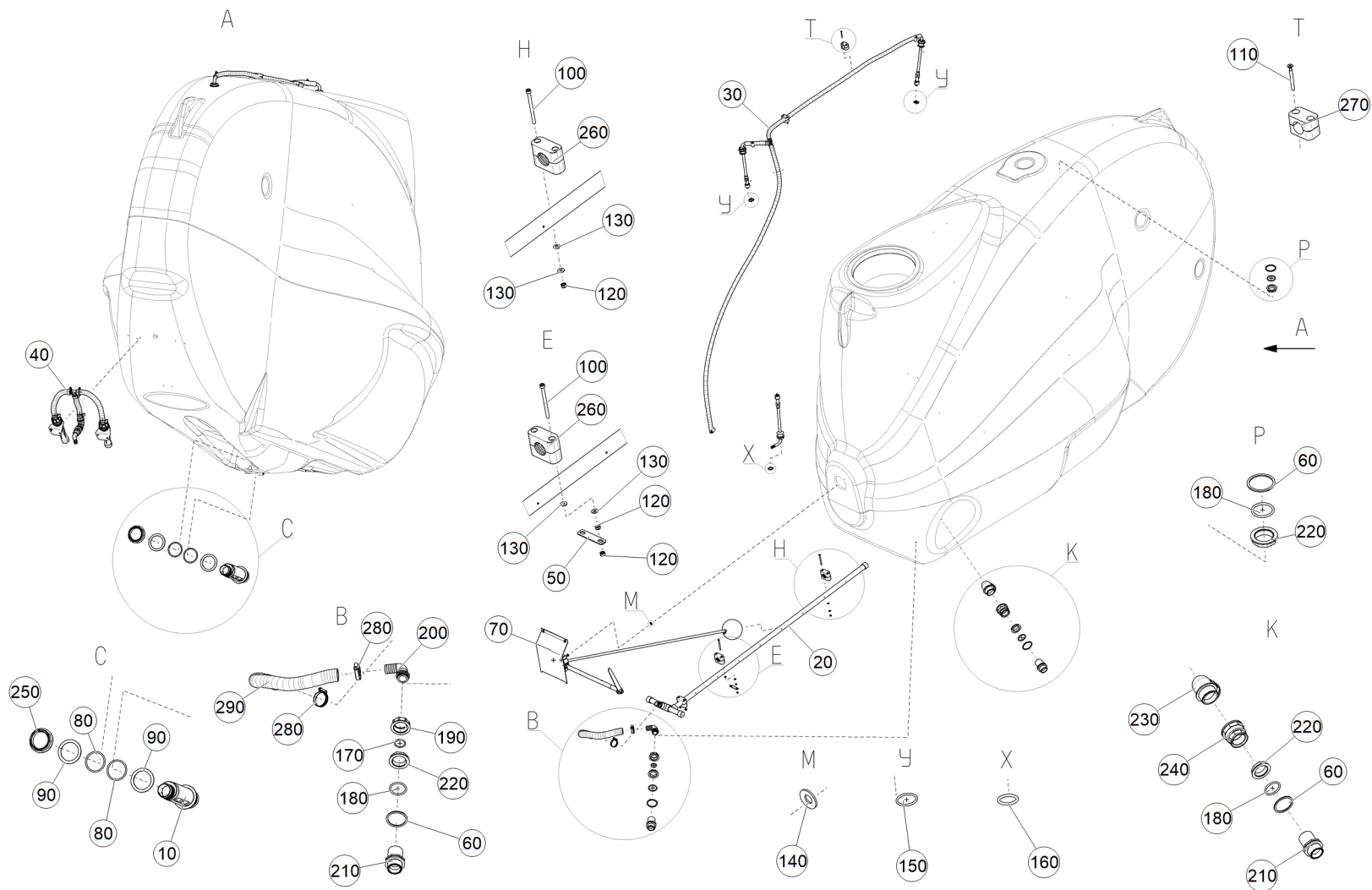
Рис. 1 ЕТВ-6000000336 (Внутренние элементы Емкости UX 5200 SUPER)
