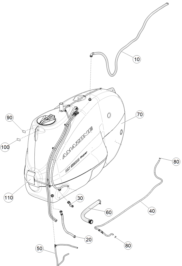
Рис. 1 ЕТВ-6000000271 (Емкость 5200л)
