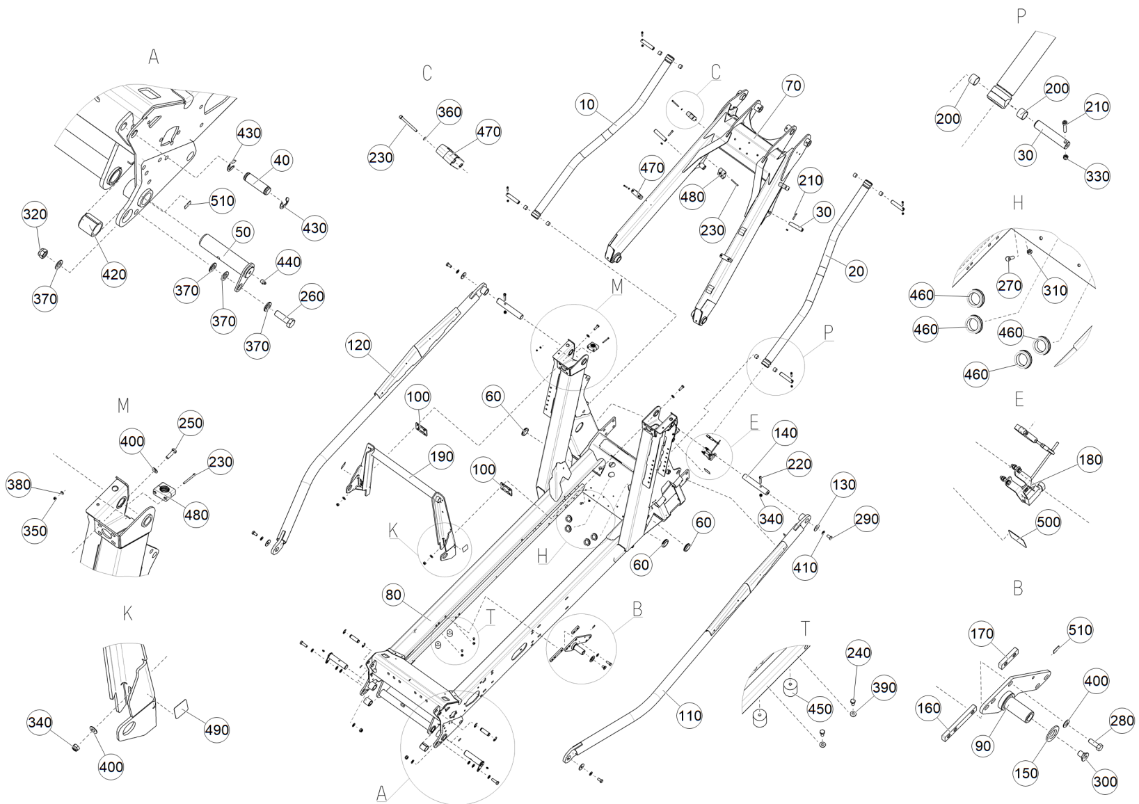
Рис. 1 ЕТВ-6000000258 (Рама с маятником)
