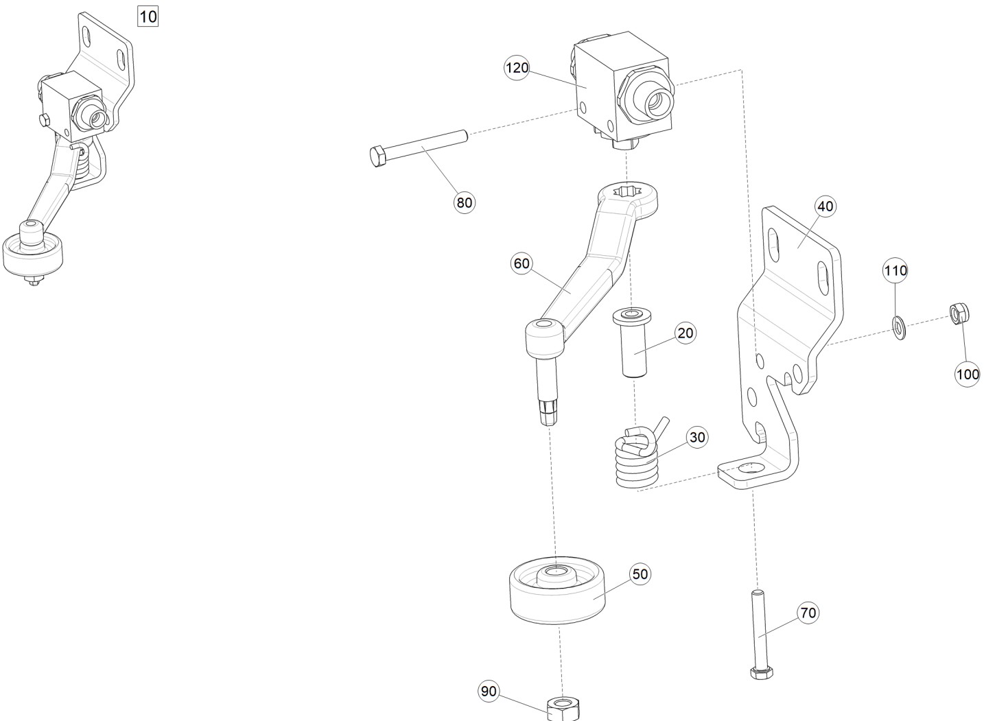
Рис. 1 ЕТВ-6000000378 (Кран гидравлический левый)
