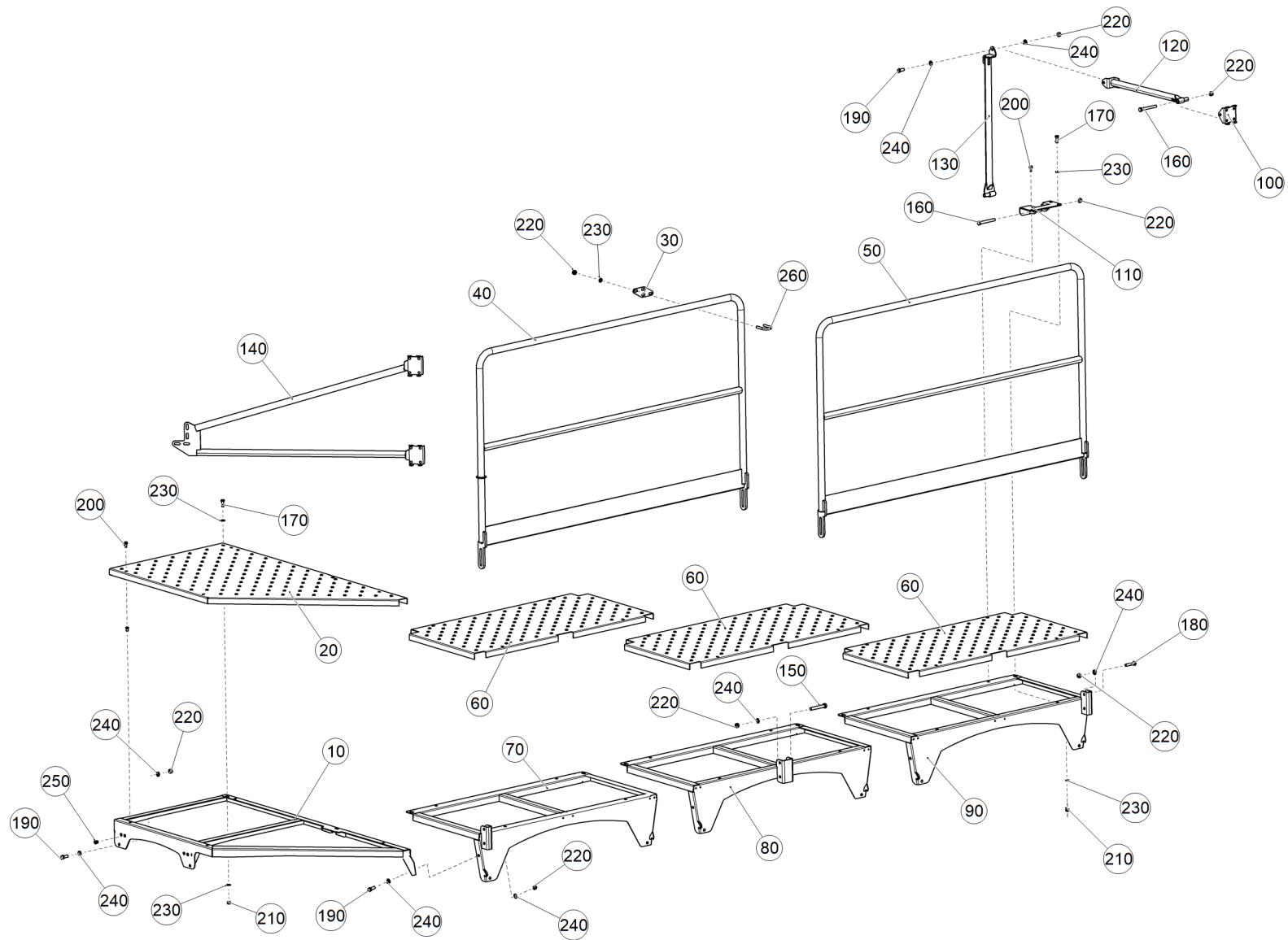
Рис. 1 ЕТВ-6000000028 (Площадка)
