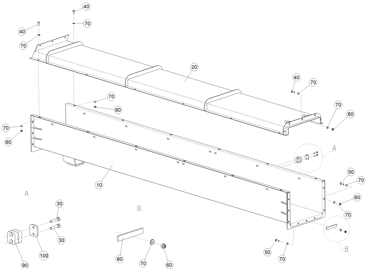
Рис. 1 ЕТВ-6000000190 (Секция нижняя)
