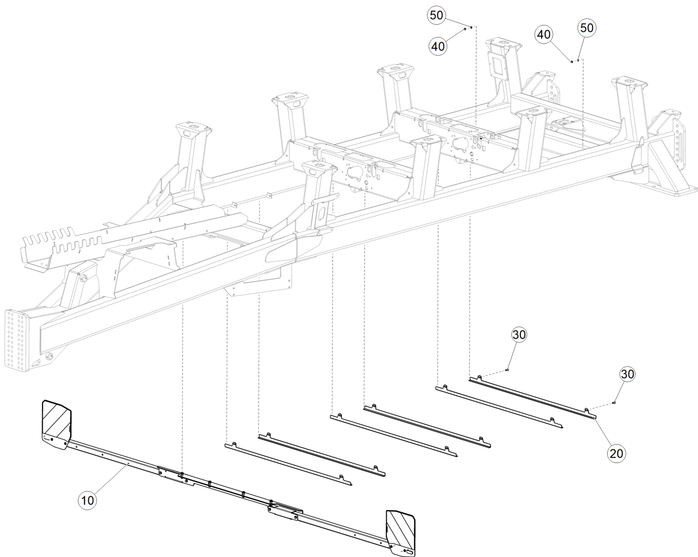
Рис. 1 ЕТВ-6000000018 (Направляющие лотка, комплект передних световозвратателей)
