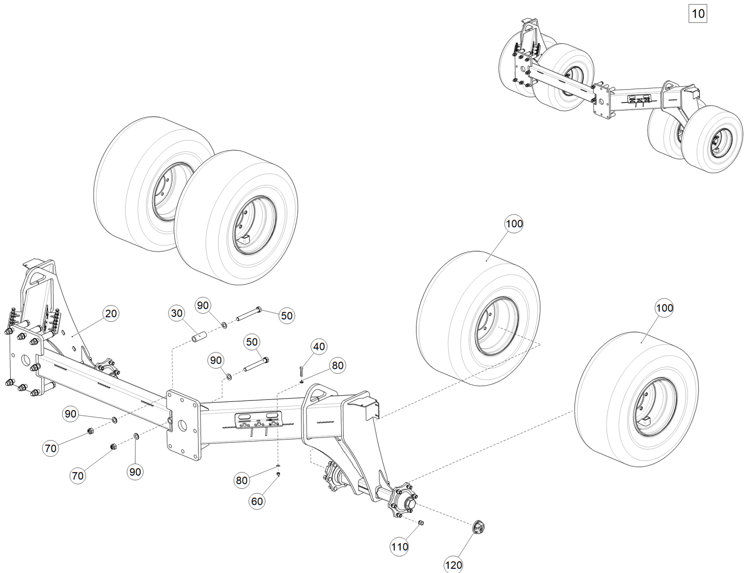
Рис. 1 ЕТВ-6000000085 (Рамa колесная задняя в сборе)
