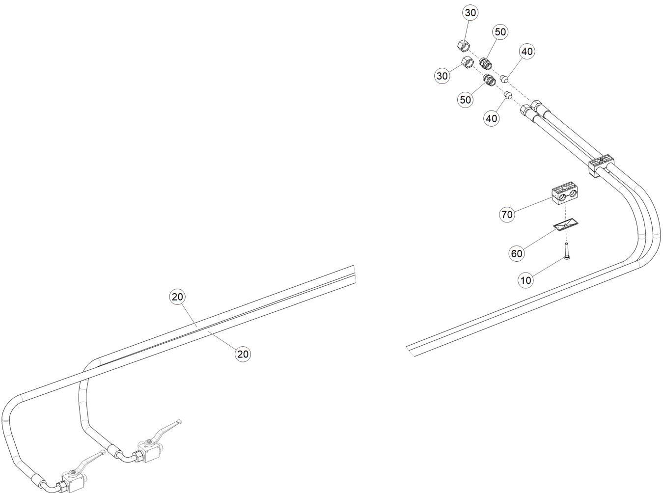
Рис. 1 ЕТВ-6000000124 (Линия загрузочного устройства)
