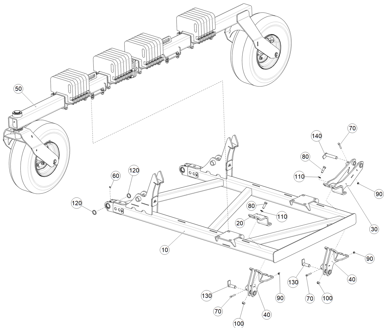
Рис. 1 ЕТВ-6000000063 (Рама левая)
