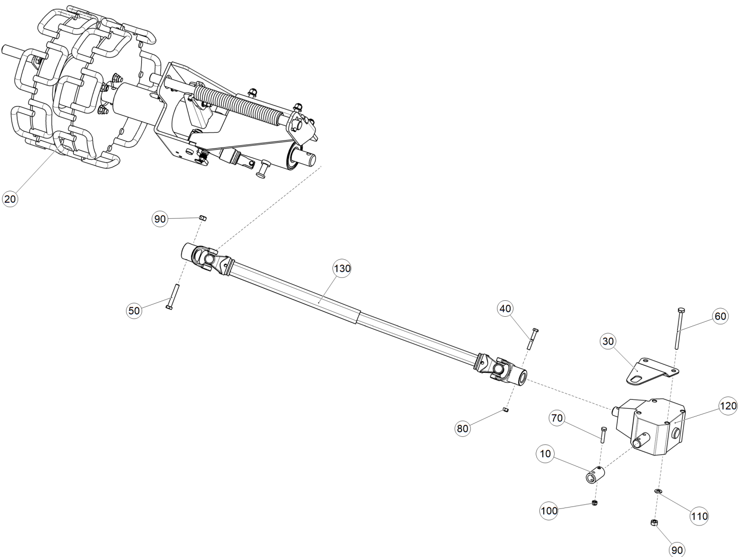
Рис. 1 ЕТВ-60000000033 (Привод колеса, кардан, редуктор)
