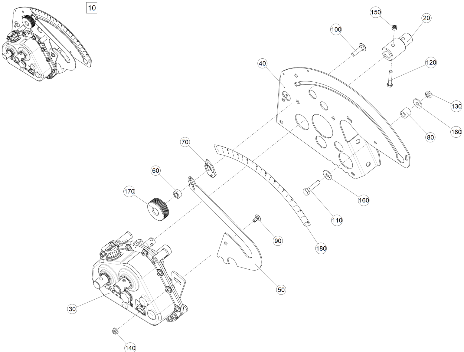
Рис. 1 ETB-6000000060 (Вариоредуктор DSC левый)
