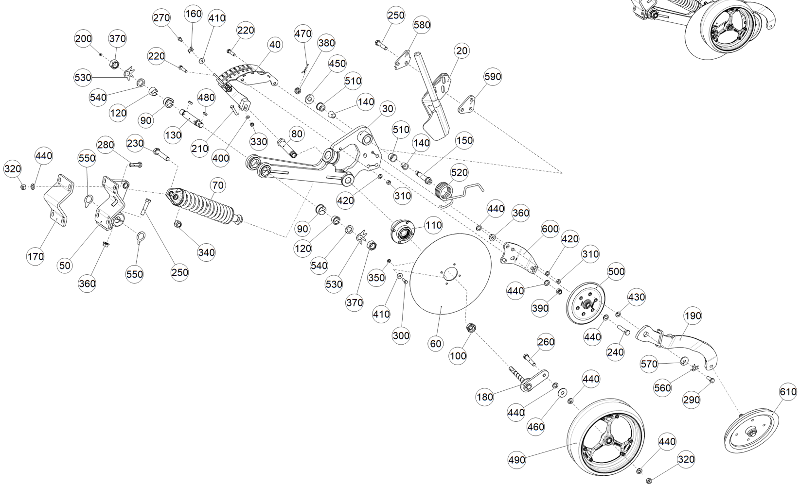
Рис. 1 ETB-6000000091 (Сошник левый DSC)
