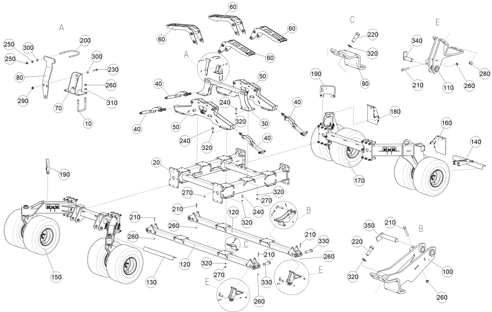
Рис. 1 ЕТВ-6000000064 (Рама центральная)
