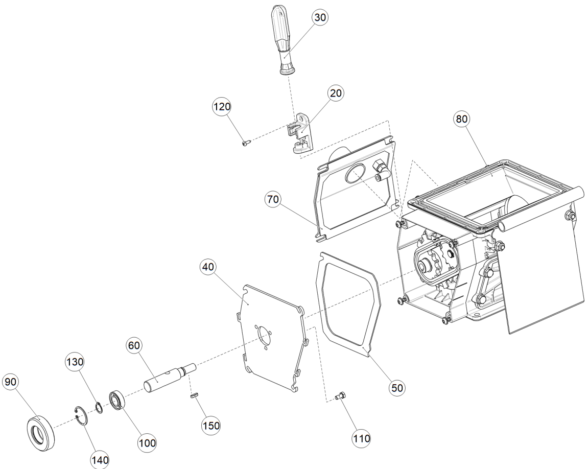
Рис. 1 ЕТВ-6000000052 (Дозатор DSC левый)
