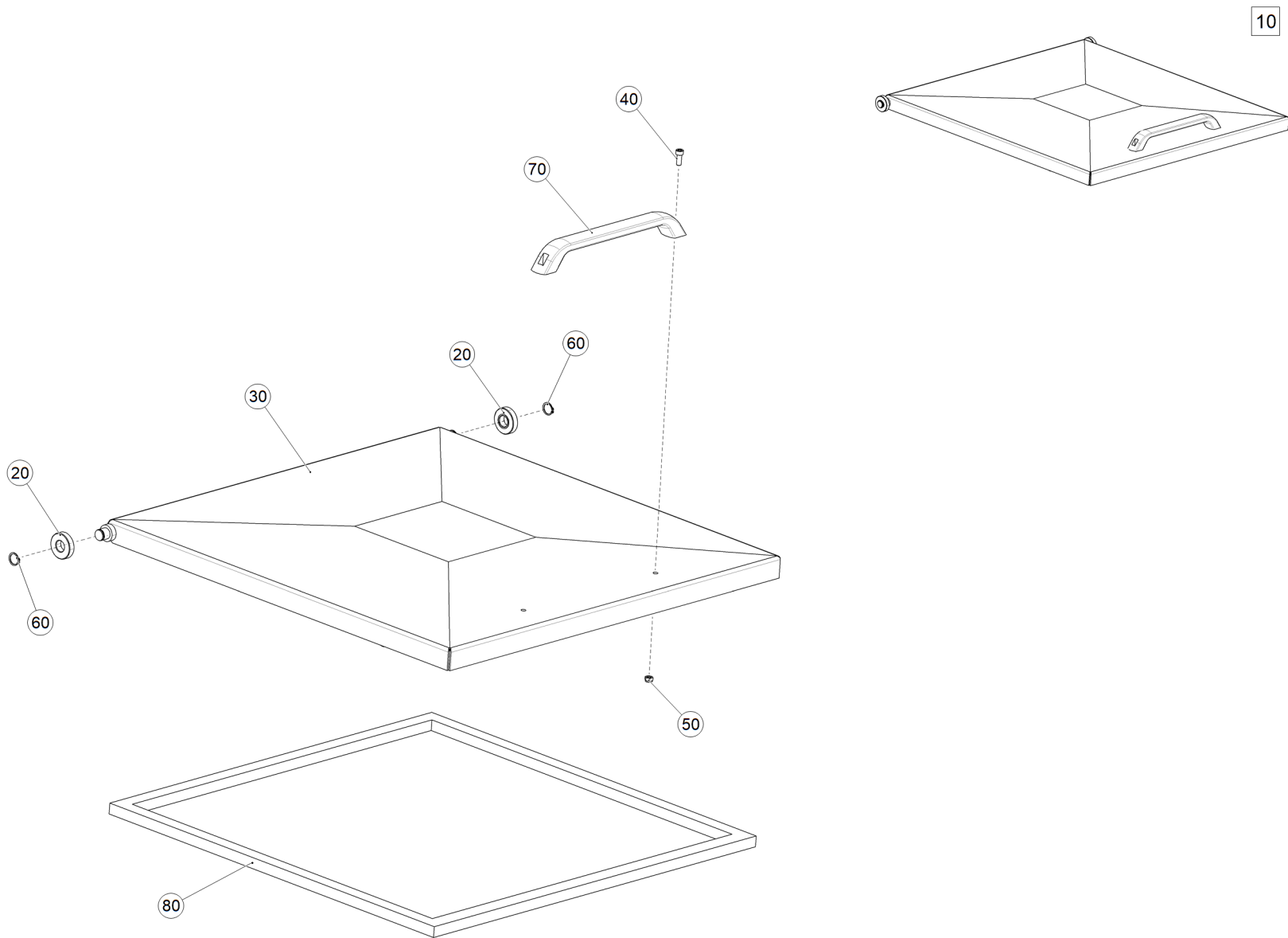
Рис. 1 ЕТВ-6000000037 (Люк)
