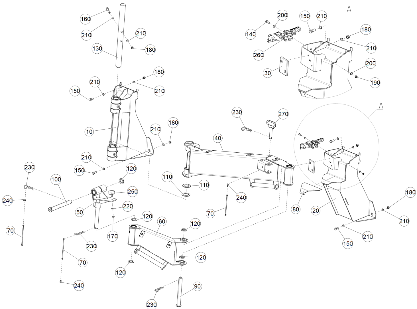
Рис. 1 ЕТВ-6000000198 (Опоры и кронштейны центральные)
