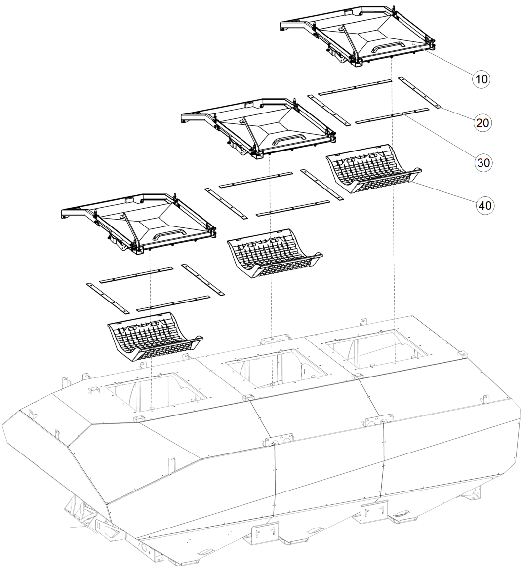
Рис. 1 ЕТВ-6000000021 (Крышка и корзина)
