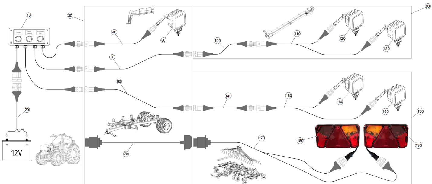
Рис. 1 ЕТВ-6000000172 (Освещение рабочее Discara)
