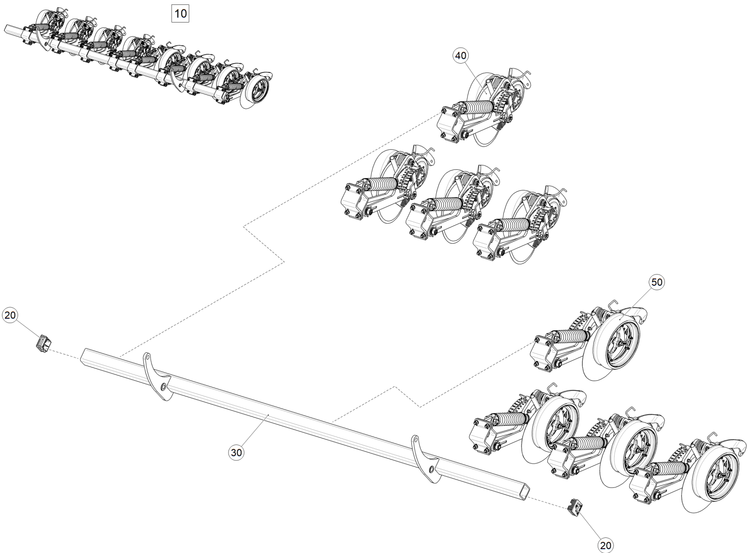
Рис. 1 ЕТВ-6000000100 (Балка сошниковая задняя центральная)
