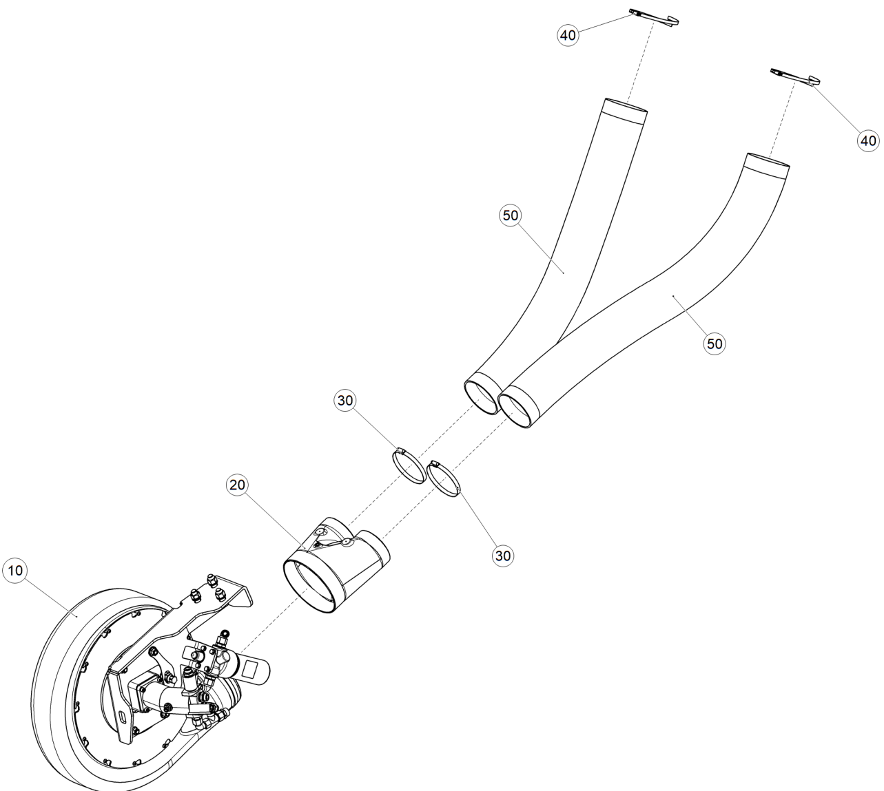
Рис. 1 ЕТВ-6000000030 (Вентилятор)
