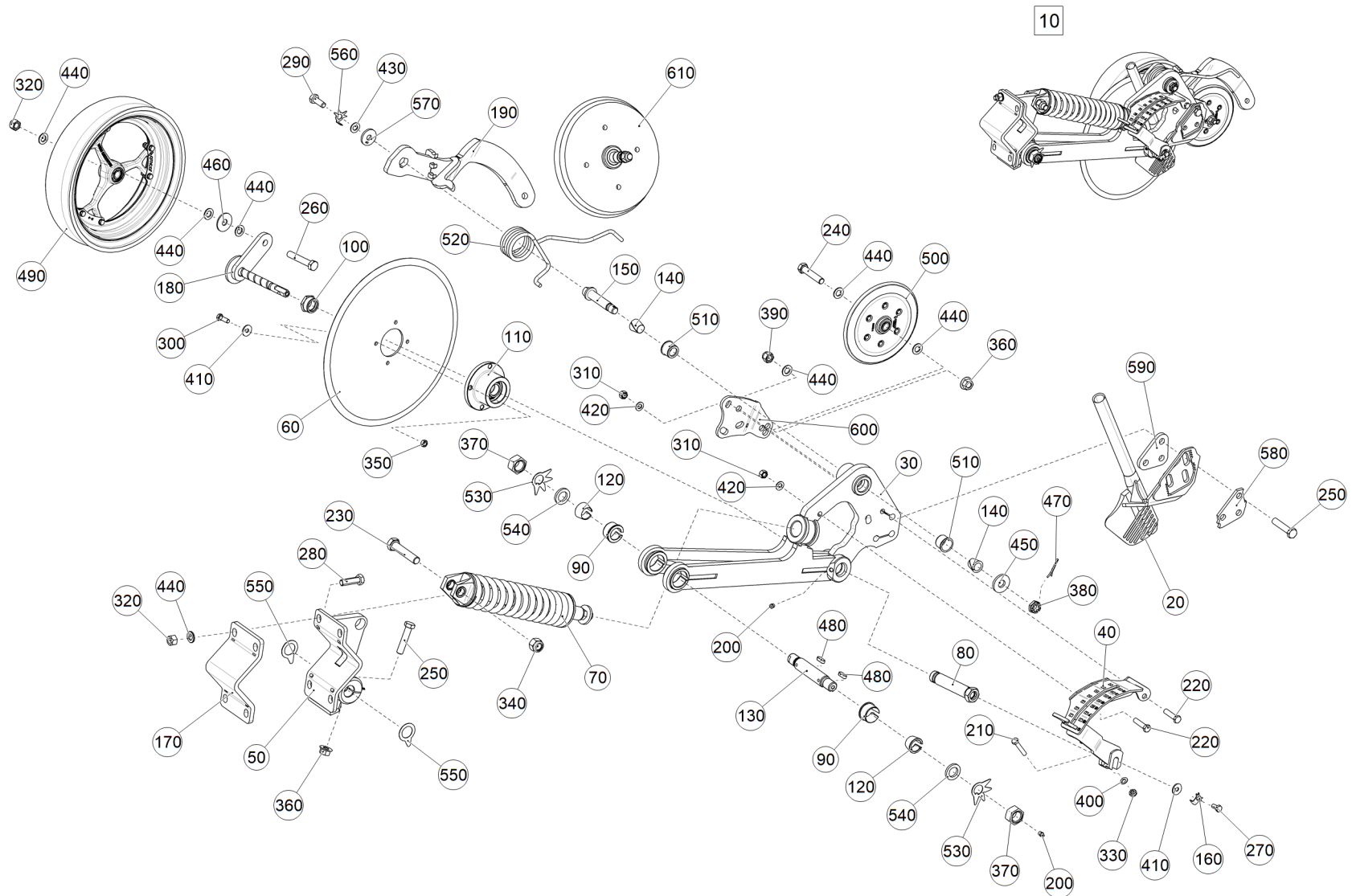
Рис. 1 ЕТВ-6000000097 (Сошник правый DSC)
