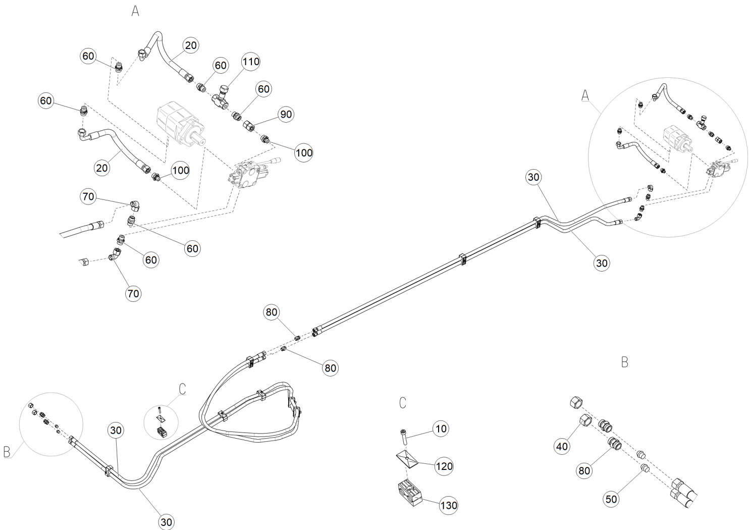
Рис. 1 ЕТВ-6000000223 (Гидрооборудование устройства загрузочного)
