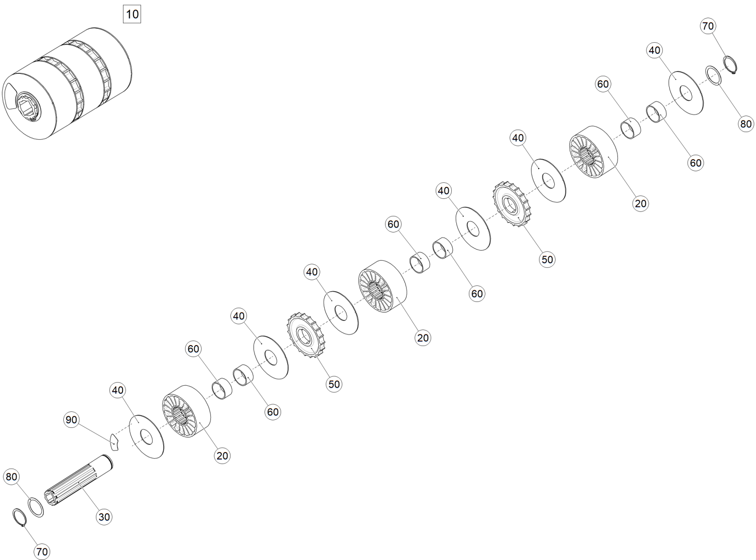
Рис. 1 ЕТВ-6000000109 (Катушка высевающая 20 см)
