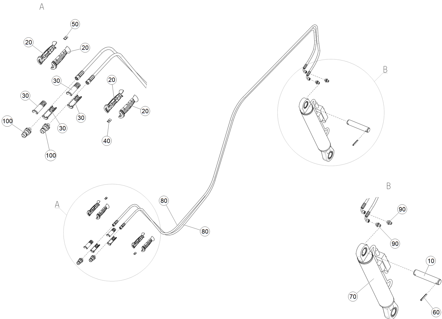
Рис. 1 ЕТВ-6000000119 (Линия опорной ноги DSC)
