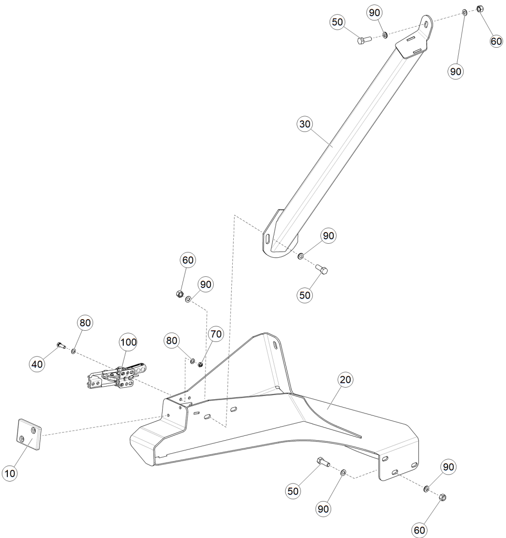
Рис. 1 ETB-6000000197 (Опоры и кронштейны нижние)
