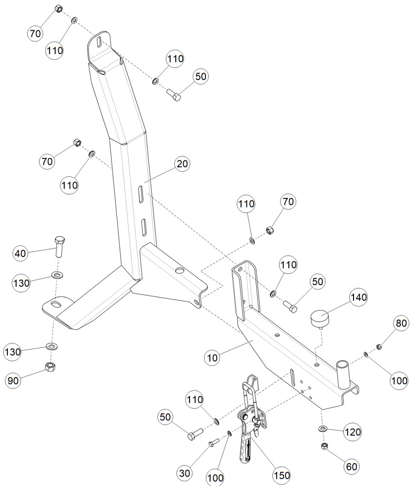
Рис. 1 ЕТВ-6000000199 (Опоры и кронштейны верхние)
