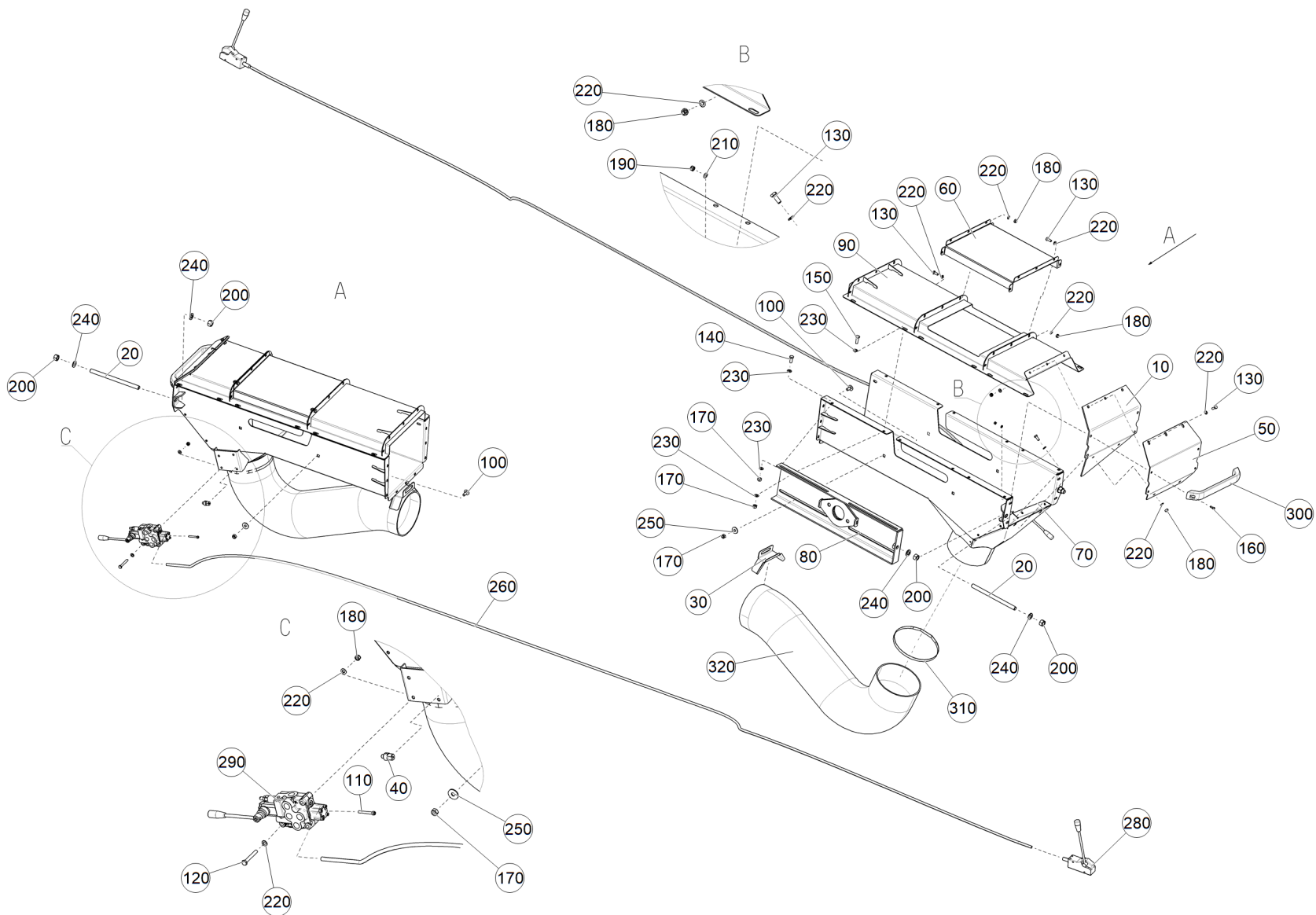
Рис. 1 ЕТВ-6000000194 (Оголовок)
