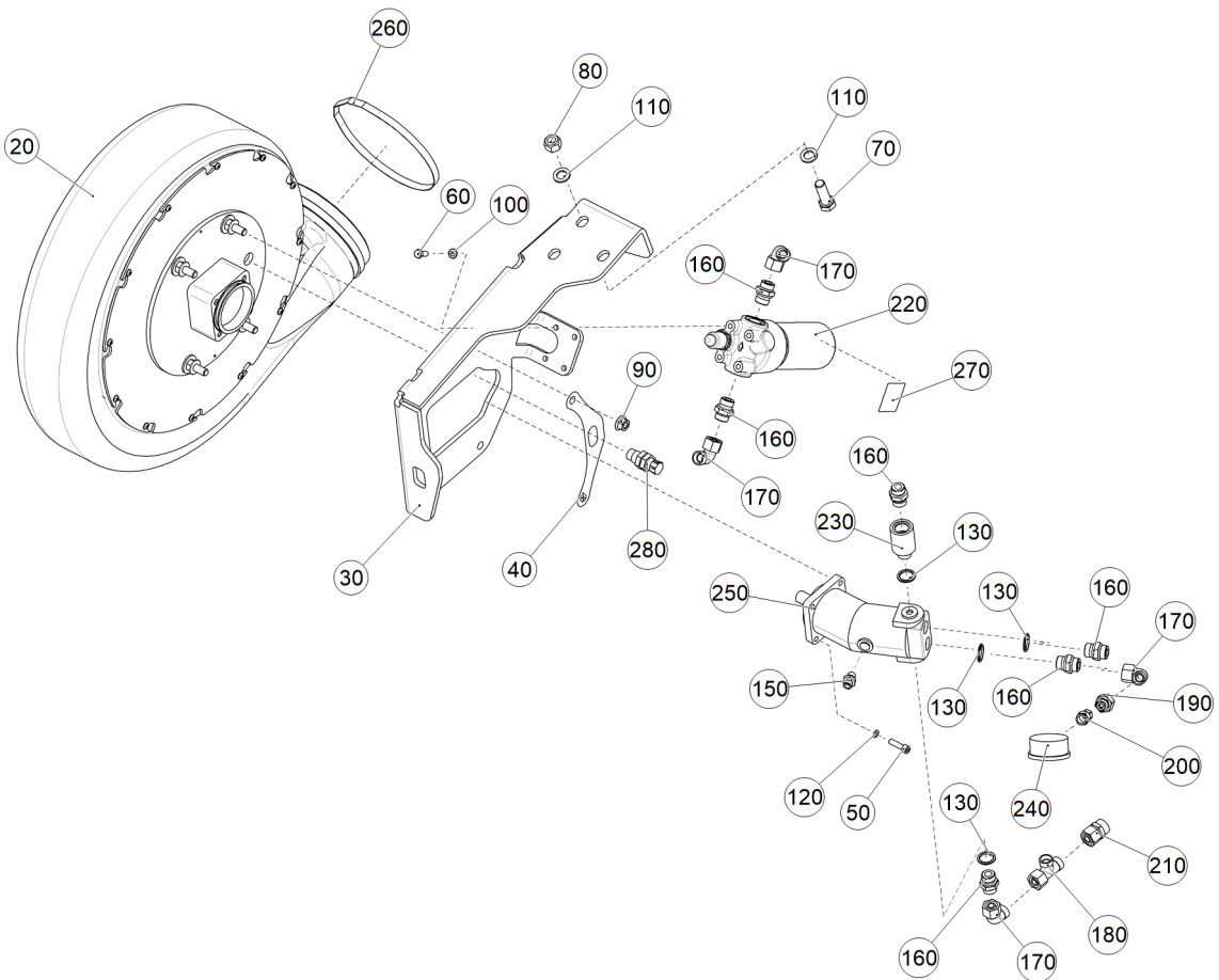
Рис. 1 ЕТВ-6000000043 (Вентилятор Discara правый)
