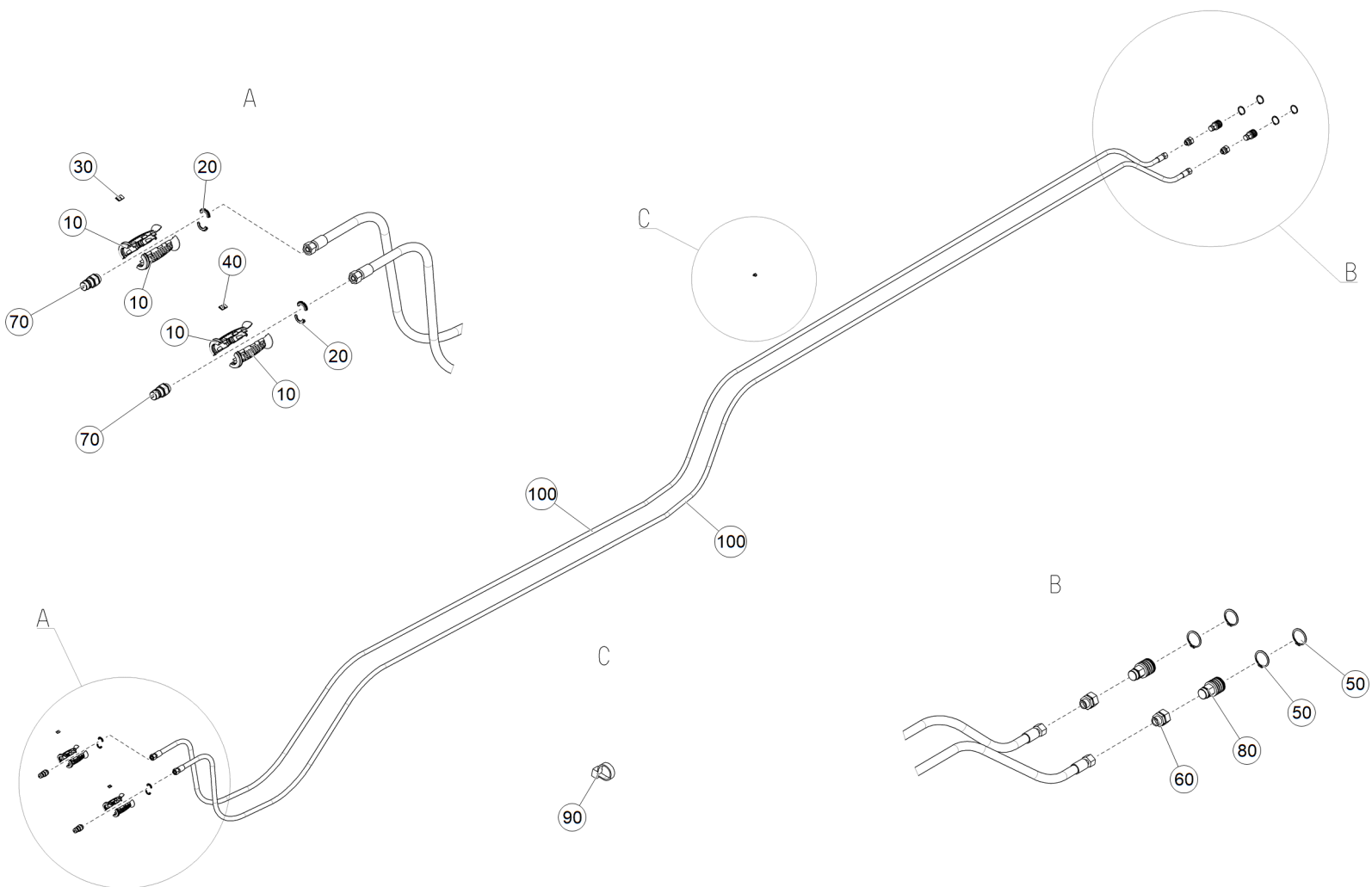
Рис. 1 ЕТВ-6000000121 (Линия крыльев DSC)
