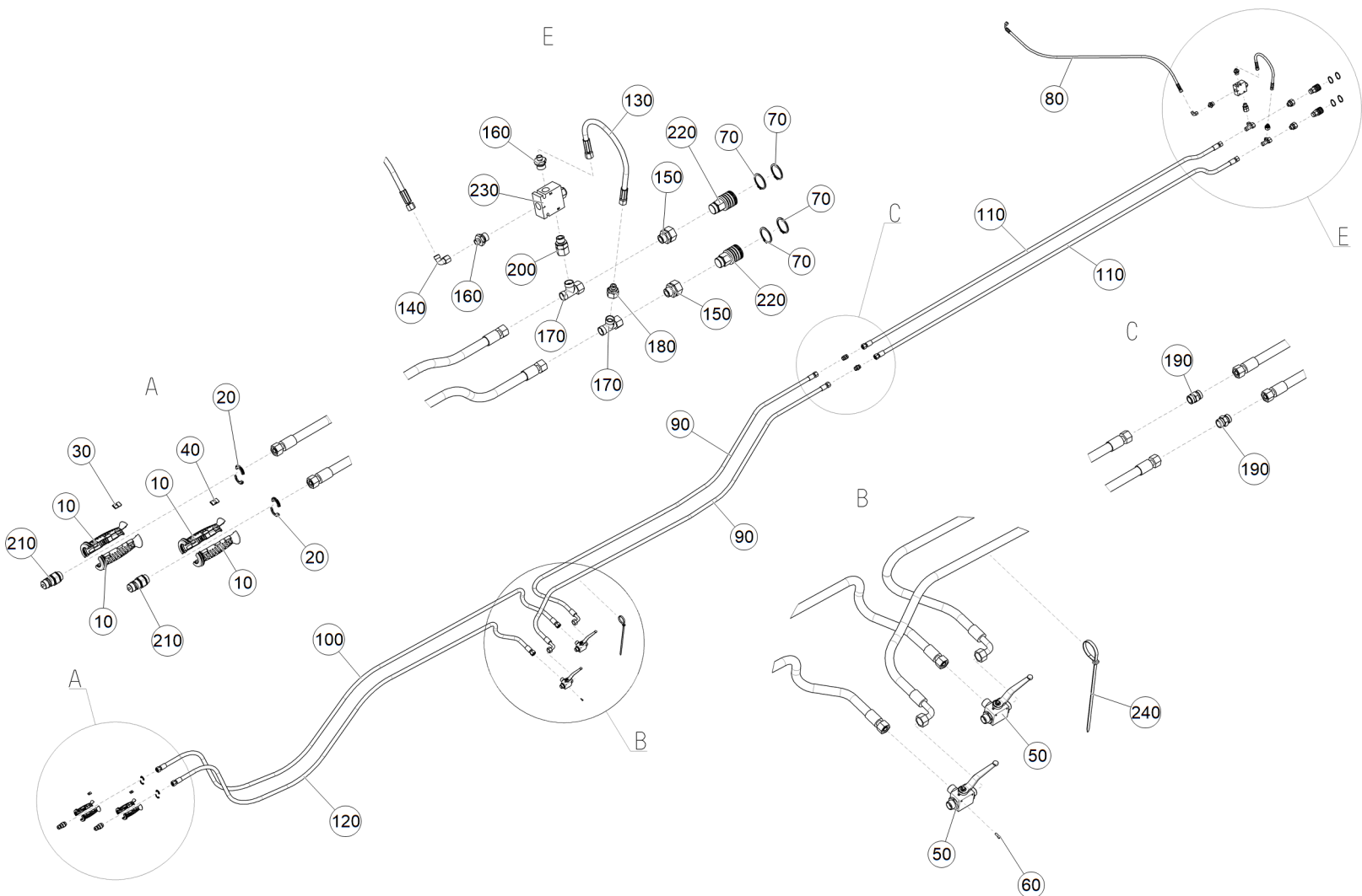
Рис. 1 ЕТВ-6000000123 (Линия сошников DSC)
