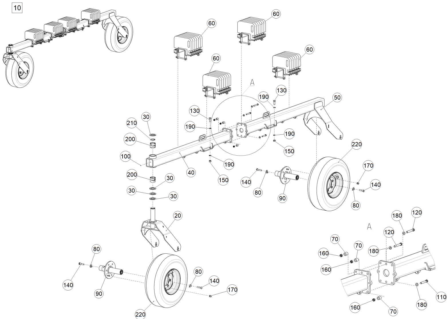
Рис. 1 ЕТВ-6000000074 (Балка продольная в сборе с грузами)
