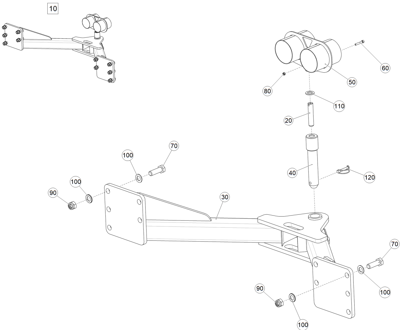
Рис. 1 ETB-6000000087 (Сцепное устройство DSC)
