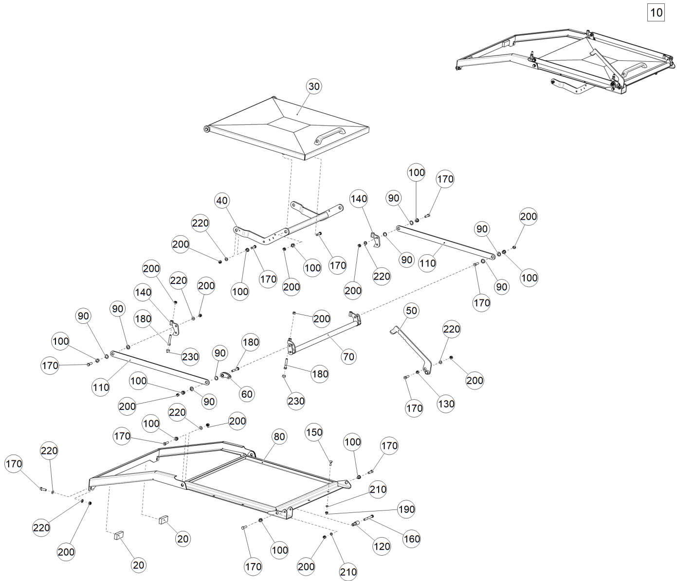
Рис. 1 ЕТВ-6000000036 (Крышка бункера)
