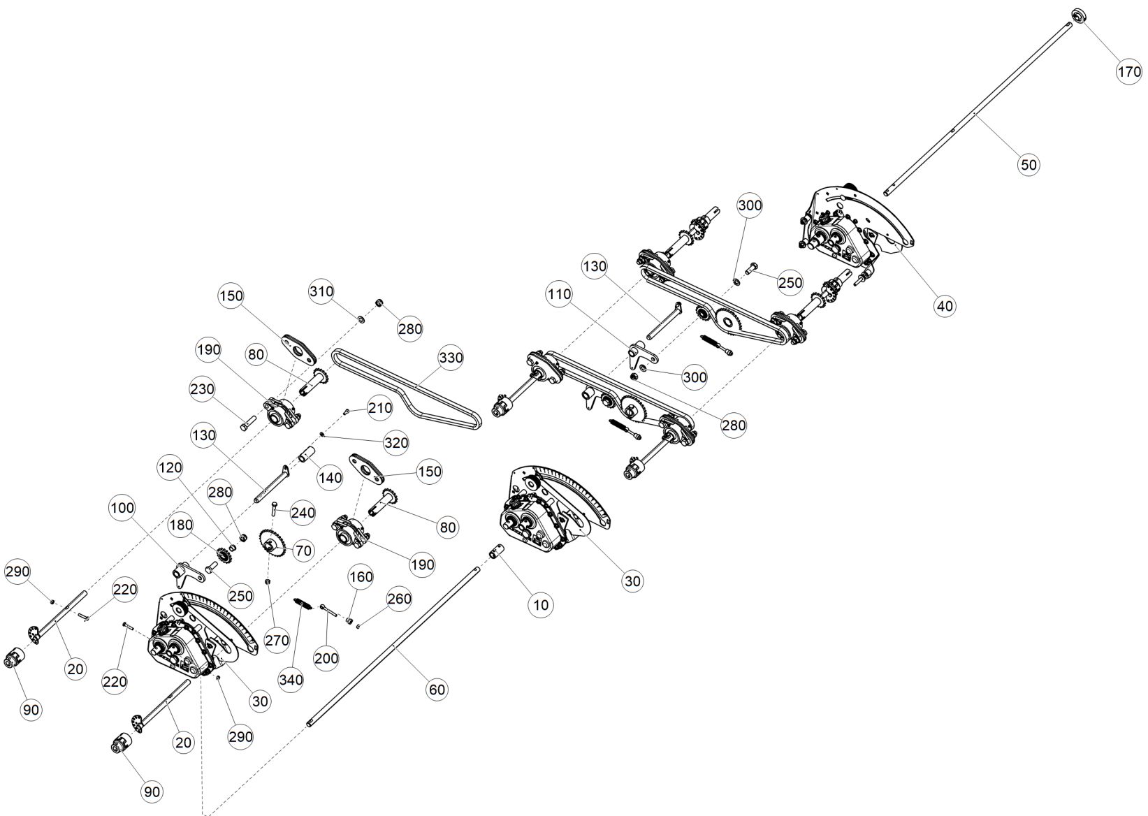
Рис. 1 ЕТВ-6000000034 (Вариоредукторы, приводы)
