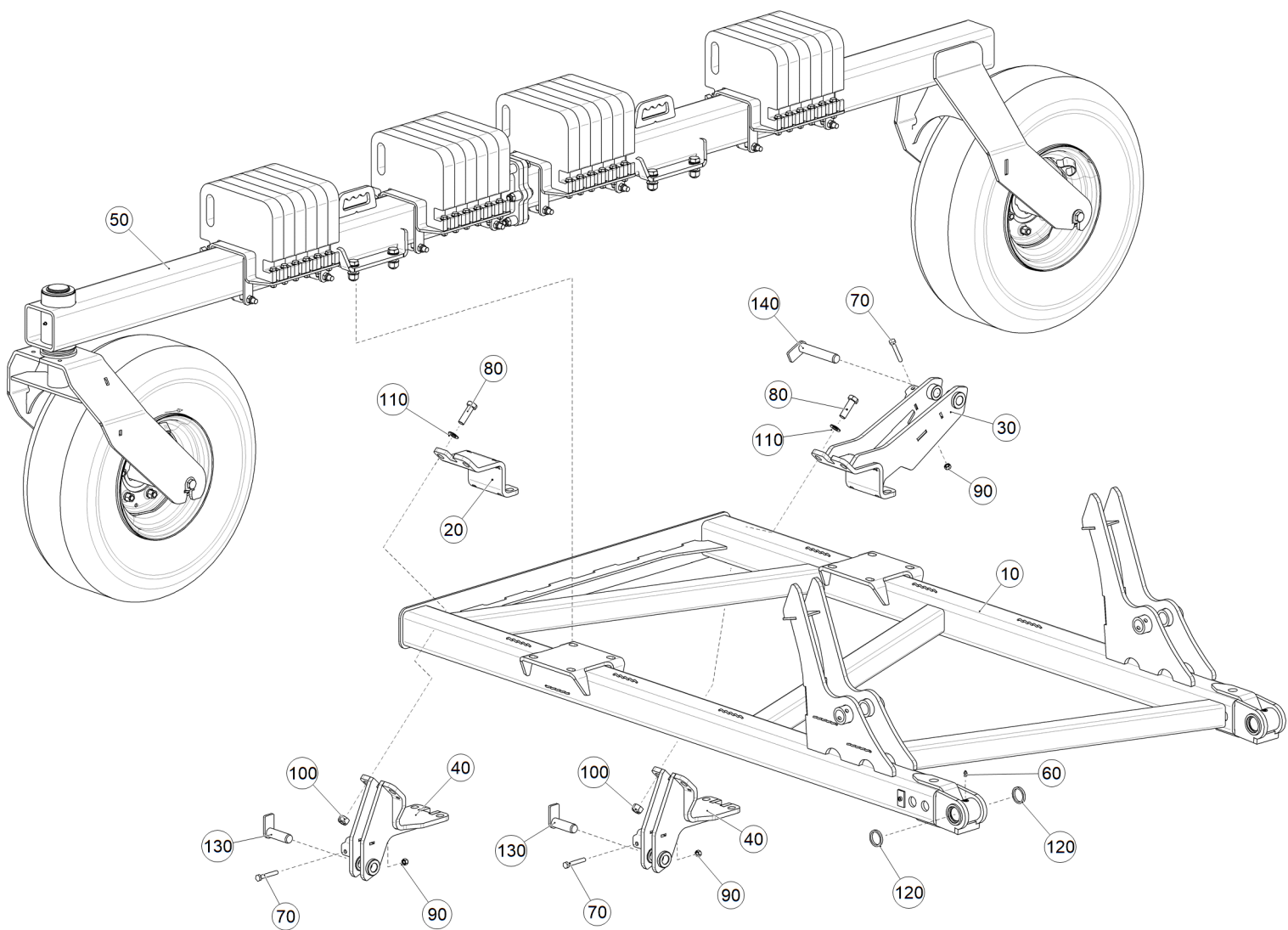
Рис. 1 ETB-6000000065 (Рама правая)
