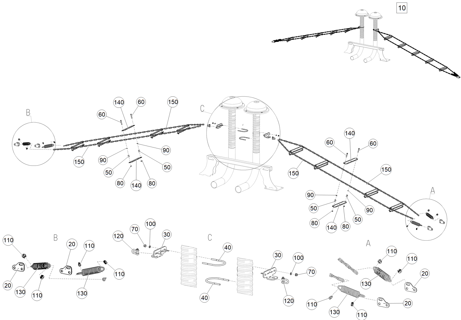
Рис. 1 ETB-6000000108 (Комплект цепей семяпроводов DSC9)
