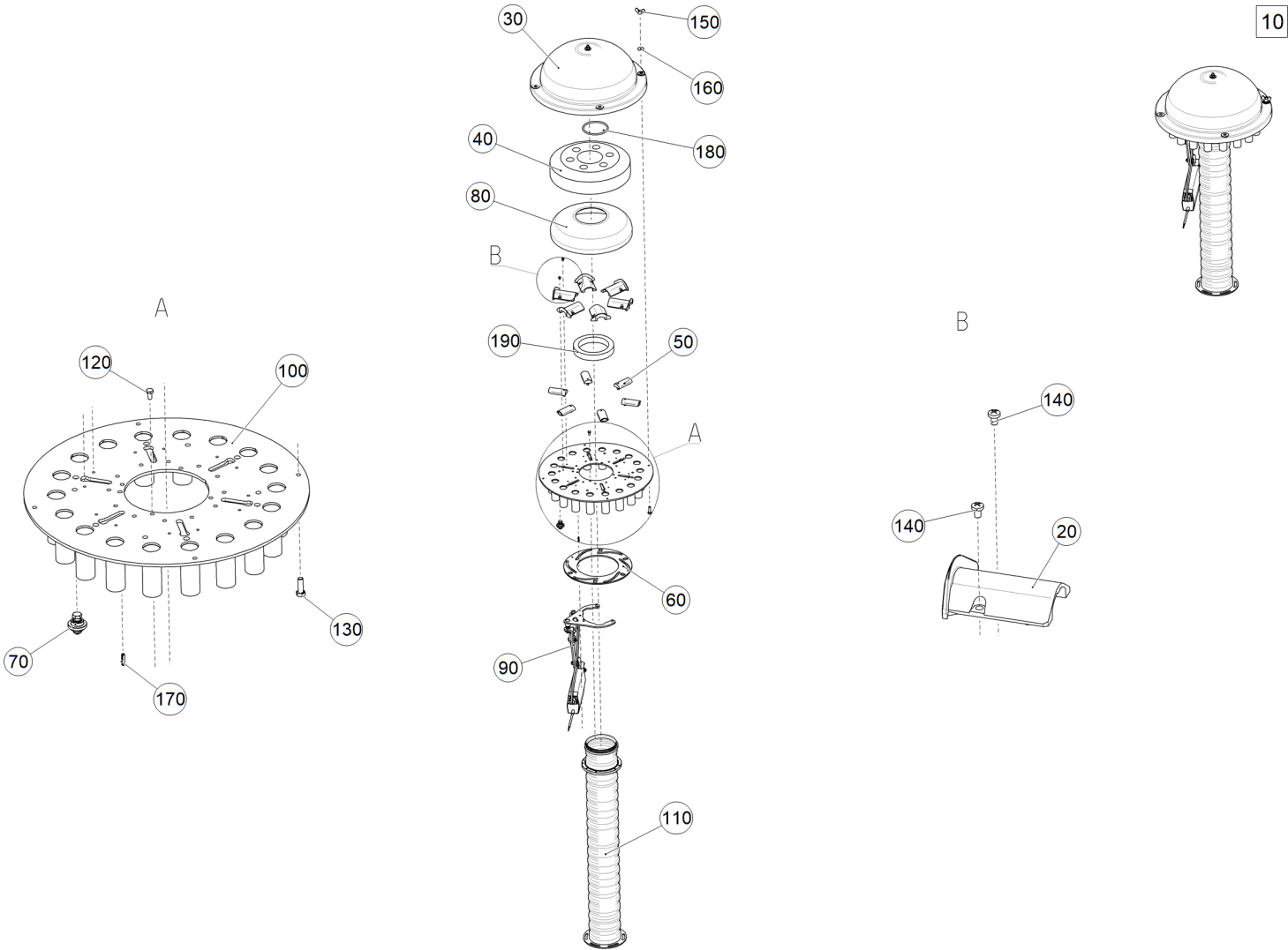
Рис. 1 ЕТВ-6000000101 (Гриб распределительный 18-125-6)
