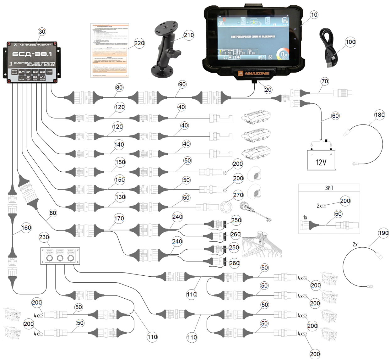
Рис. 1 ЕТВ-6000000173 (63250578- Базовый комплект электроники СКИФ-38)
