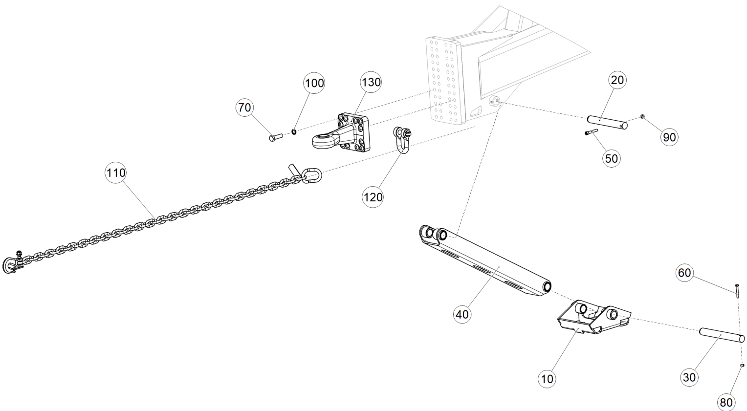
Рис. 1 ЕТВ-6000000014 Передняя часть
