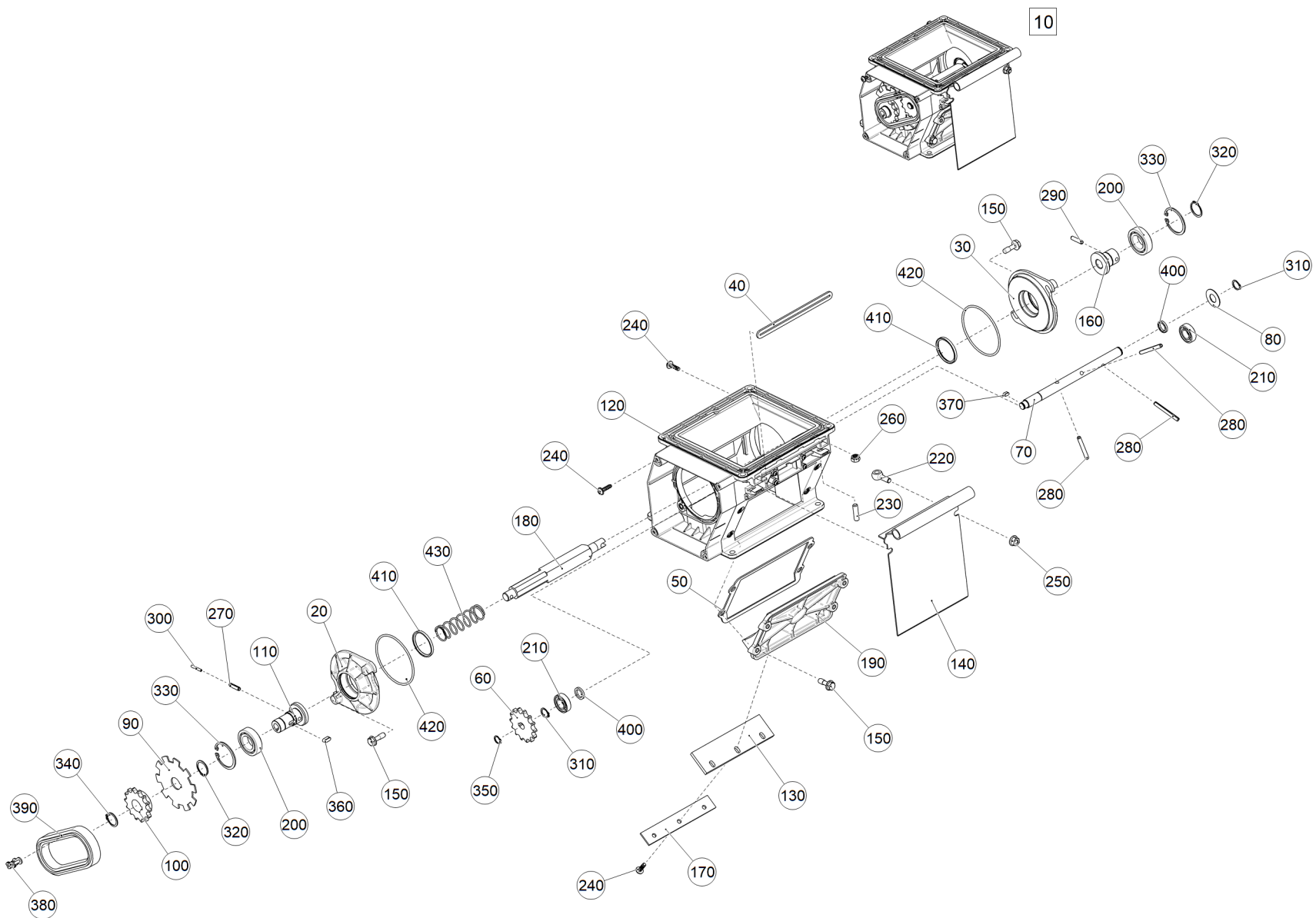
Рис. 1 ЕТВ-6000000046 (Дозатор 3.1 D12 левый)
