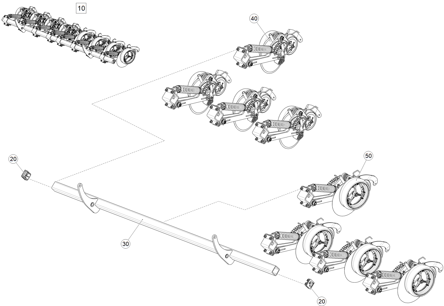
Рис. 1 ЕТВ-6000000099 (Балка сошниковая передняя центральная)
