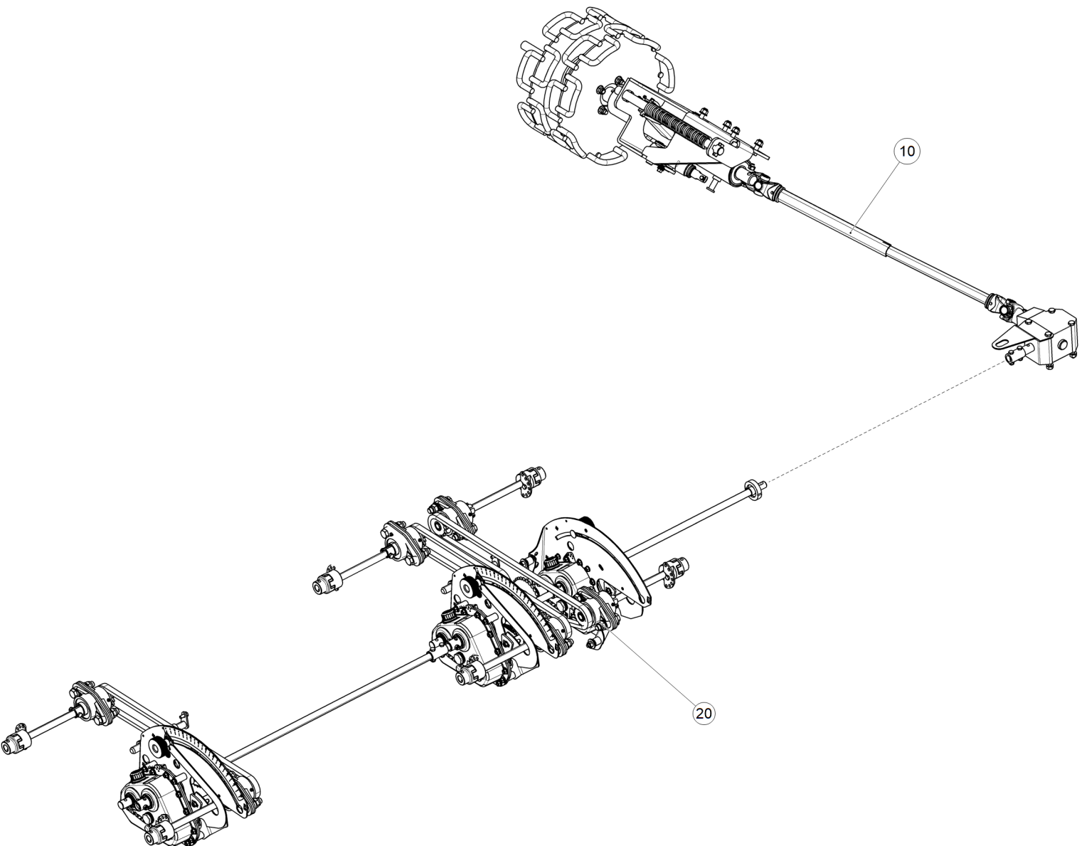
Рис. 1 ETV-6000000032 (Привод)
