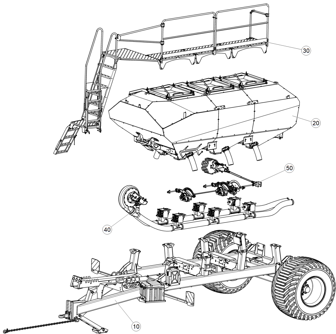
Рис. 1 HBG-01 (Бункер/Рама)
