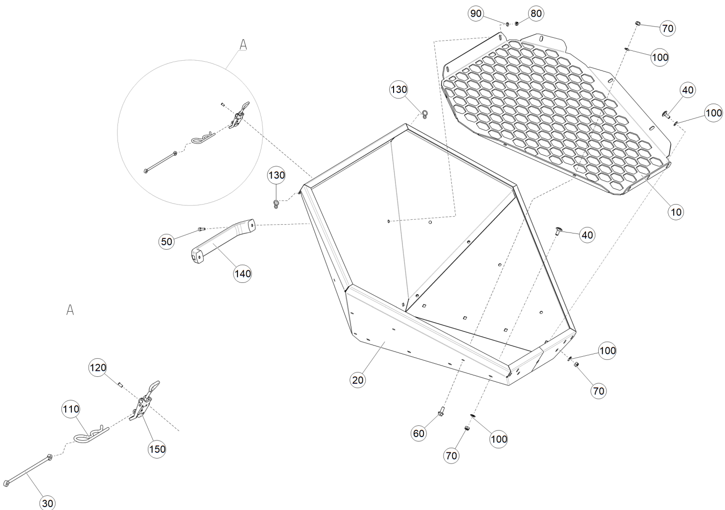
Рис. 1 ЕТВ-6000000187 (Ковш)
