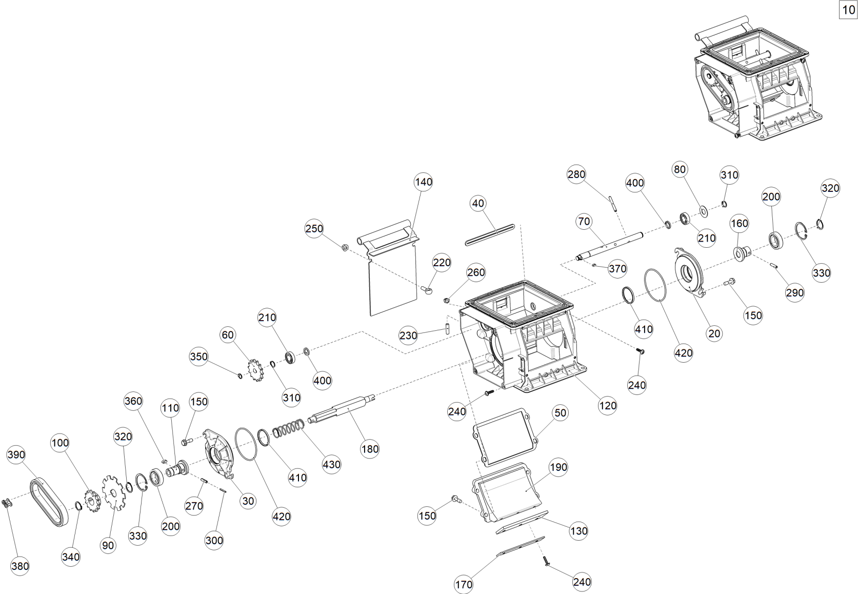
Рис. 1 ЕТВ-6000000050 (Дозатор 3.1 D12 правый)
