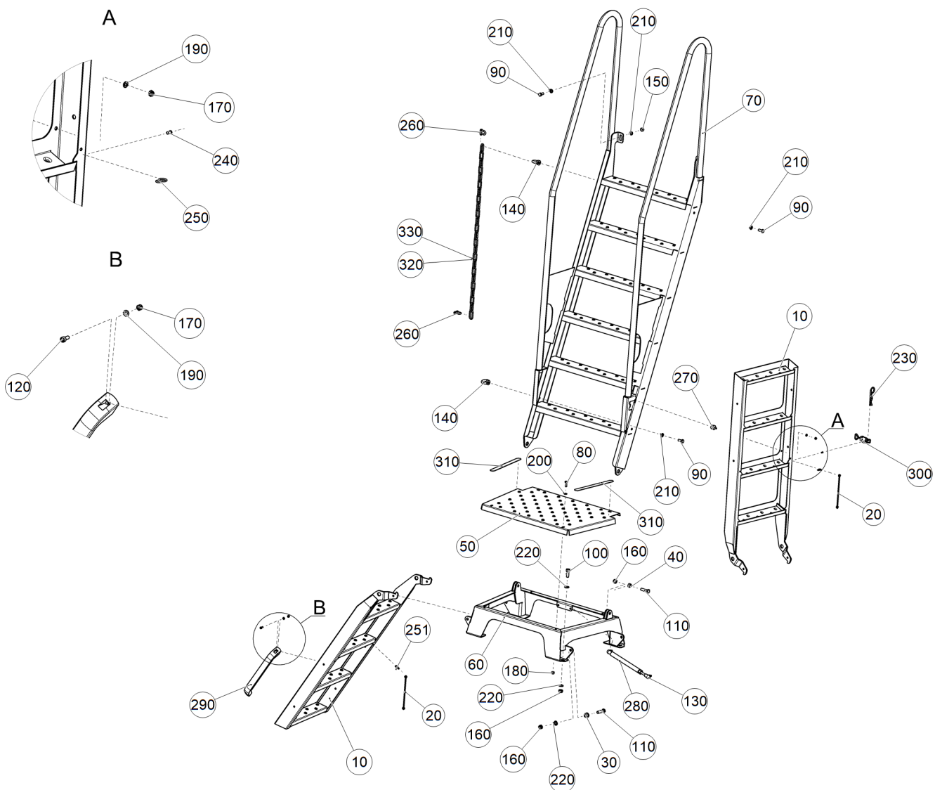
Рис. 1 ЕТВ-6000000027 (Лестница)
