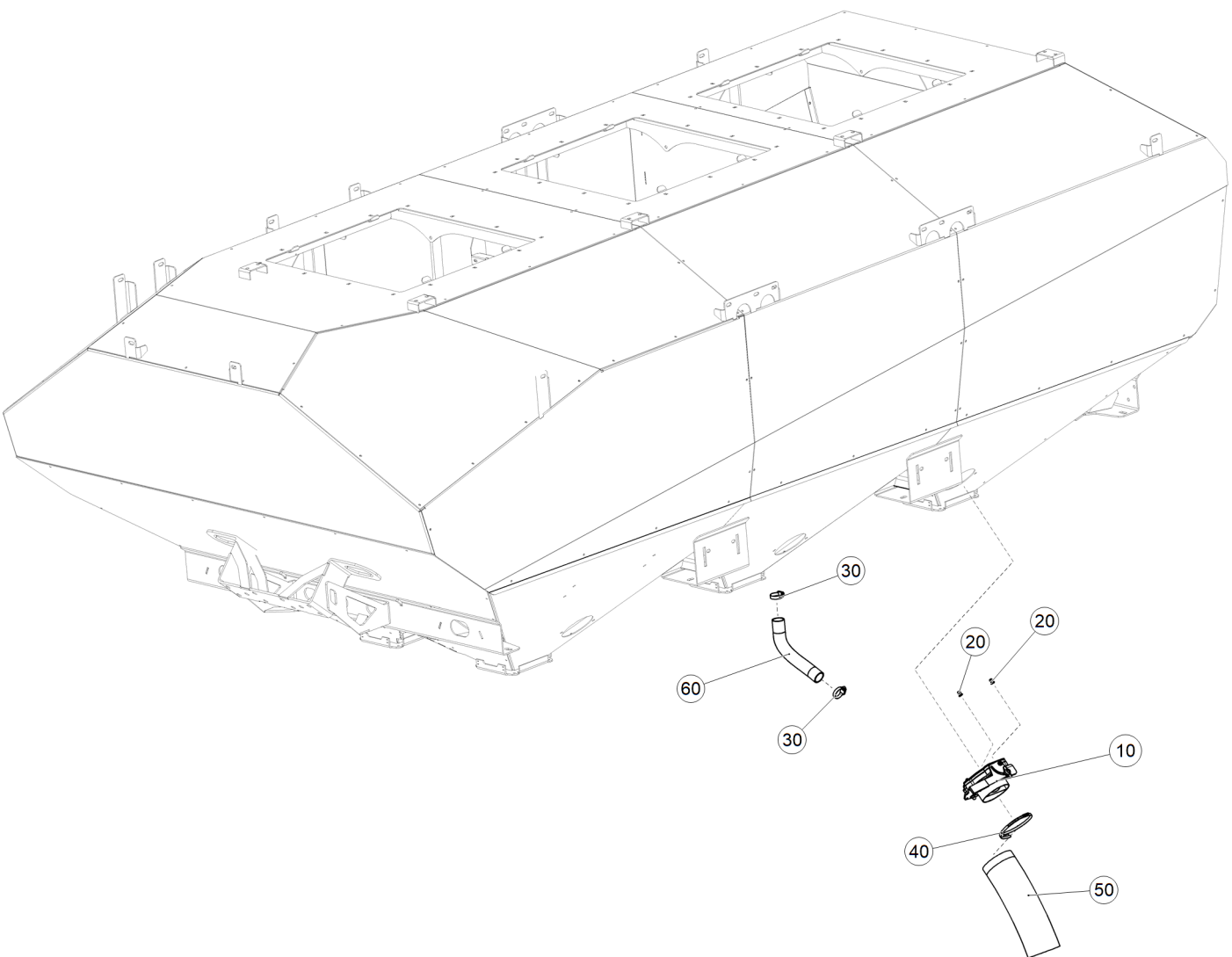
Рис. 1 ЕТВ-6000000024 (Устройство быстрого опорожнения)
