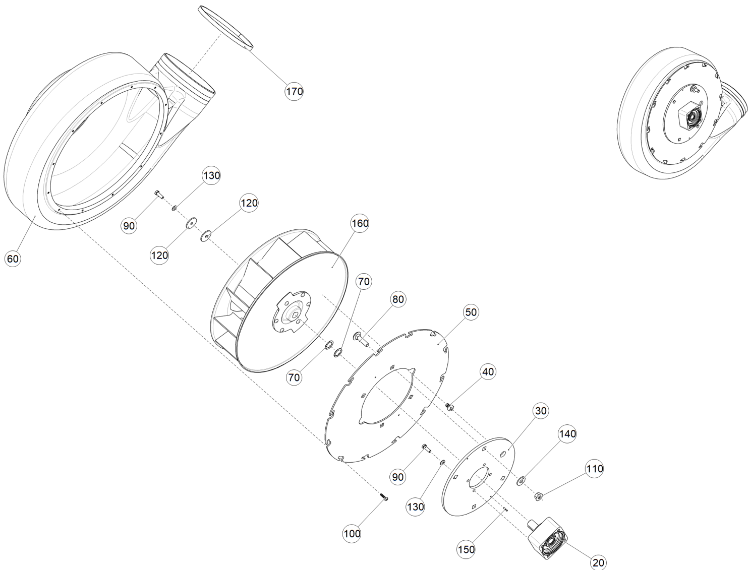
Рис. 1 ЕТВ-6000000044 (Кожух вентилятора)
