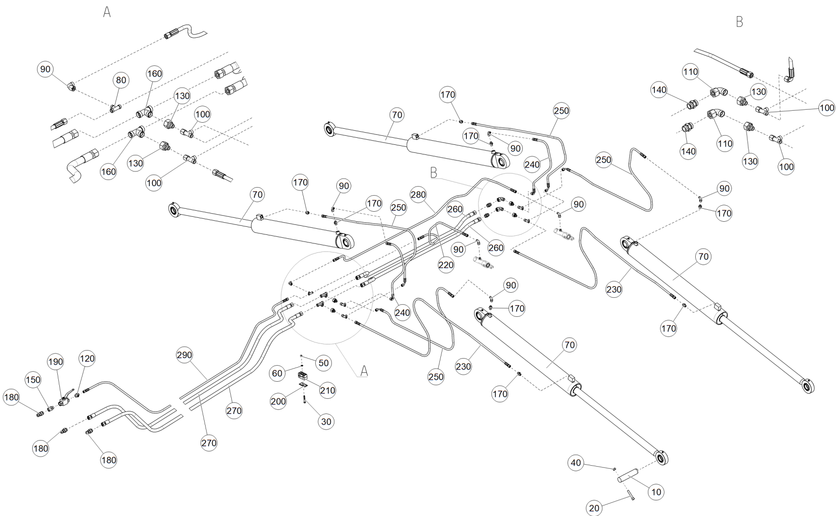
Рис. 1 ЕТВ-6000000224 (Гидрооборудование складывания секций)
