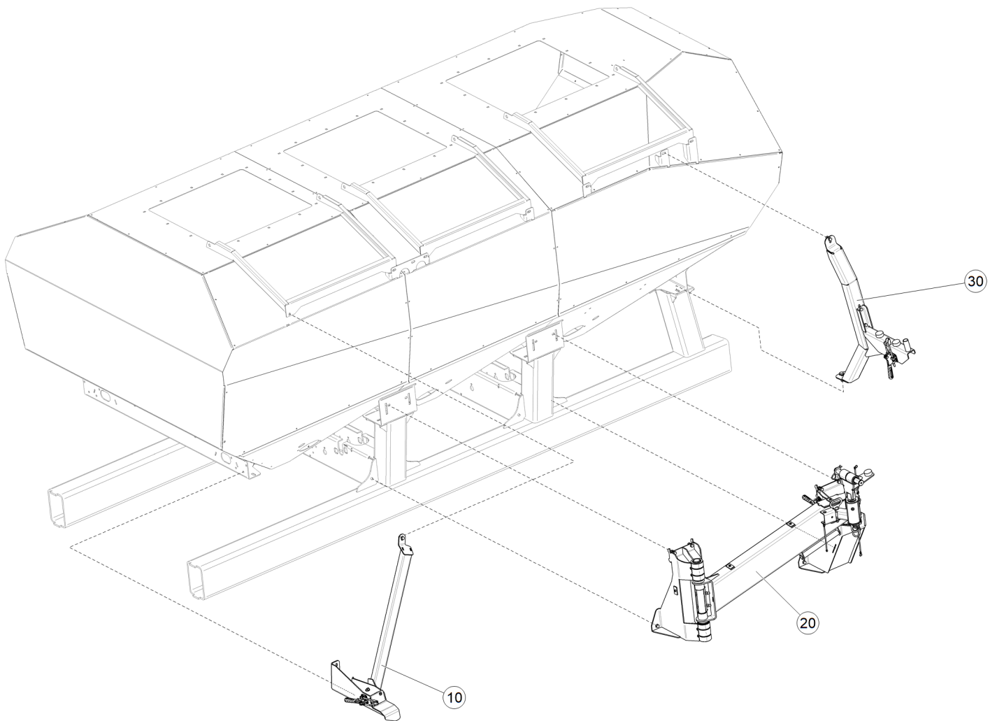
Рис. 1 ЕТВ-6000000196 (Опоры и кронштейны)
