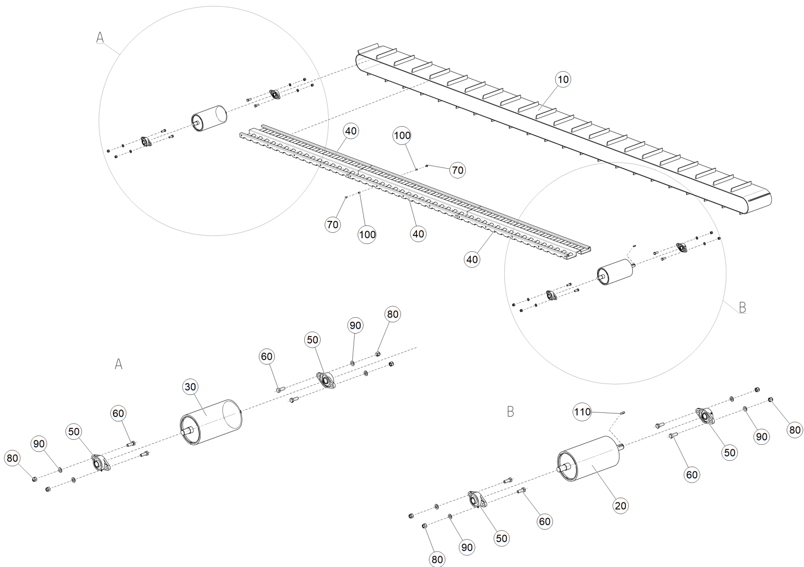
Рис. 1 ЕТВ-6000000192 (Лента конвейерная)
