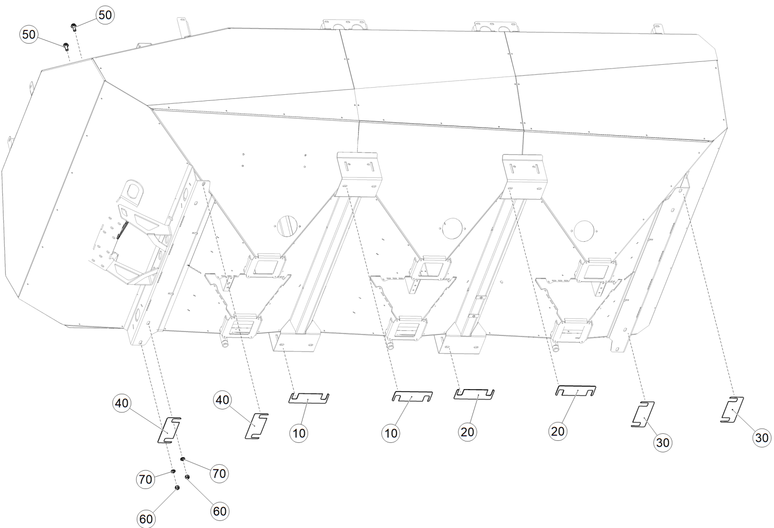
Рис. 1 ЕТВ-6000000023 (Подкладки с крепежом)
