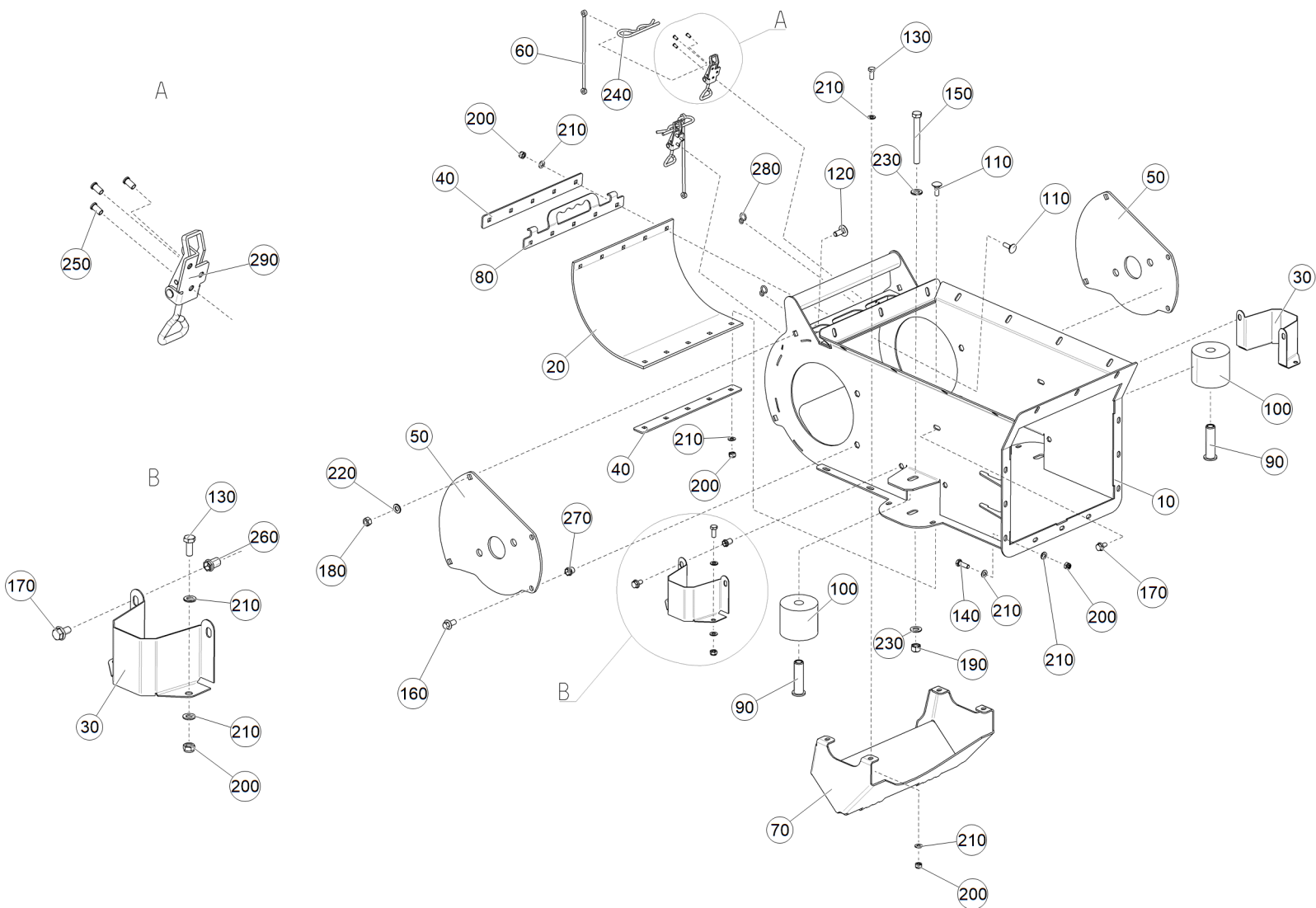
Рис. 1 ЕТВ-6000000186 (Башмак)
