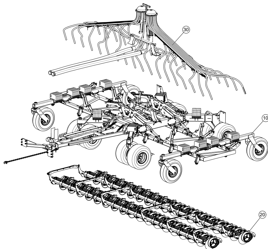
Рис. 1 HBG-02 (Рама сеялки)
