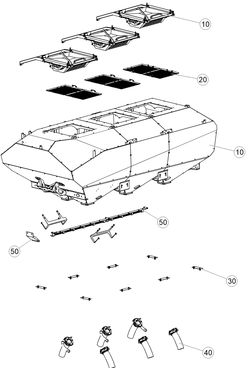
Рис. 1 ЕТВ-6000000020 (Бункер)
