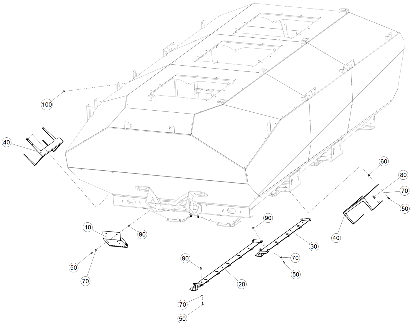
Рис. 1 ЕТВ-6000000025 (Кронштейны и лотки)
