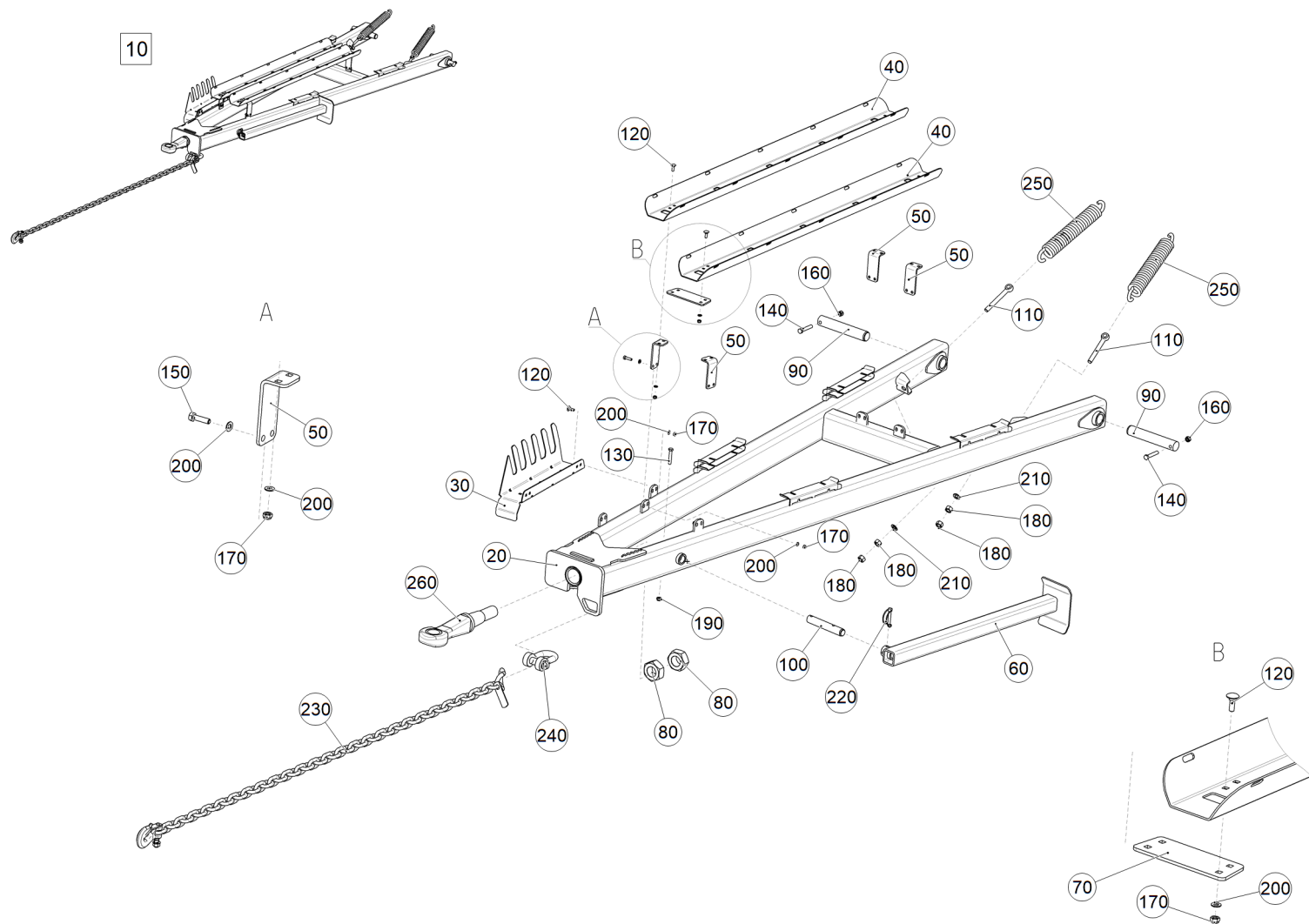
Рис. 1 ЕТВ-60000000088 (Дышло DSC в сборе)
