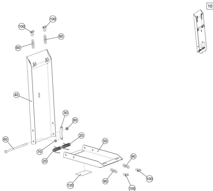
Рис. 1 ЕТВ-6000000125 (Башмак складной)
