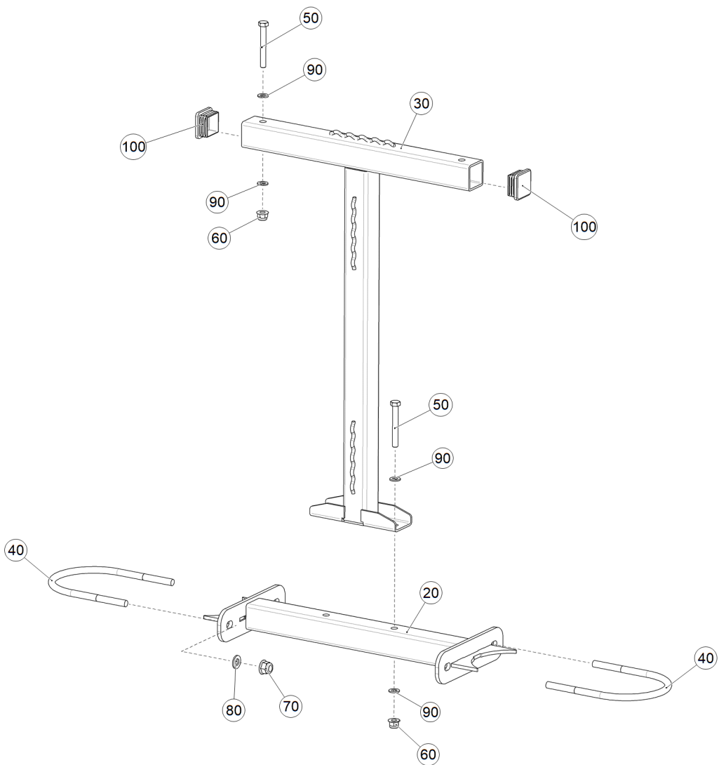
Рис. 1 ETB-6000000107 (Кронштейн освещения)
