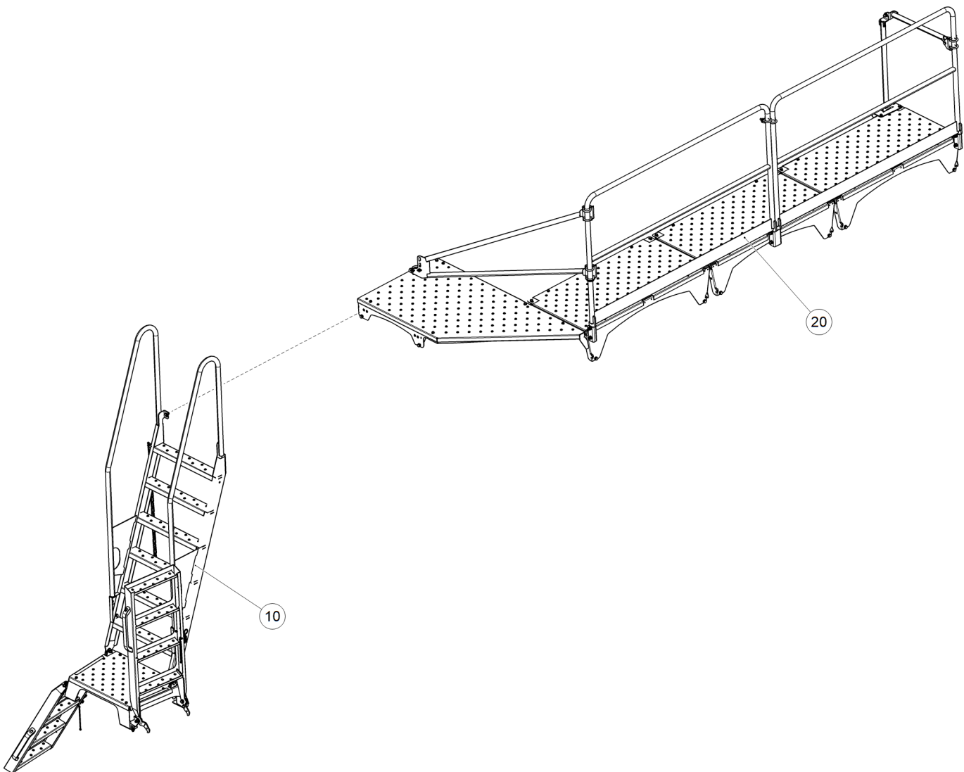
Рис. 1 ЕТВ-6000000026 (Площадка и лестницы)
