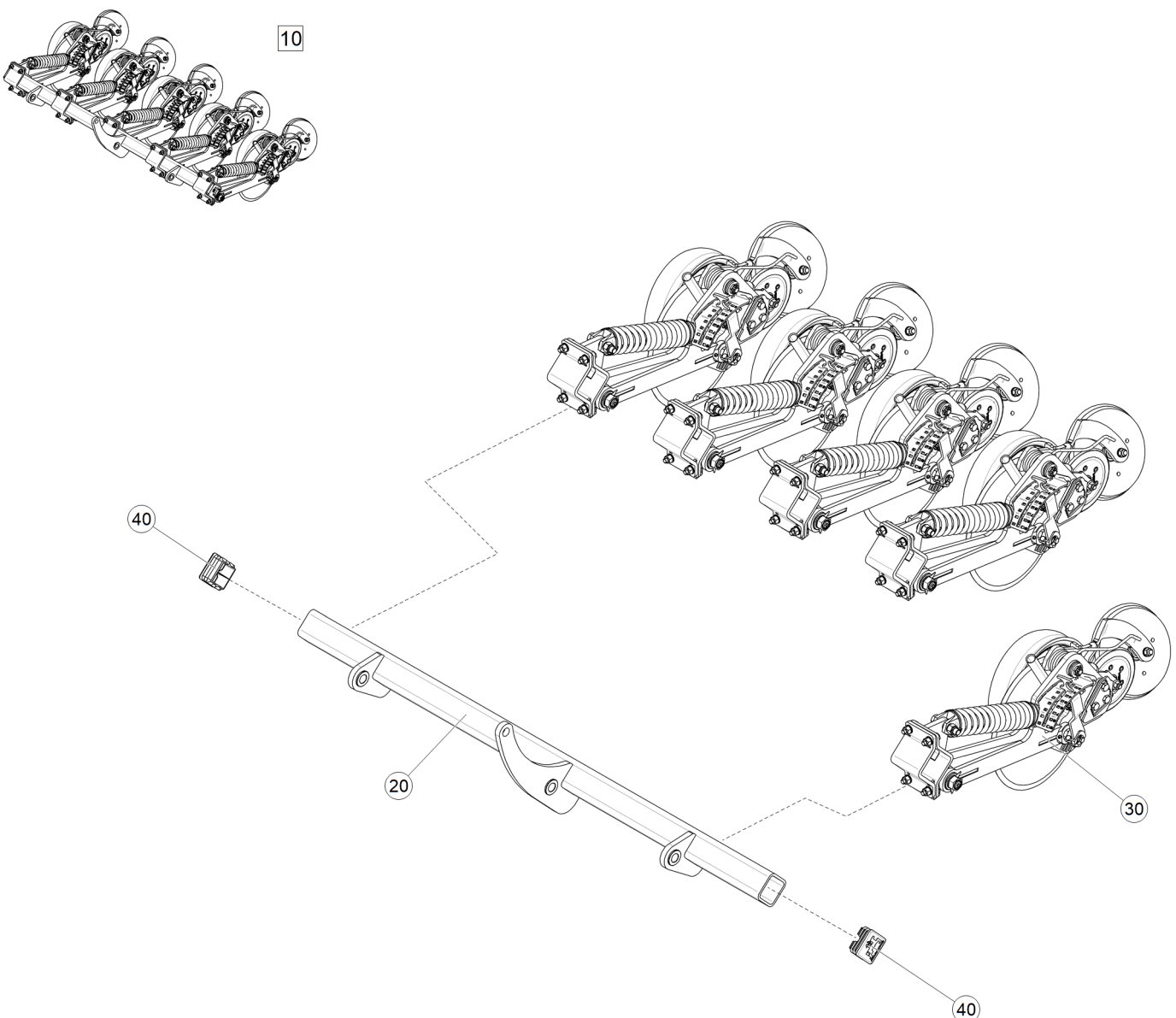
Рис. 1 ЕТВ-6000000156 (Балка сошниковая правая средняя задняя)
