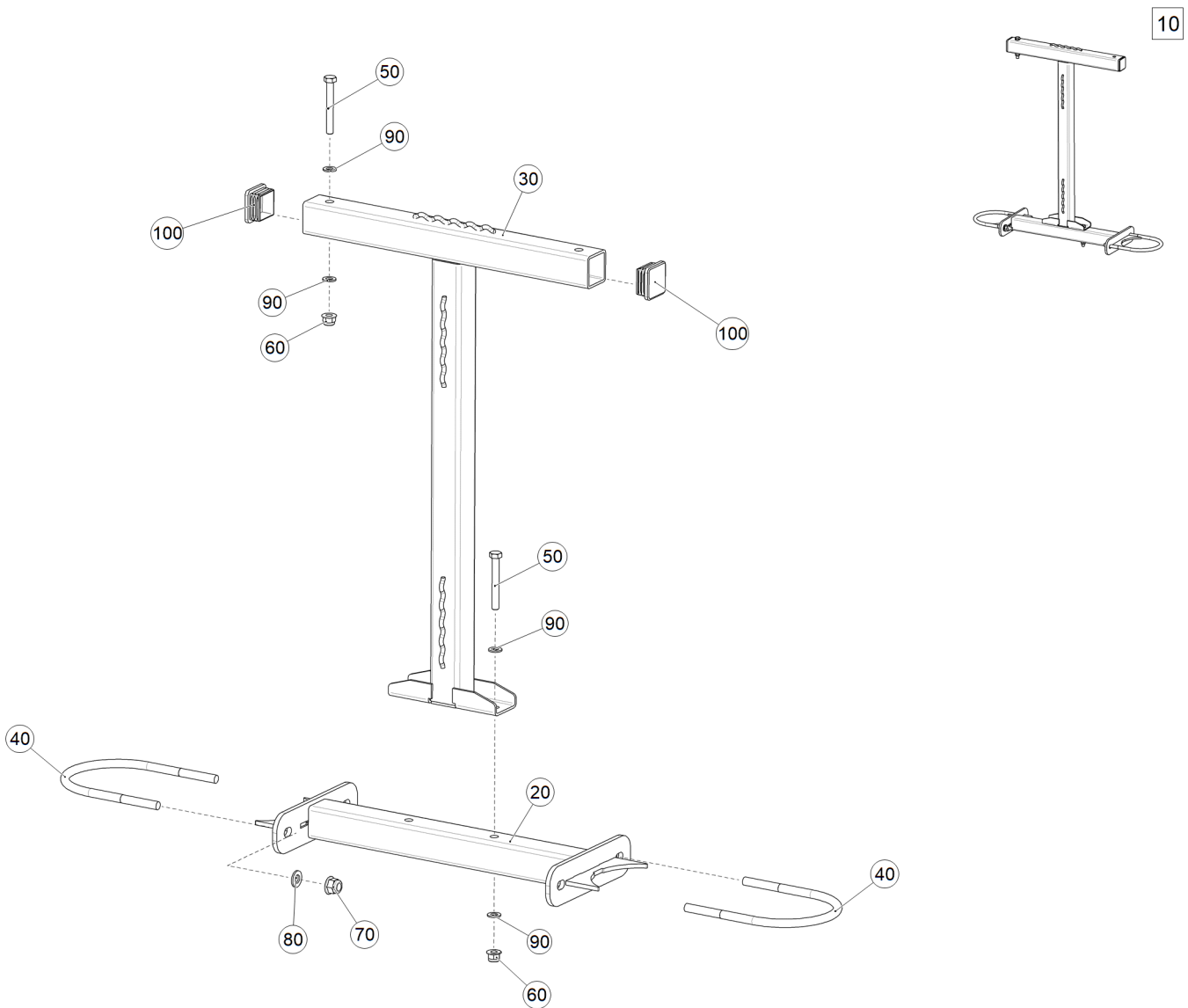
Рис. 1 ЕТВ-6000000107 (Кронштейн освещения)
