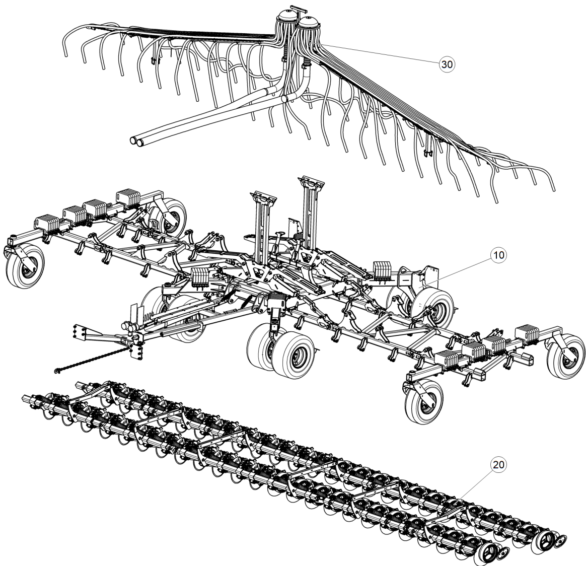
Рис. 1 HBG-02 (Рама сеялки)
