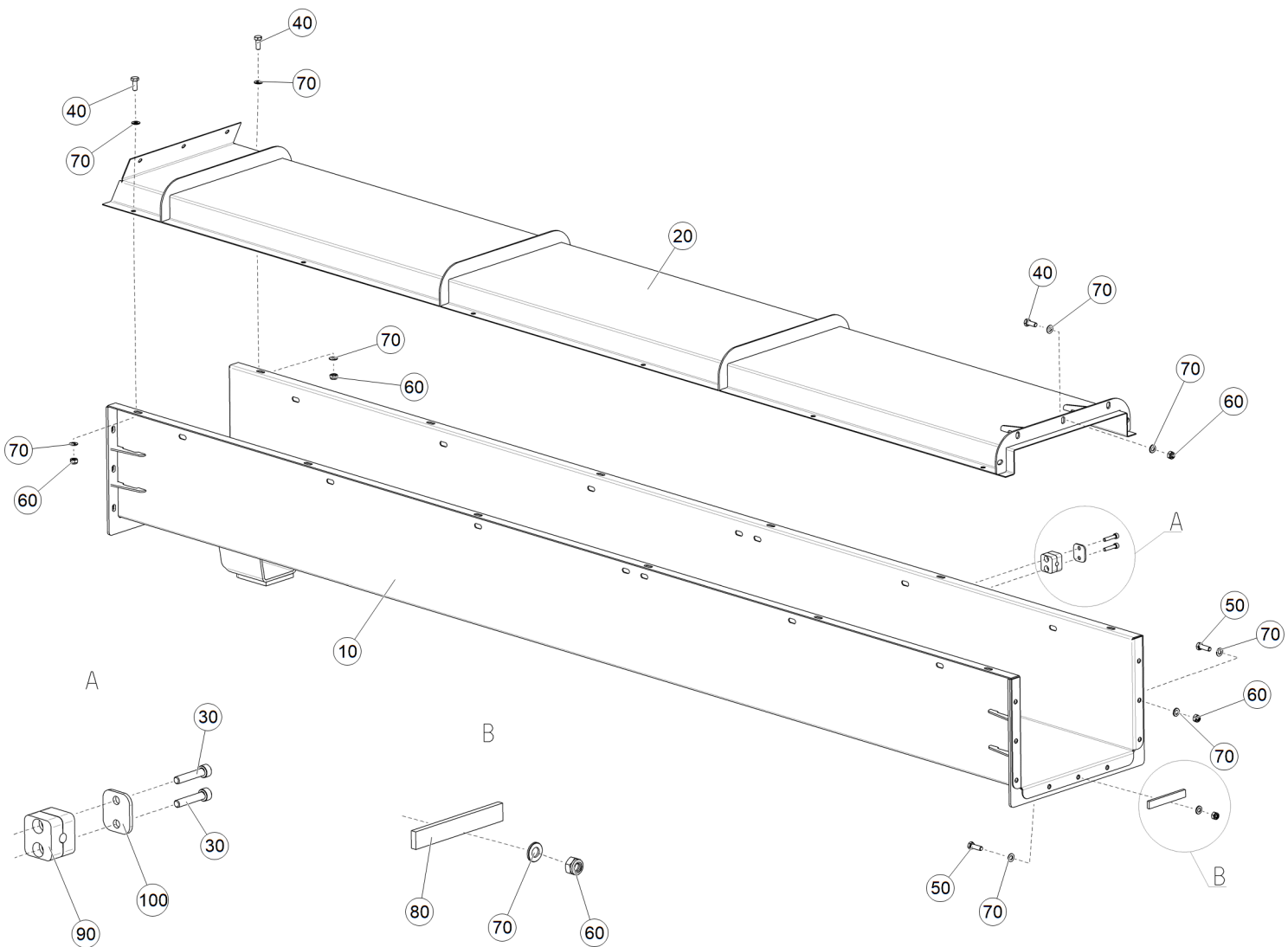
Рис. 1 ETV-6000000190 (Секция нижняя)
