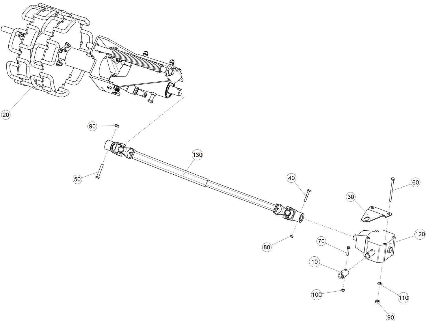
Рис. 1 ЕТВ-6000000033 (Привод колеса, кардан, редуктор)
