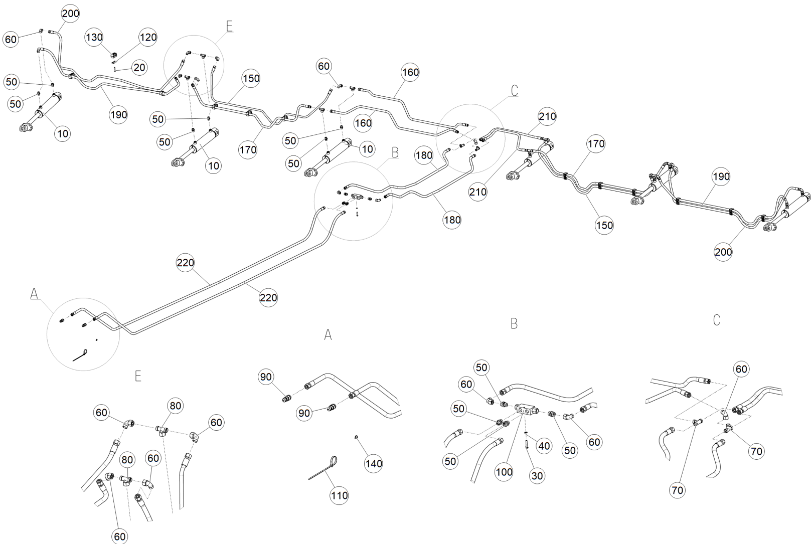
Рис. 1 ЕТВ-6000000235 (Гидрооборудование подъема/опускания сошников)
