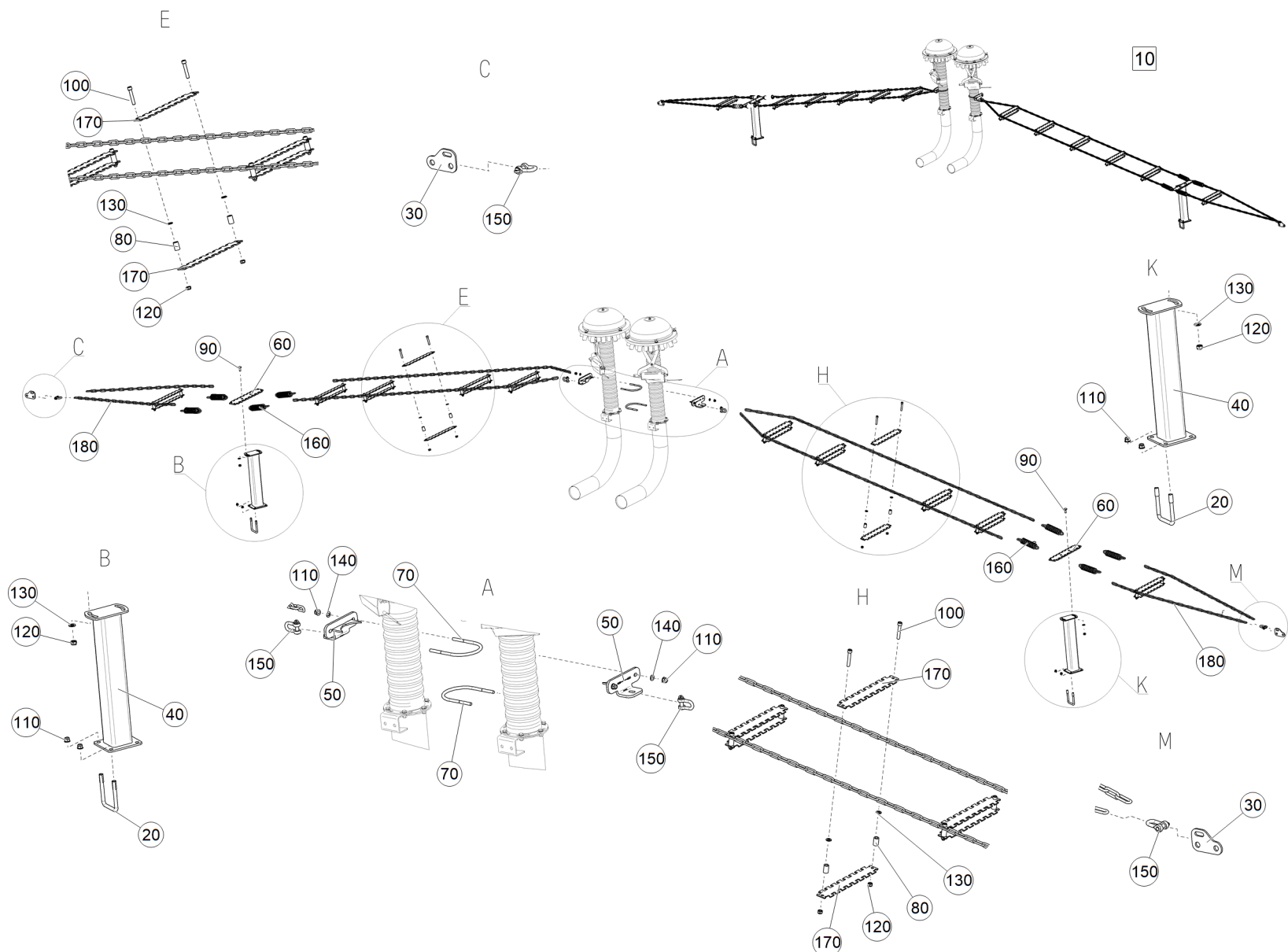
Рис. 1 ЕТВ-6000000165 (Комплект цепей семяпродов DSC12)
