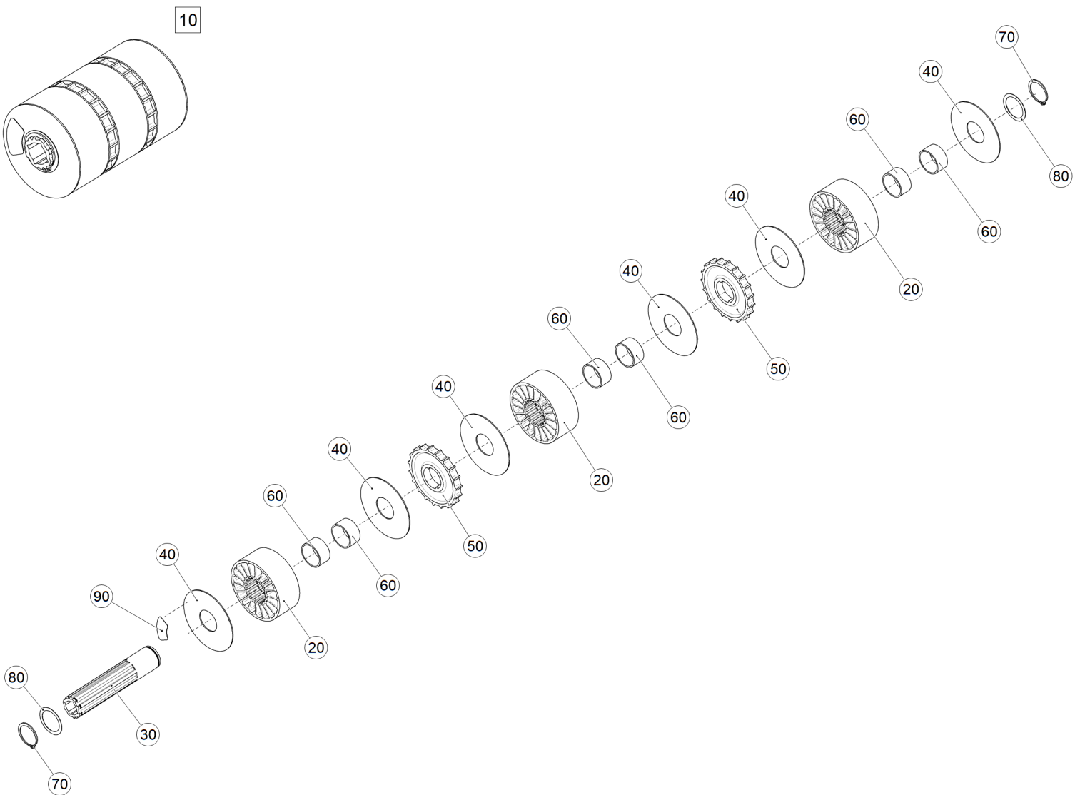
Рис. 1 ETB-6000000109 (Катушка высевающая 20 см)
