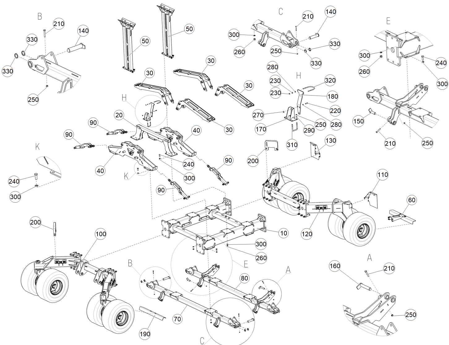
Рис. 1 ETV-6000000137 (Рама центральная)
