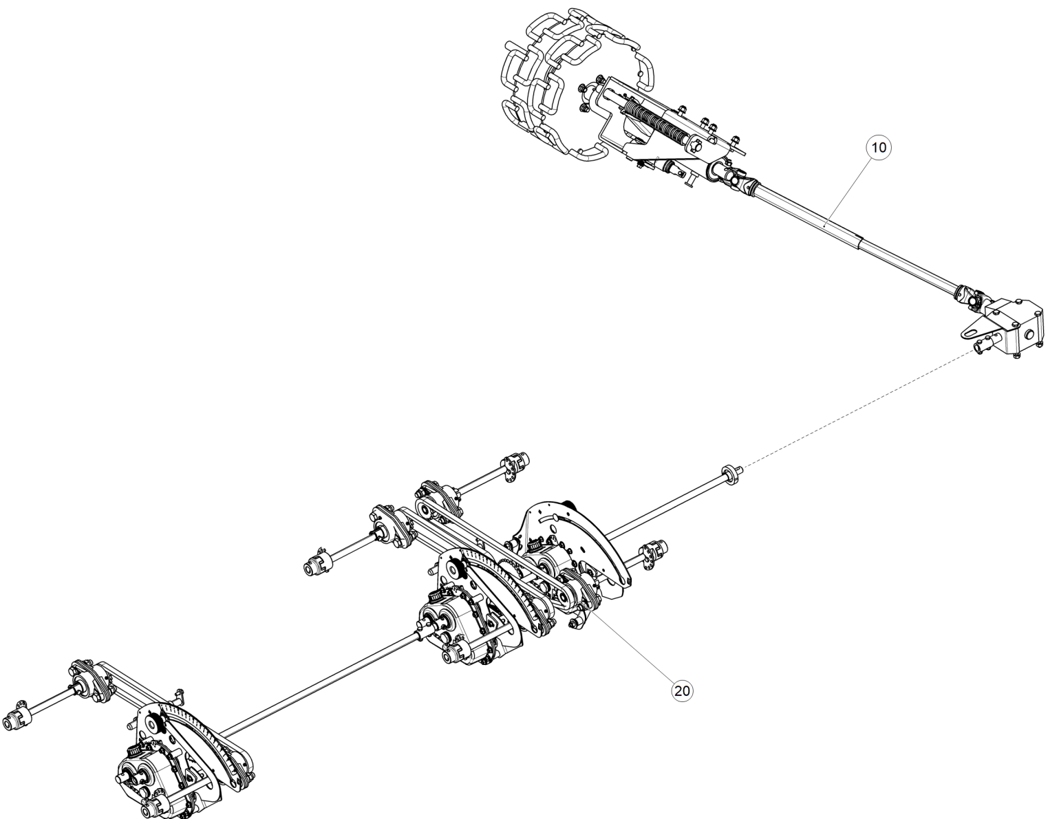
Рис. 1 ETV-6000000032 (Привод)
