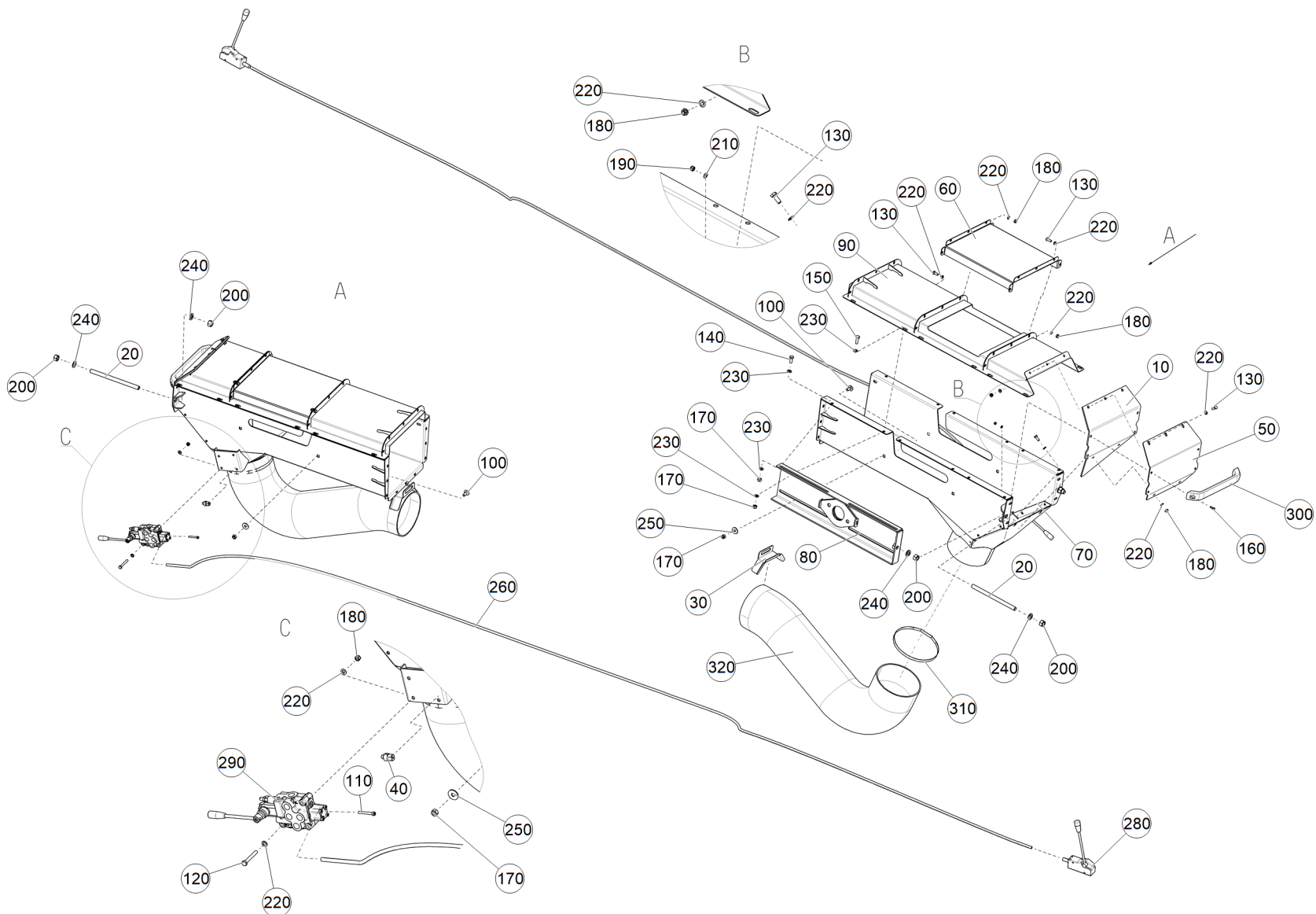
Рис. 1 ETB-6000000194 (Оголовок)
