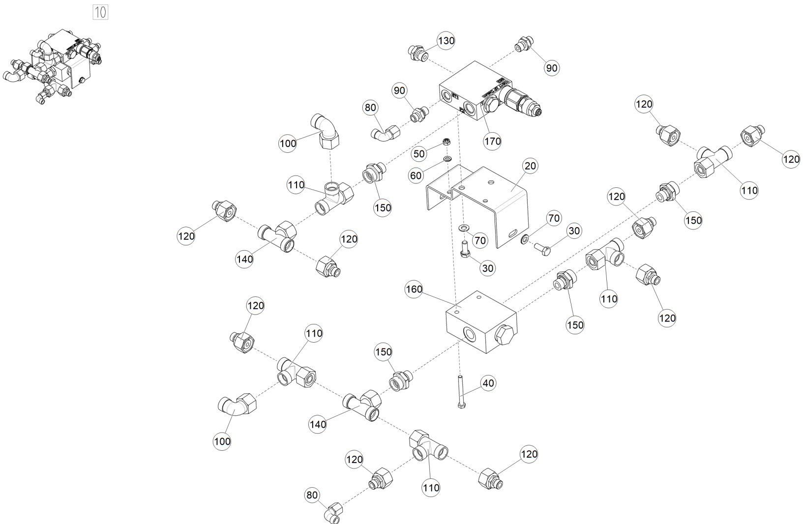
Рис. 1 ЕТВ-6000000238 (Сборка гидроблоков DSC12)
