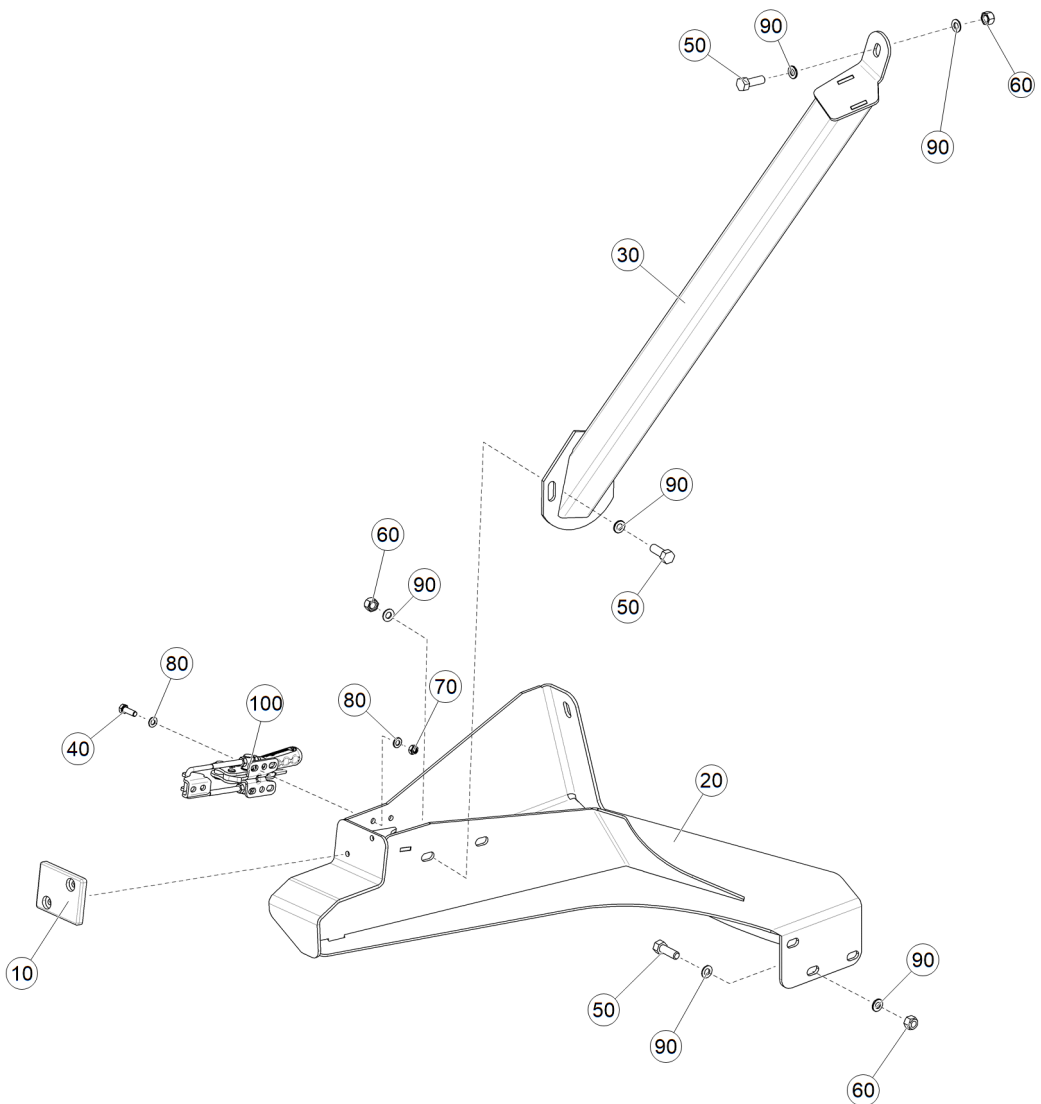
Рис. 1 ETB-6000000197 (Опоры и кронштейны нижние)
