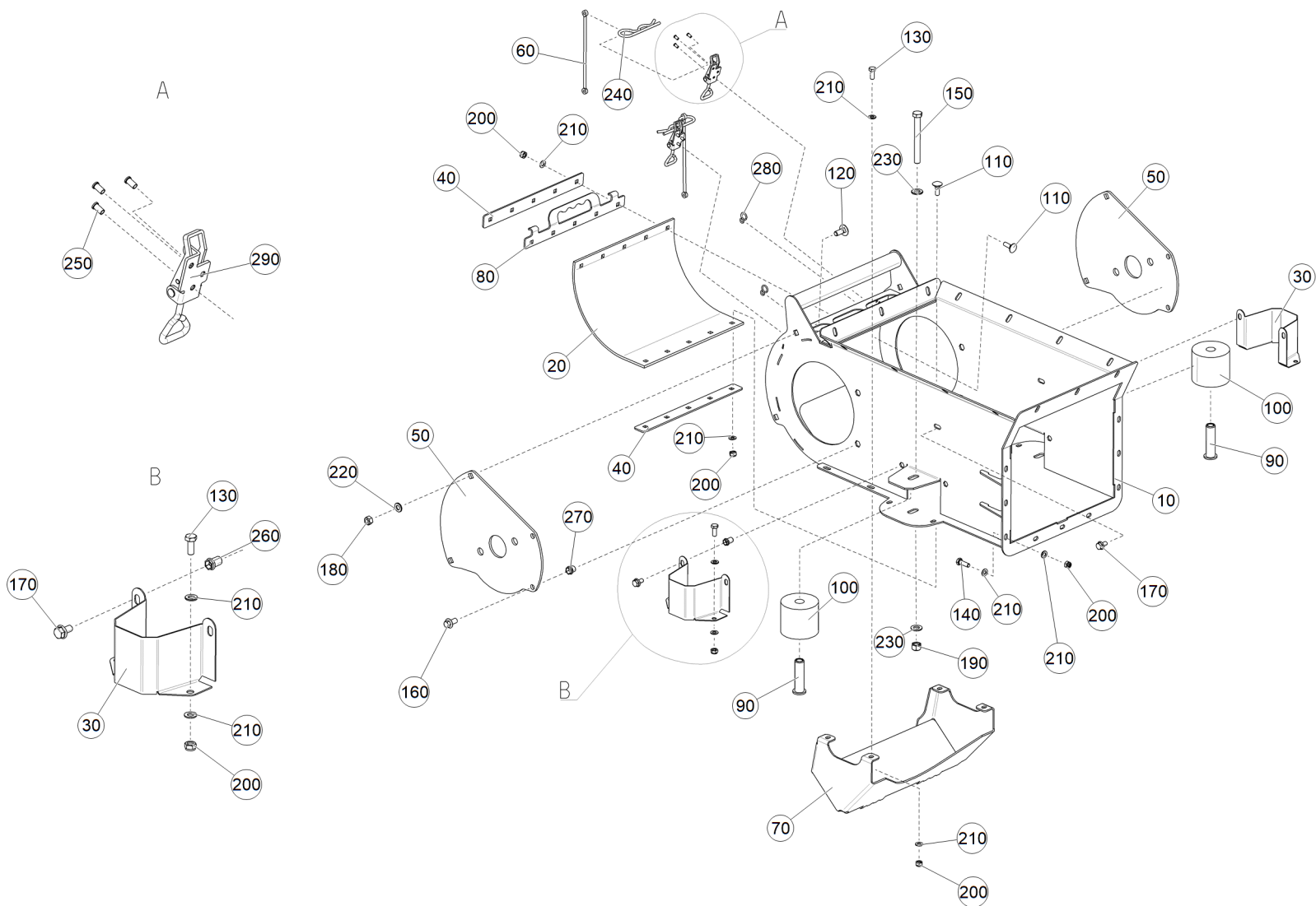
Рис. 1 ЕТВ-6000000186 (Башмак)
