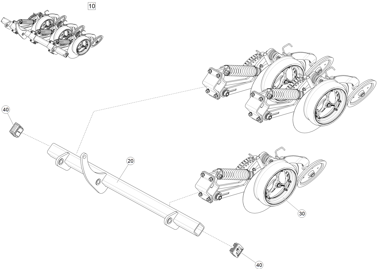
Рис. 1 ЕТВ-6000000147 (Балка сошниковая левая крайняя передняя)
