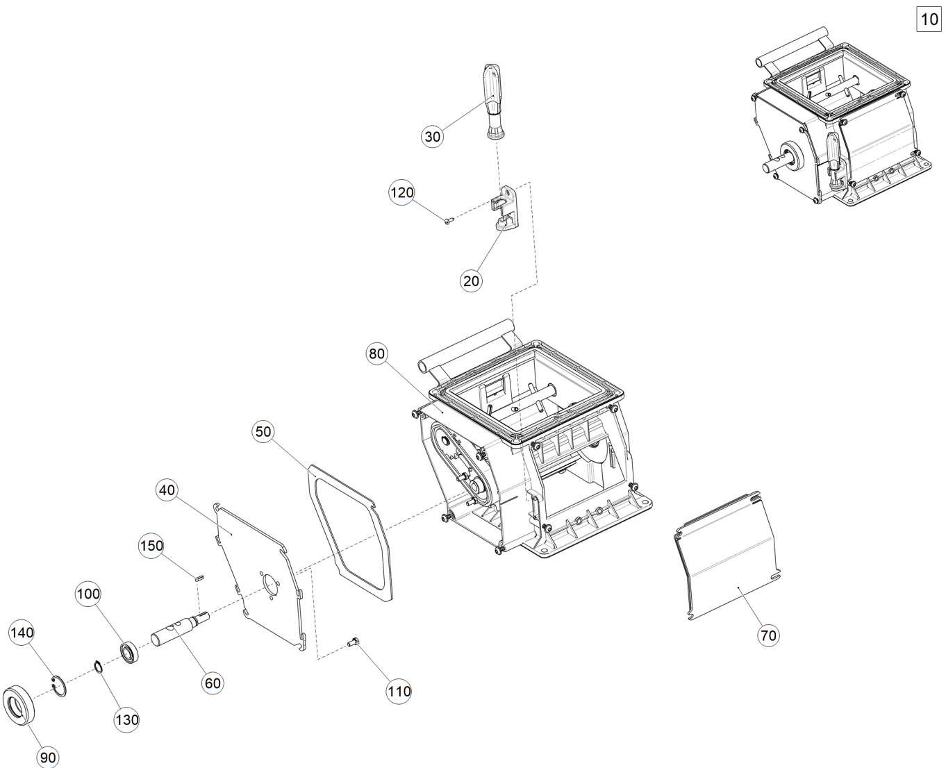
Рис. 1 ЕТВ-6000000049 (Дозатор DSC без патрубка правый)
