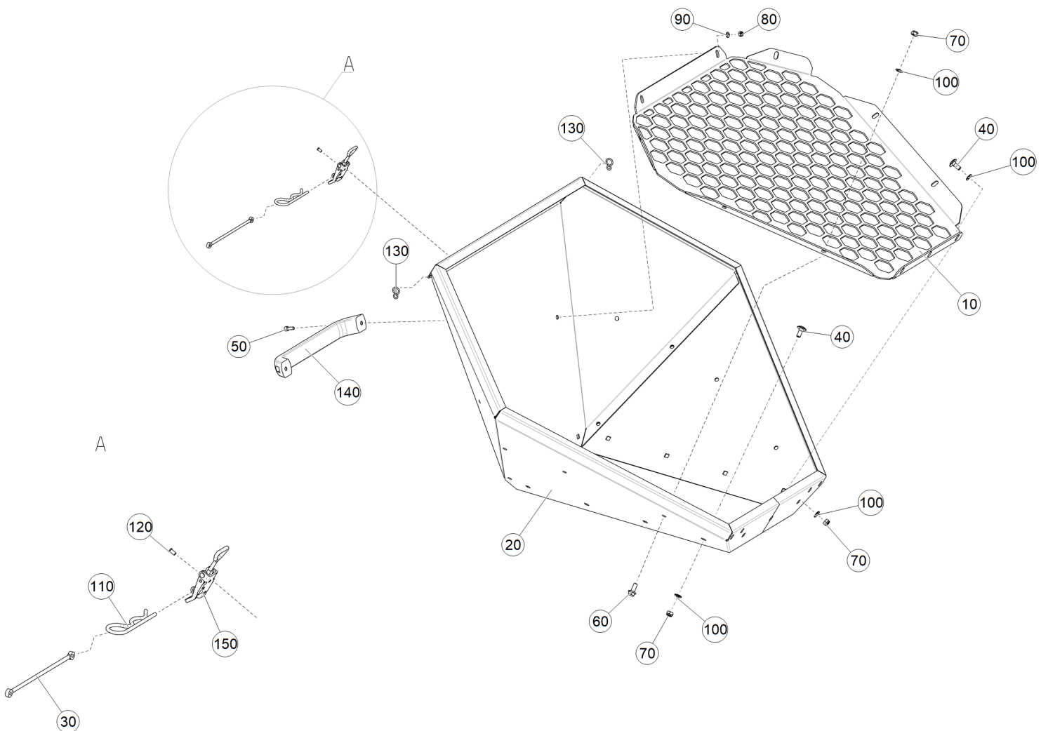
Рис. 1 ЕТВ-6000000187 (Ковш)
