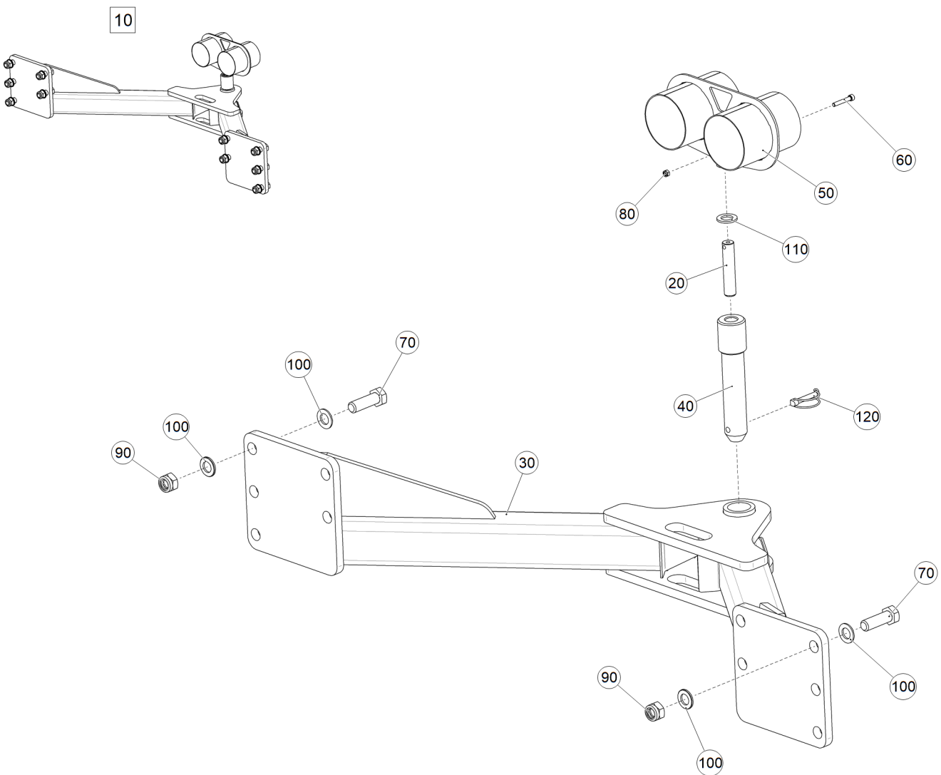
Рис. 1 ЕТВ-6000000087 (Сцепное устройство DSC)
