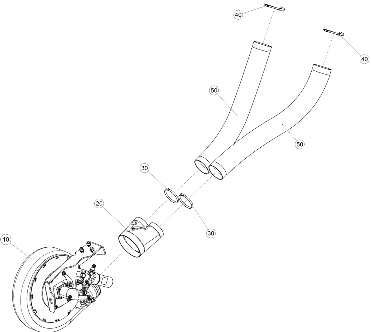
Рис. 1 ЕТВ-6000000030 (Вентилятор)
