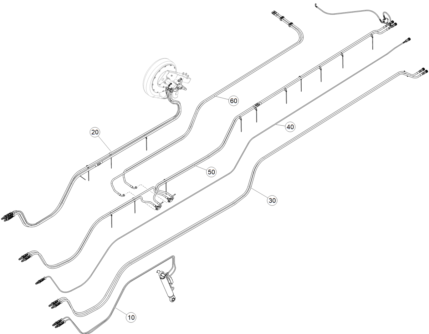
Рис. 1 ЕТВ-6000000115 (Гидрооборудование бункер/рама)
