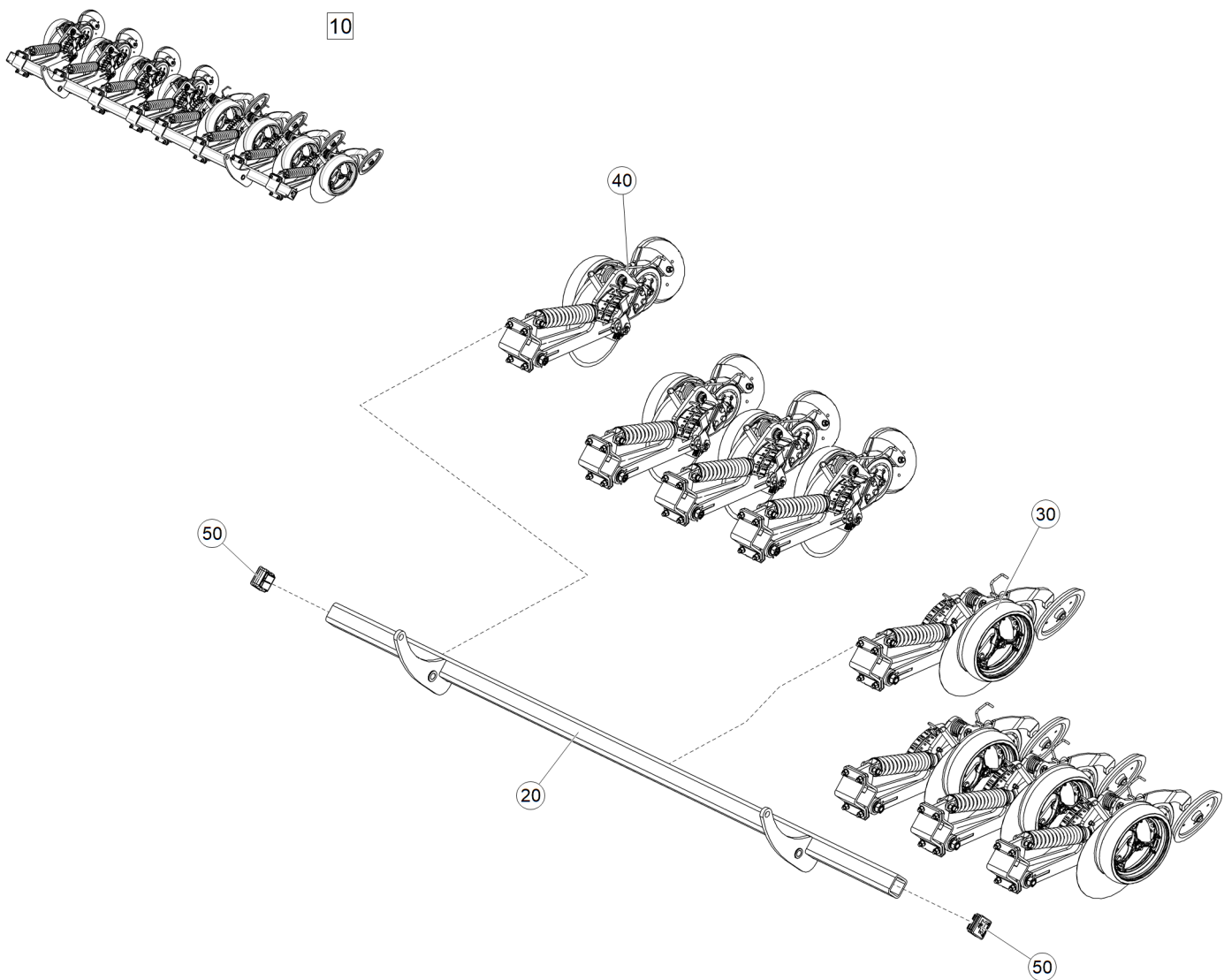
Рис. 1 ЕТВ-6000000151 (Балка сошниковая центральная передняя)
