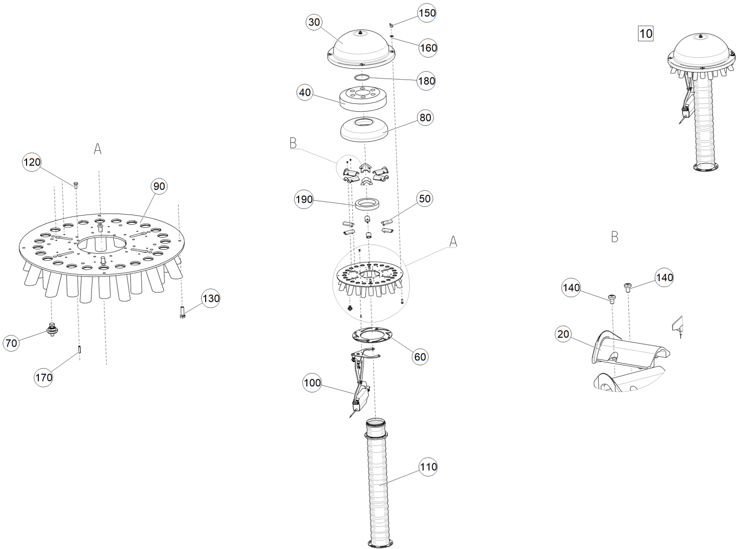
Рис. 1 ЕТВ-6000000163 (Гриб распределительный 24-125-6)
