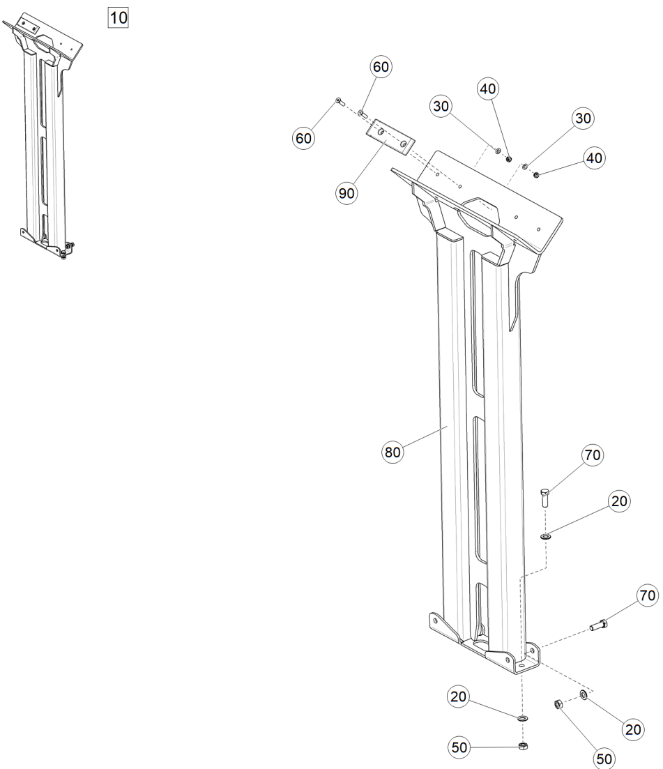
Рис. 1 ЕТВ-6000000157 (Стойка)
