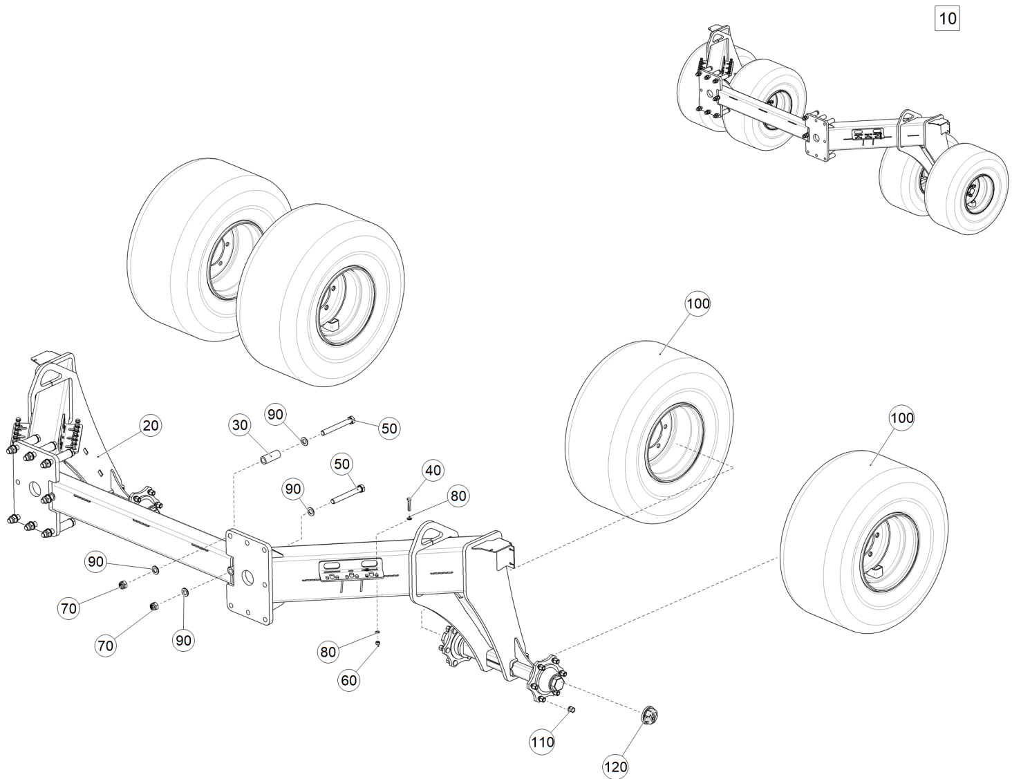
Рис. 1 ЕТВ-6000000085 (Рама колесная задняя в сборе)
