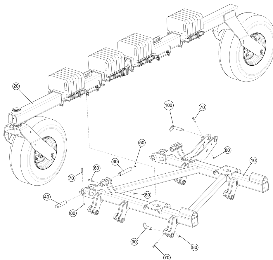
Рис. 1 ETB-6000000135 (Рама левая крайняя)
