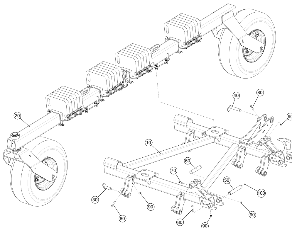
Рис. 1 ETB-6000000138 (Рама правая крайняя)
