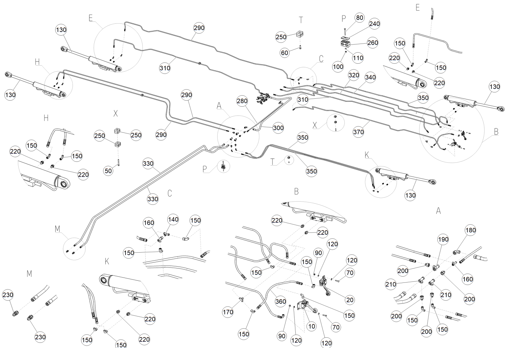
Рис. 1 ЕТВ-6000000237 (Гидрооборудование складывания крайних секций)
