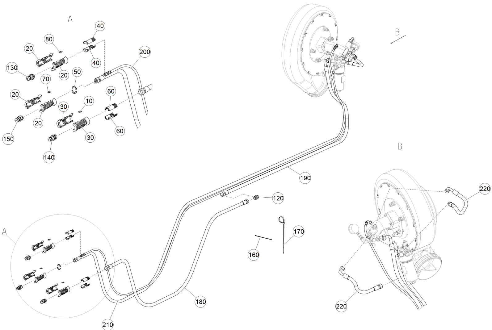
Рис. 1 ЕТВ-6000000120 (Линия вентилятора DSC)
