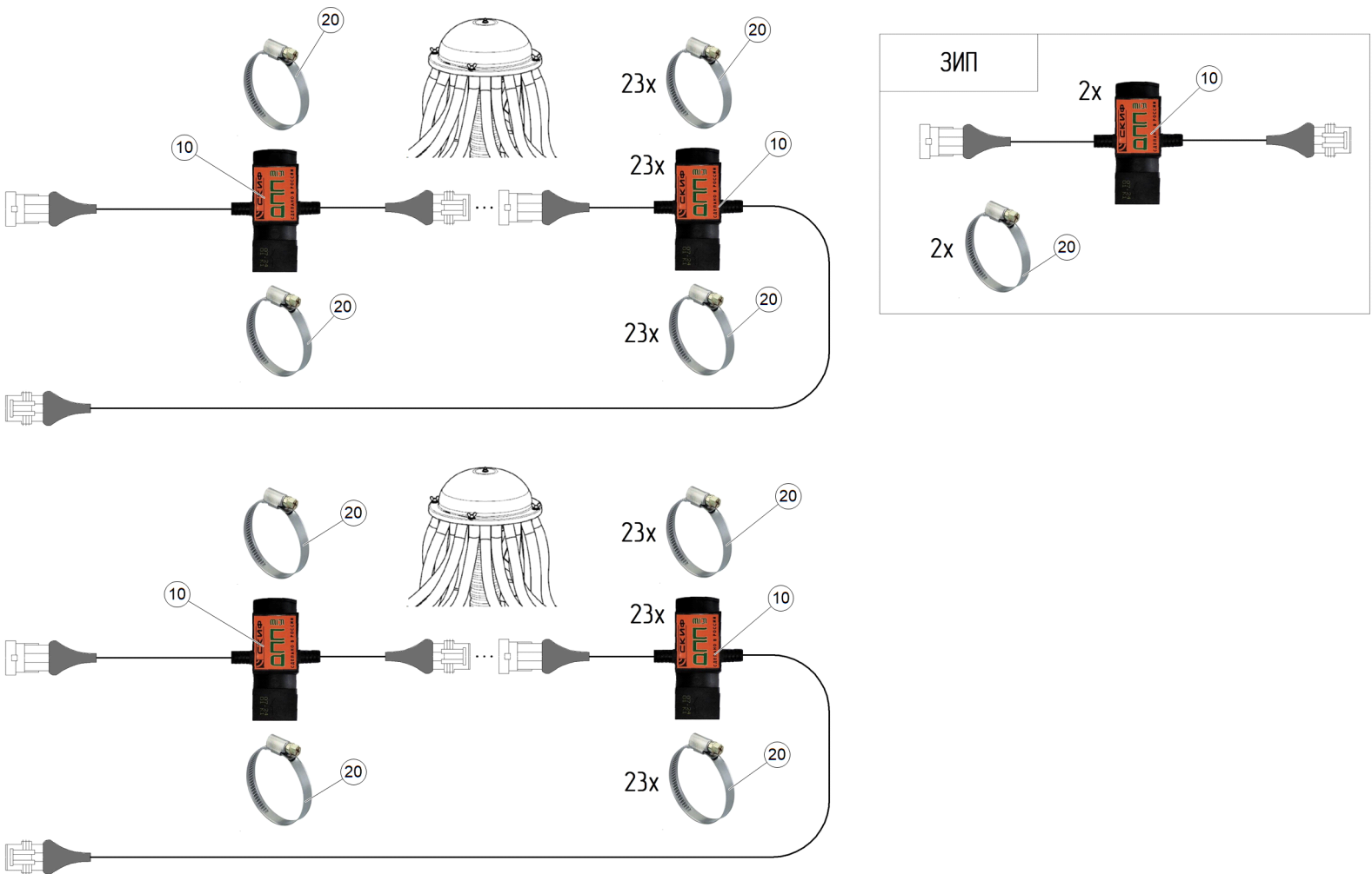
Рис. 1 ЕТВ-6000000234 (63251236 - Система контроля высева семян для DISCARA 12000 м/р 25 с СКИФ-38 в базе (опция))
