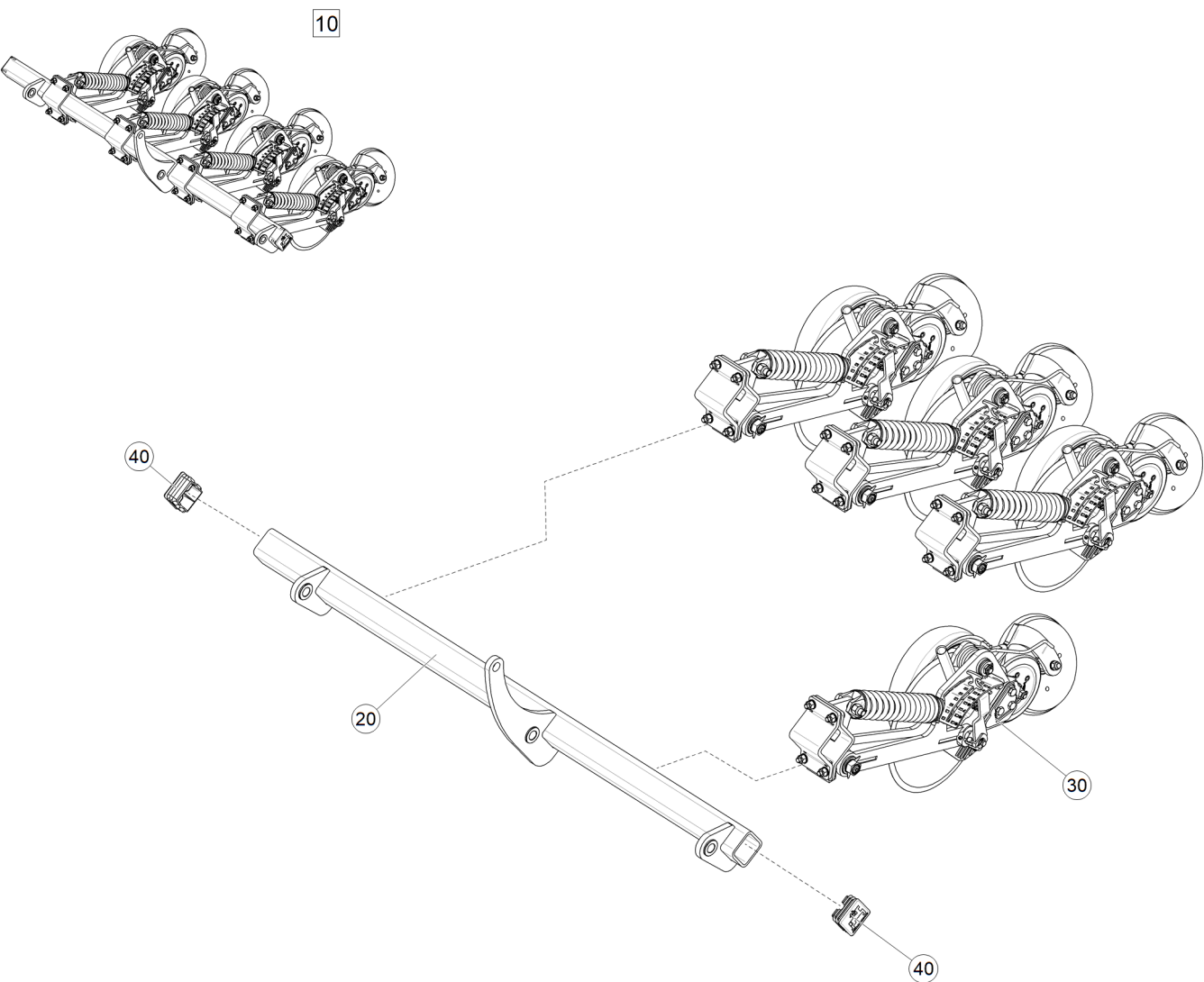
Рис. 1 ЕТВ-6000000155 (Балка сошниковая правая средняя передняя)
